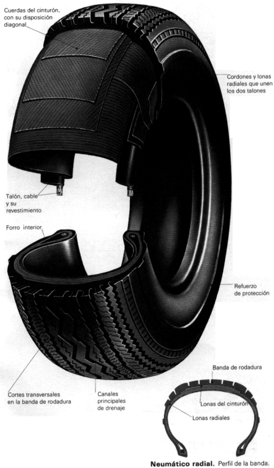
Figura 21. ("El Automóvil" Selecciones de Reader s Digest.)
