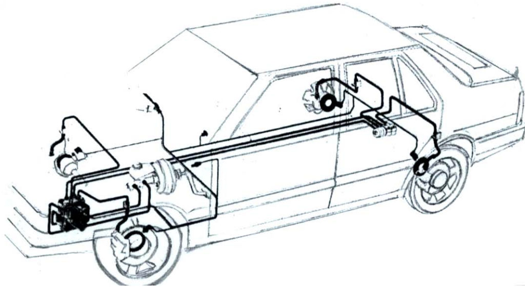
Figura 9.( Del libro “Tecnologías avanzadas del automóvil”.)
