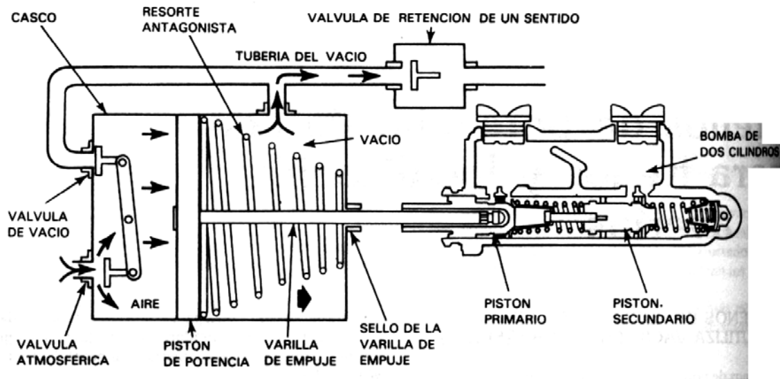
Figura 13.-Vista esquemática de un reforzador de un frenos de potencia de vacío. (Del libro "Equipo Diesel" tomo I, Erich J. Schulz, Edit. CECOSA, primera edición 1985.)
