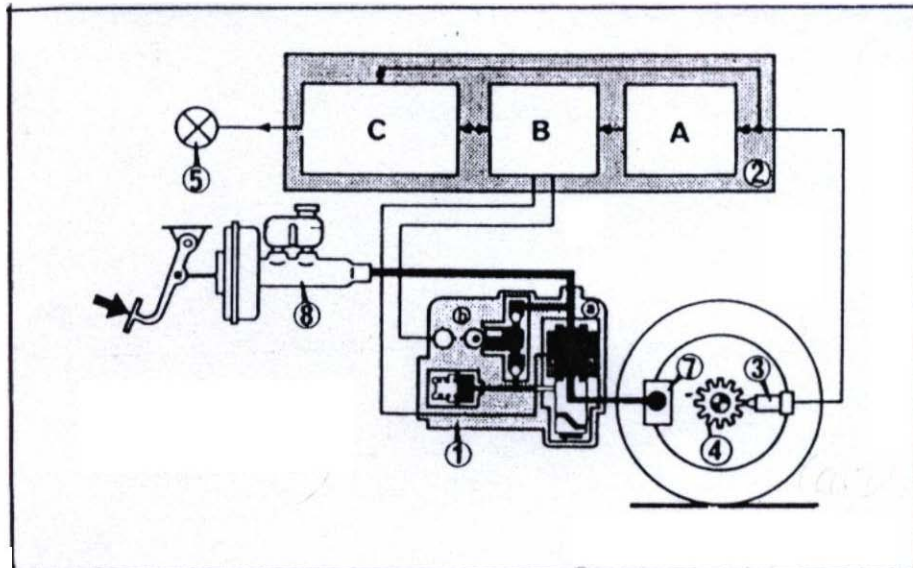
Figura 10. ( Del libro “Tecnologías avanzadas del automóvil”.)
