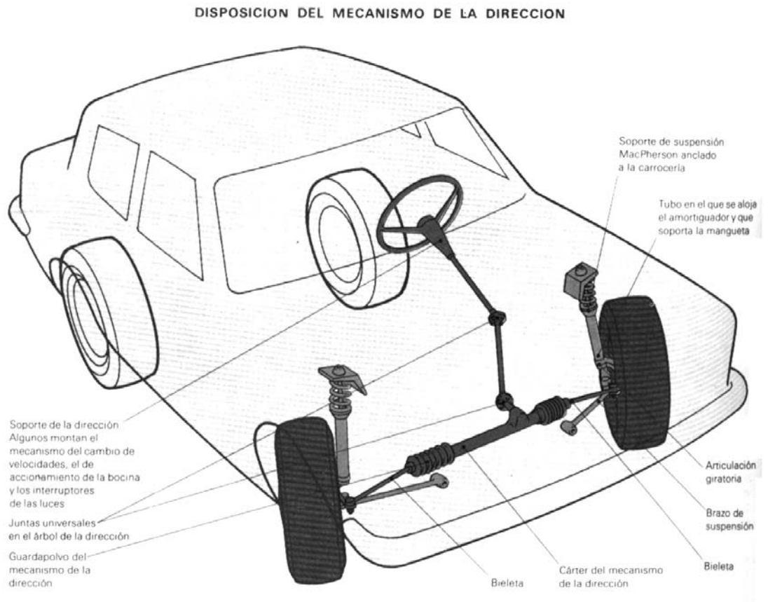
Figura 15.-Disposición del mecanismo de la dirección.( “El Automóvil” Selecciones de Reader s Digest)
