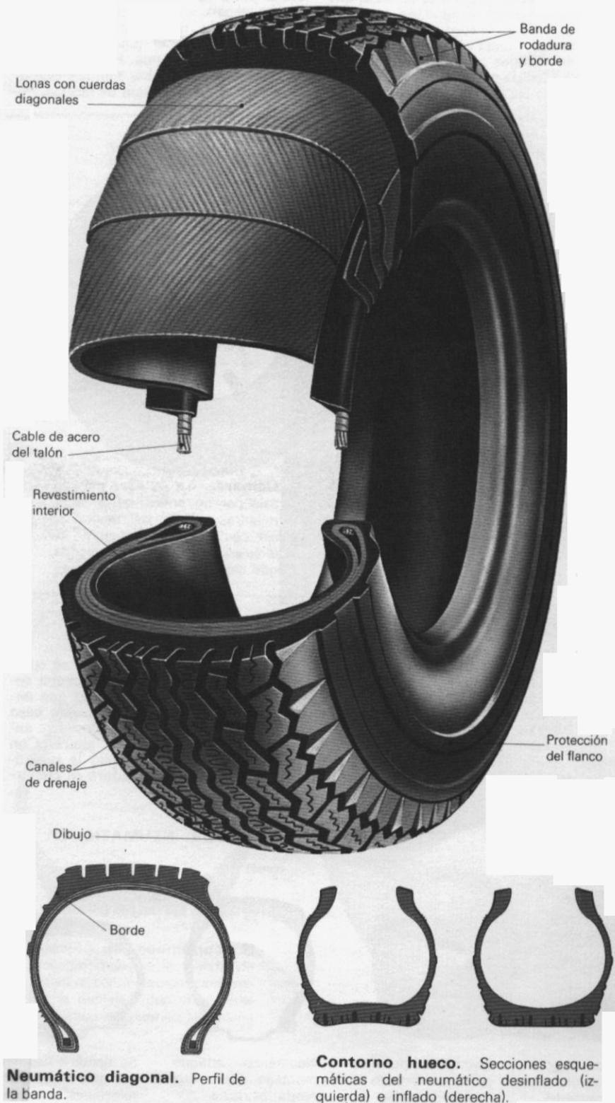
Figura 20. ("El Automóvil" Selecciones de Reader s Digest.)
