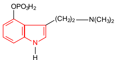
Psilocibina
