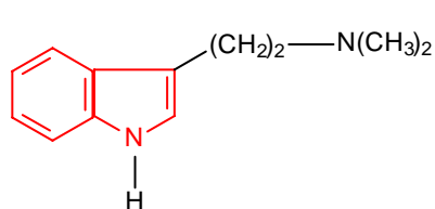
N, N-Dimetiltryptamina
