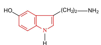
Serotonina
