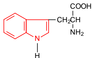
Triptófano
