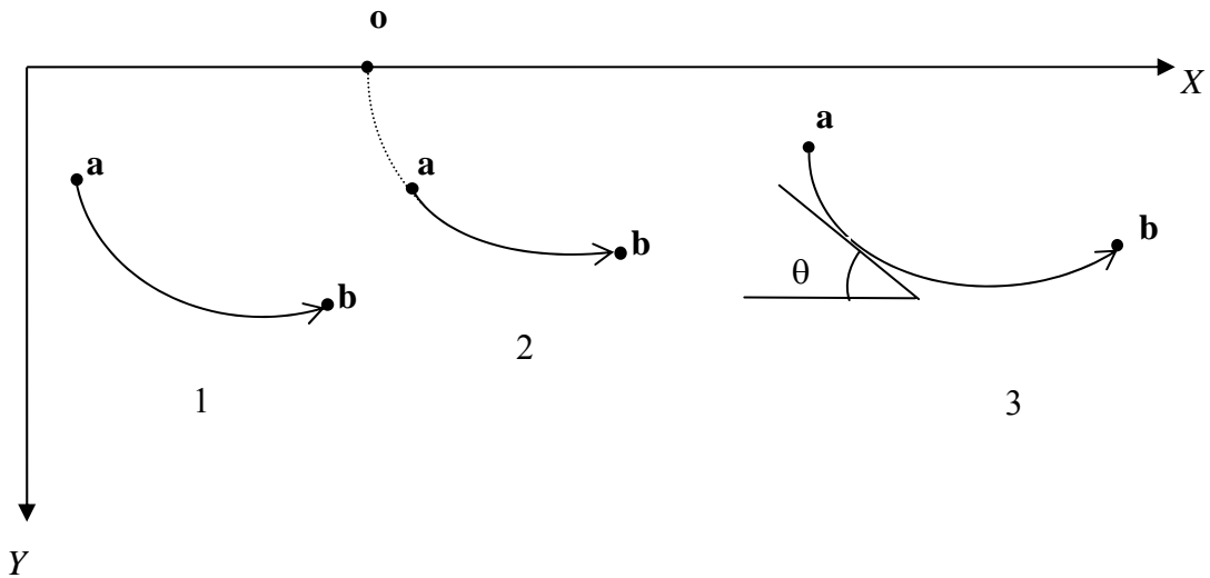
Fig. 4 Braquistócronas
