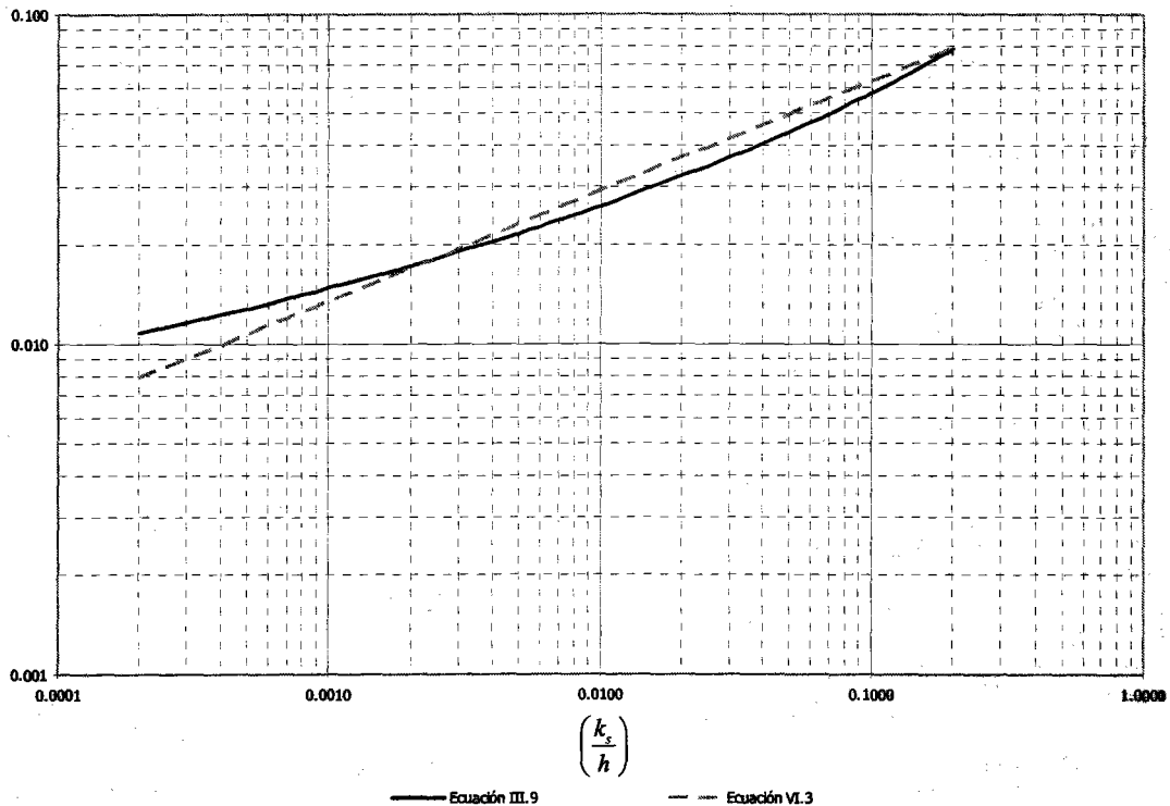
Figura 25.- Ajuste de potencia para el factor f .
