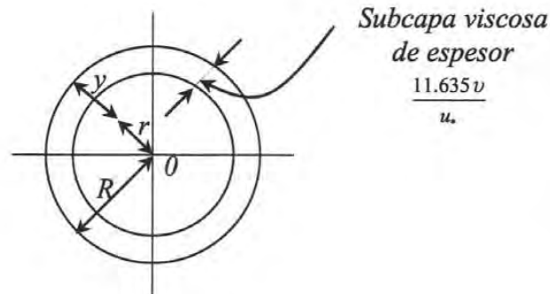
Figura 9.- Sección circular donde se considera la subcapa viscosa
