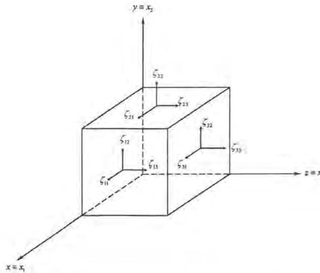
Figura 13.- Componentes del tensor de esfuerzos
