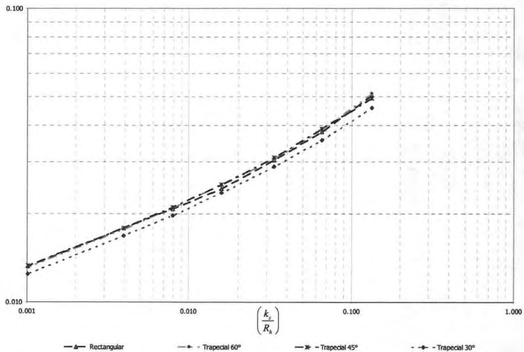
Figura 22.- Comparación de los valores de f para los resultados del modelo numérico sin incluir el caso del canal ancho.
