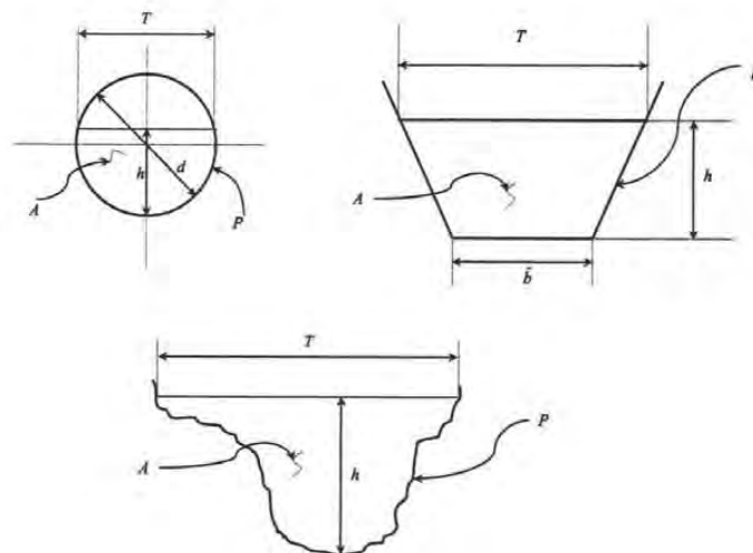
Figura 1.- Secciones transversales y sus características geométricas
