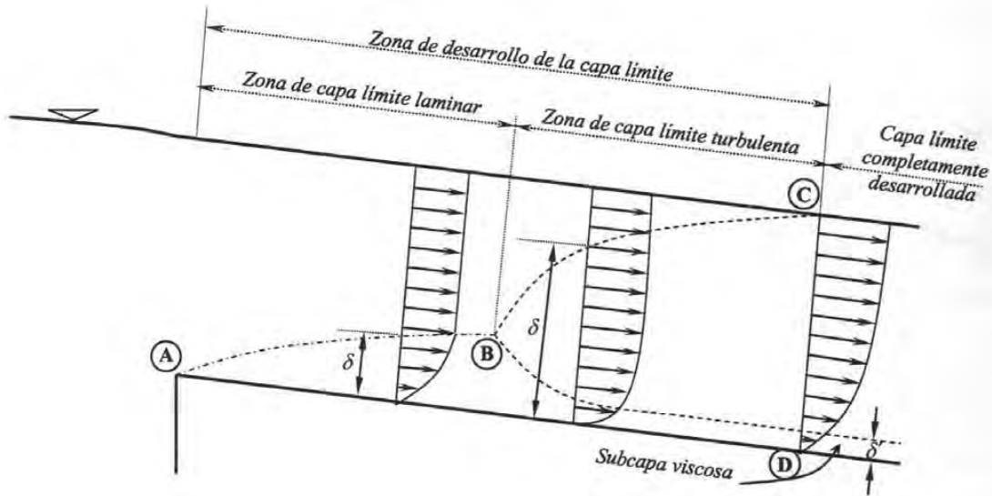
Figura 3.- Desarrollo de la capa límite en un canal abierto
