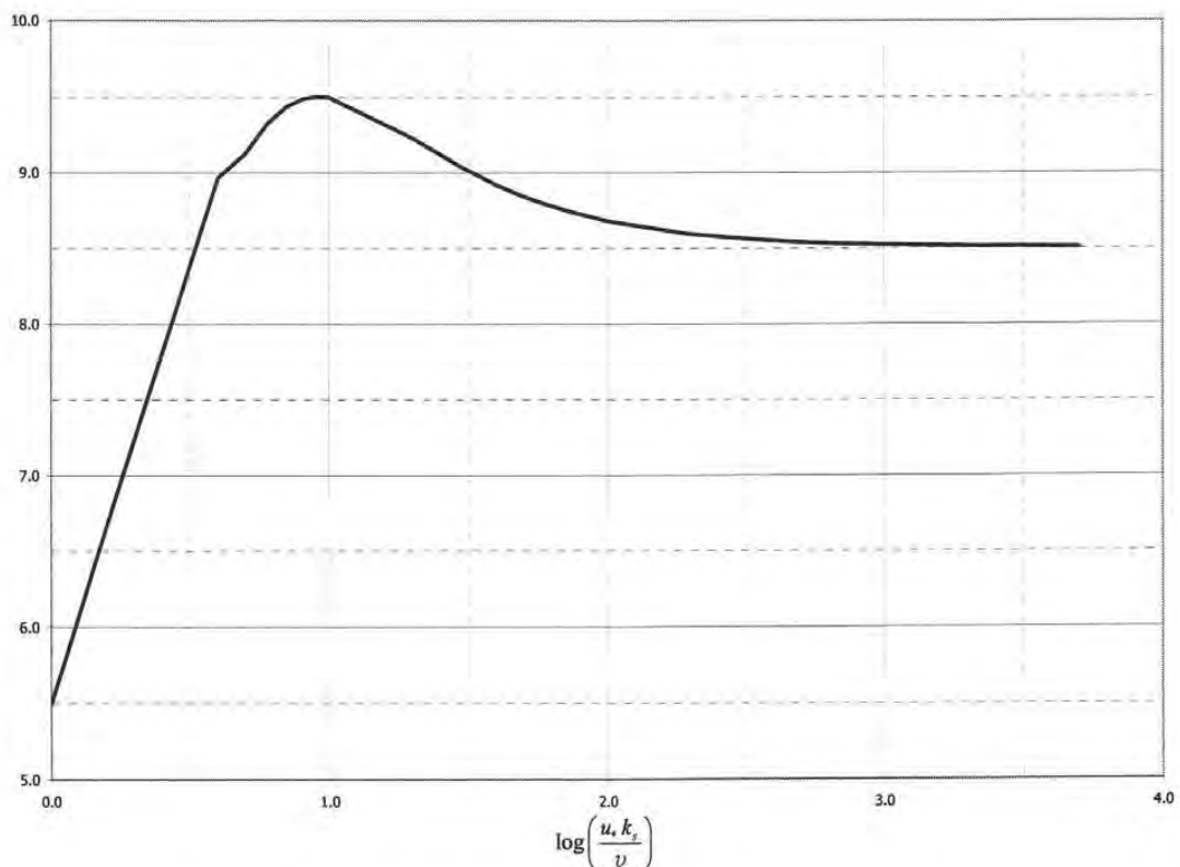
Figura 5.- Comportamiento del factor B para flujos turbulentos
