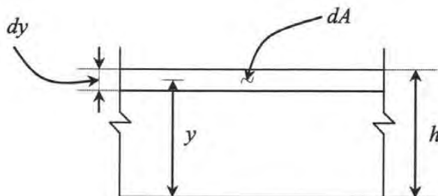
Figura 8.- Sección rectangular de ancho unitario
