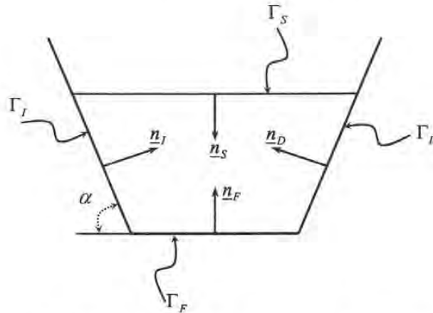
Figura 17.- Esfuerzos actuantes normales
