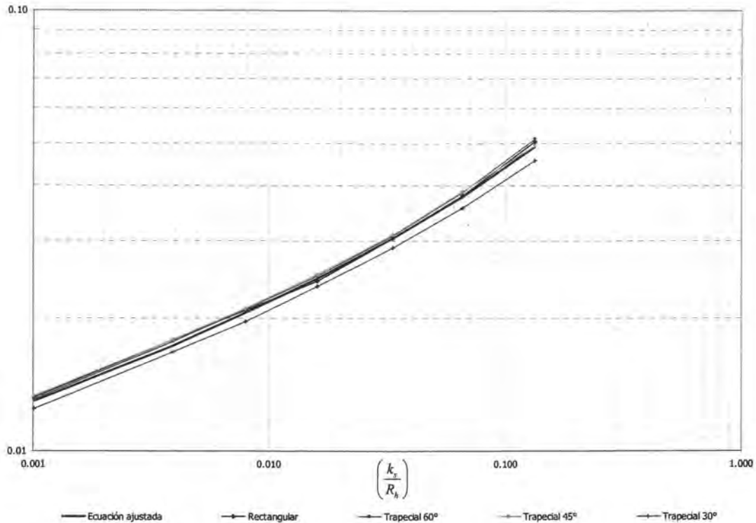
Figura 24.- Curvas para f obtenidas a partir de los resultados del modelo numérico y la curva para f del ajuste seleccionado.
