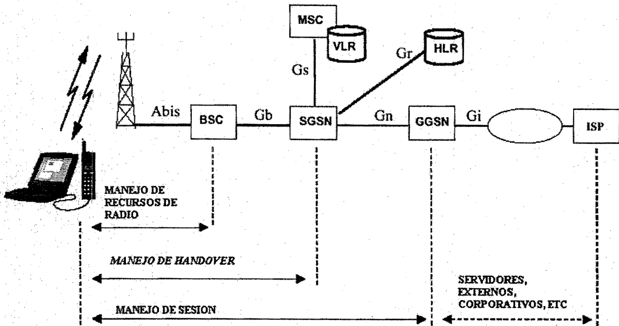
Figura 4.18. Funciones y tipo de Interfaz en una red GPRS.
