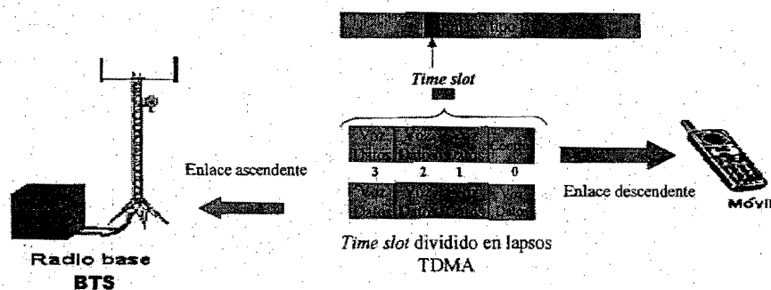
Figura 2.3. Ejemplo de tramas TDMA en GSM.
