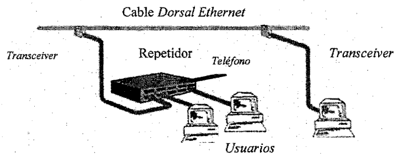
Figura 4.10. Conexión para un repetidor.
