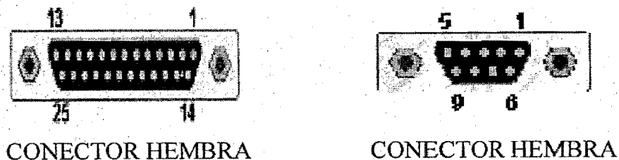
Figura 3.14. Dibujo de un conector DB-25 y DB-9.
