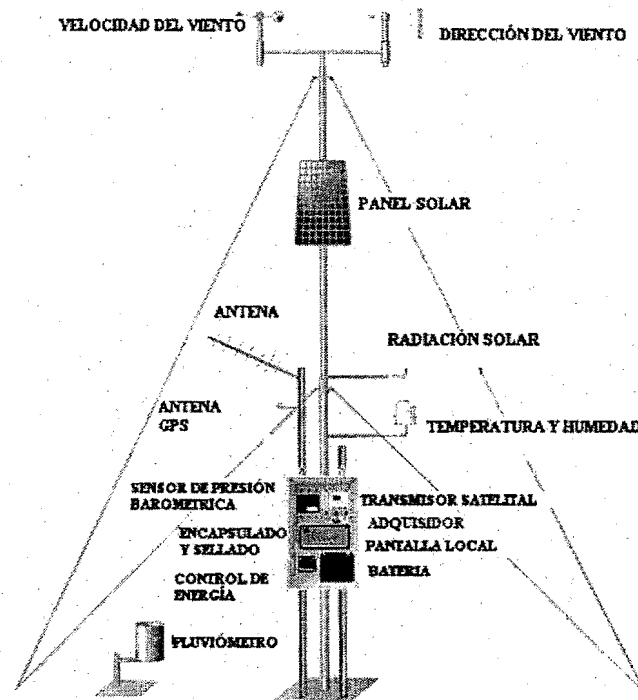
Figura 3.2. Elementos de una estación meteorológica.
