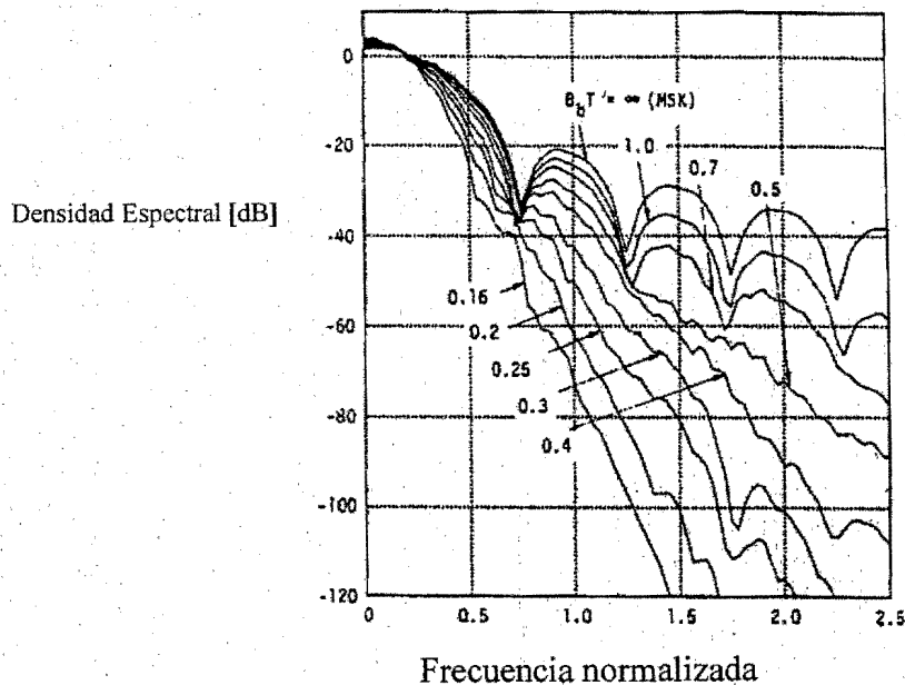
Figura B.3. Densidad de potencia espectral de una señal.
