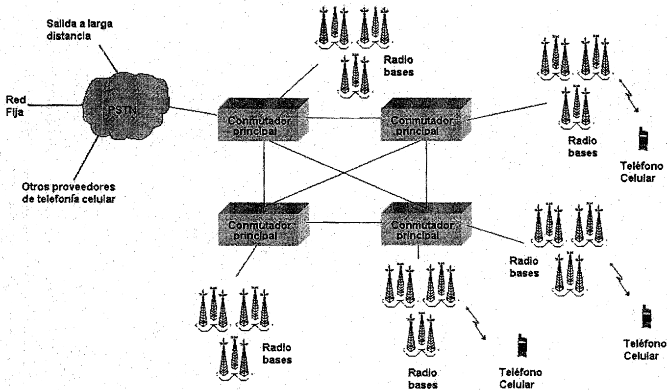
Figura 2.1. Red básica de telefonía celular.
