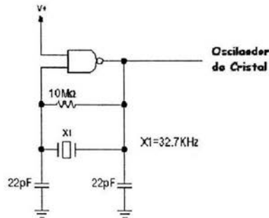
Fig. 5.6 Oscilador generador de portadora
