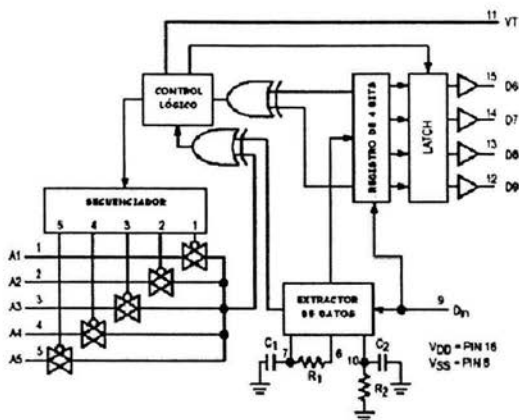
Figura 3.15 Diagrama de bloques del decodificador MC145027
