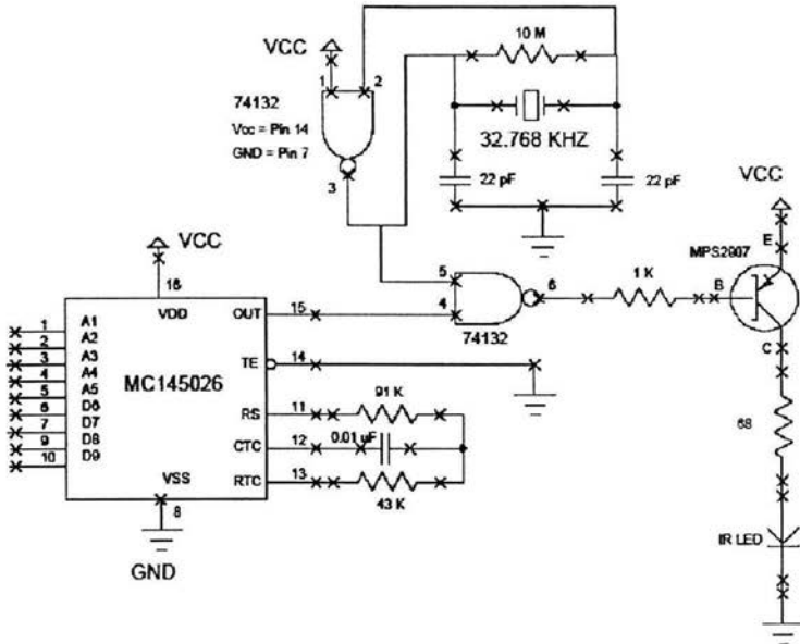
Figura 3.13 Módulo de Transmisión
