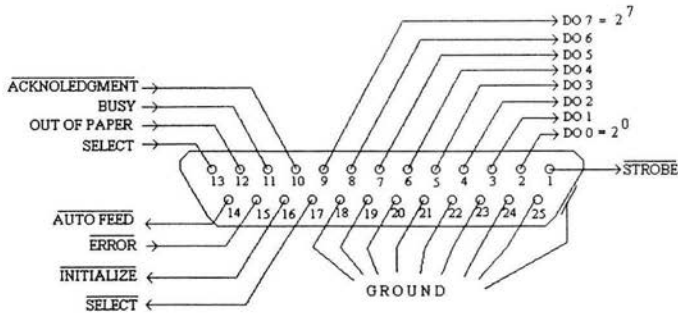
Fig. 2.2 Conector hembra DB-25S.
