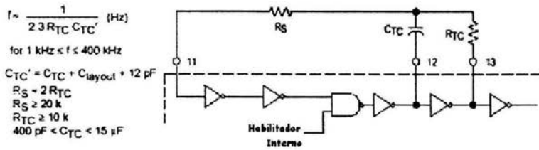
Figura 3.12 Oscilador RC.
