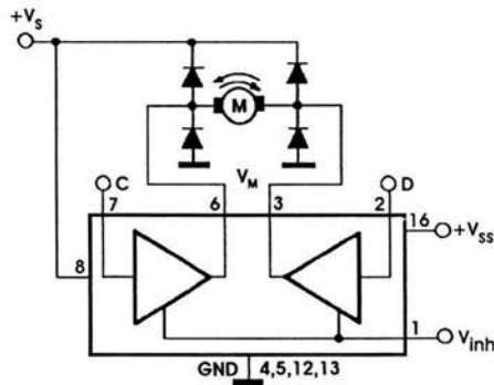
Fig. 4.9 Diagrama esquemático de un CI L293B
