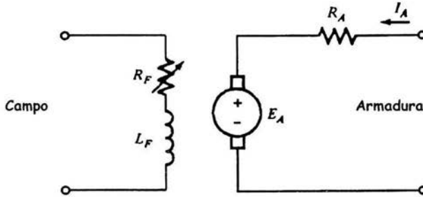
Fig. 4.2 Circuito equivalente de un motor de CD.
