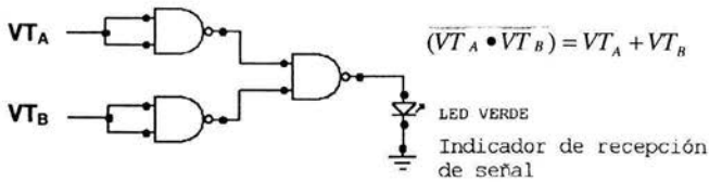
Figura 5.9 Arreglo de compuertas NAND para obtener OR.
