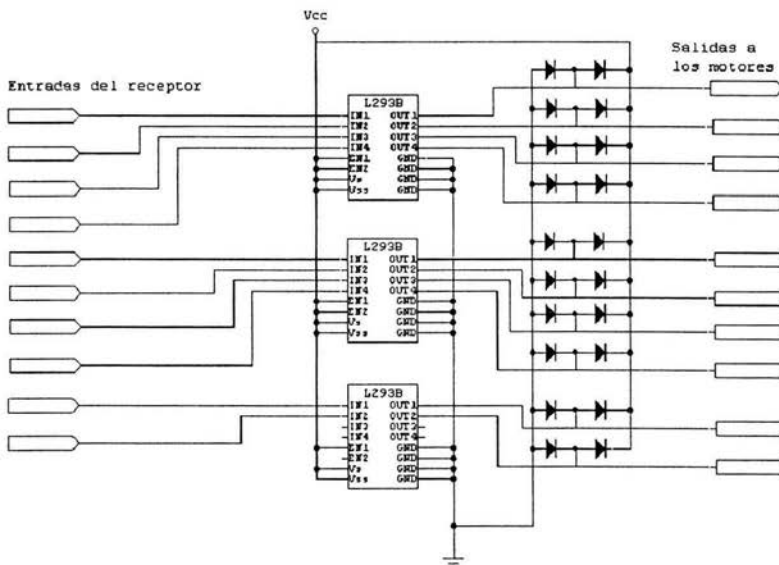
Figura 4.9 Esquema de conexión del circuito de potencia.
