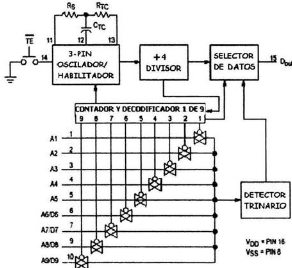
Figura 3.9 Diagrama de bloques del circuito MC145026
