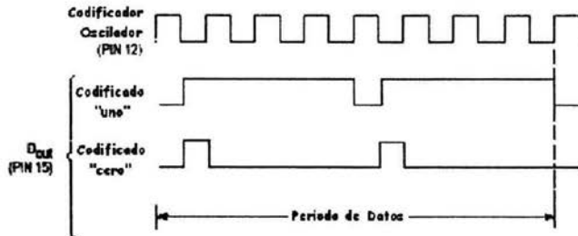
Figura 3.11 Codificación de estados.
