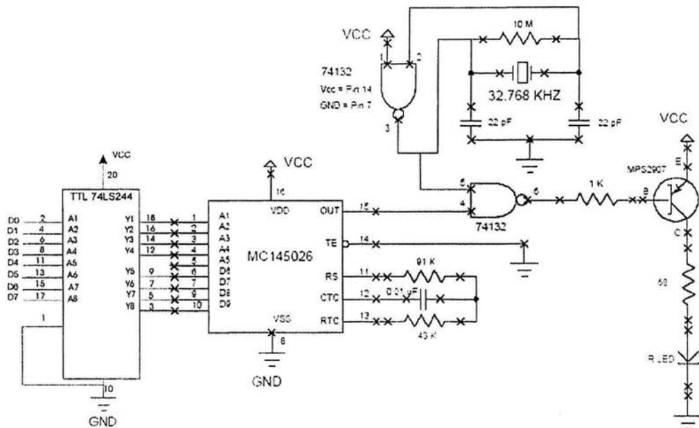
Figura 5.5 Integración de la Protección del Puerto Paralelo y el Transmisor
