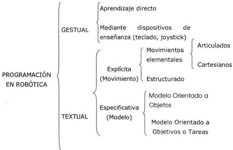
Figura 1.1 Clasificación de la Programación
