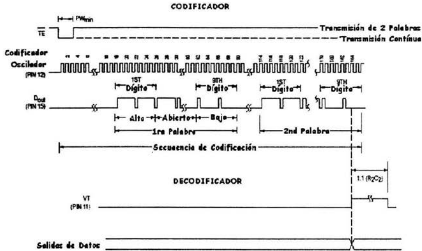
Figura 3.10 Diagrama de codificación y decodificación en el tiempo.
