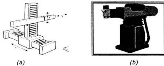
Fig. 1.4 Esquema de movimientos de coordenadas rectangulares. (b) Robot con configuración de coordenadas rectangulares.
