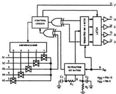
Diagrama de Bloques del Decodificador
