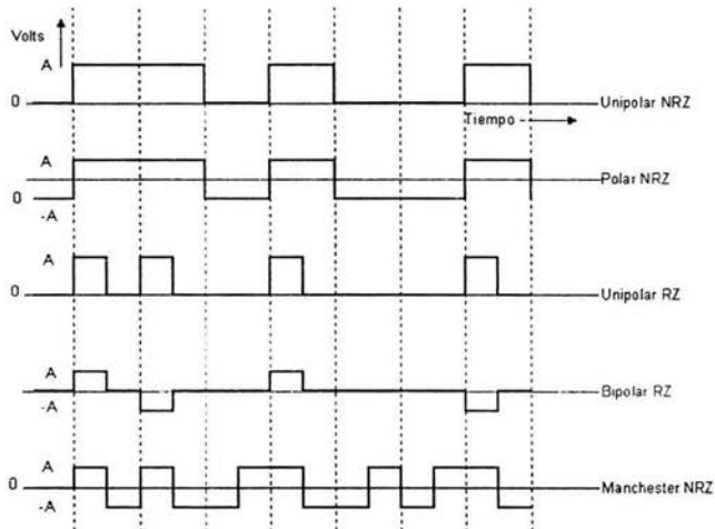
Figura 3.7 Formatos de Codificación Binaria
