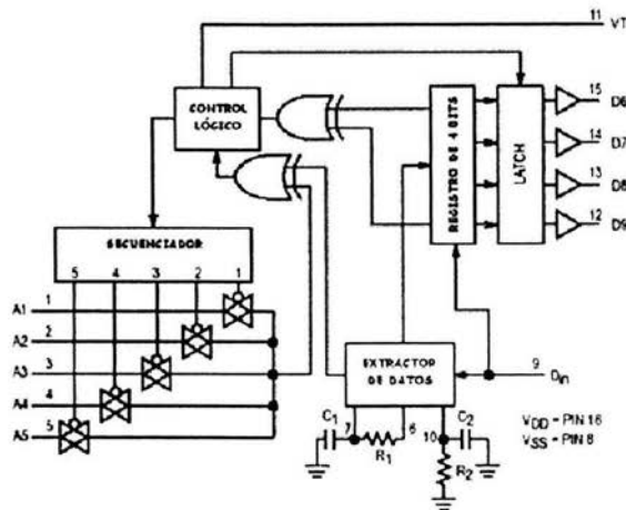
5.8 Diagrama de Bloques del Decodificador
