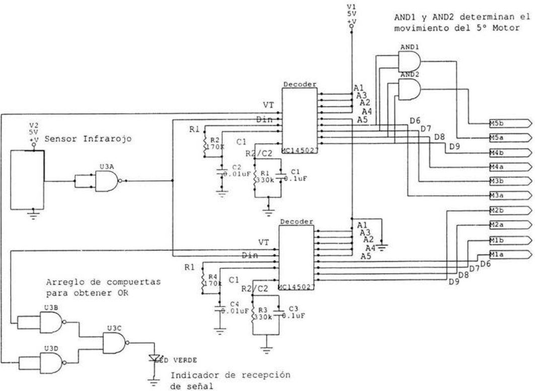
Figura 3.17 Diagrama Eléctrico del Circuito Receptor.
