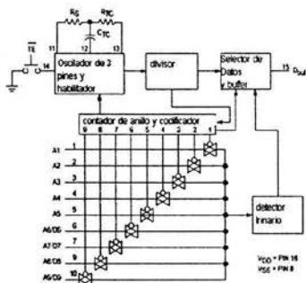
Diagrama de Bloques del Codificador
