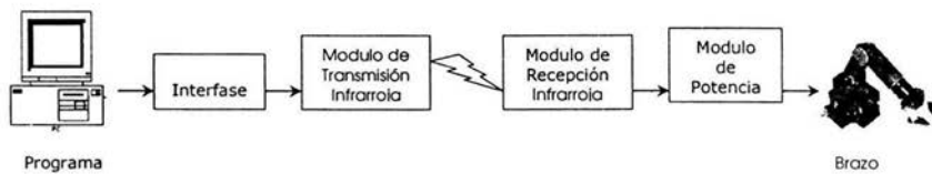
Fig. 5.1 Diagrama de Bloques del Sistema de Control
