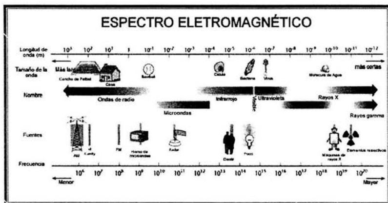
Figura 3.6 Espectro Electromagnético.
