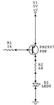
Figura 5.7 Amplificación de la señal
