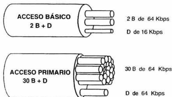
Figura 1.14 Acceso Básico y Primario
