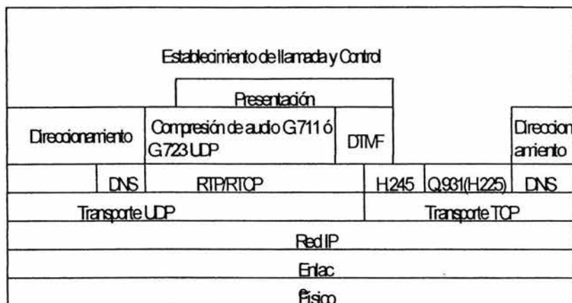
Figura 3.1 Pila de protocolos en VoIP
