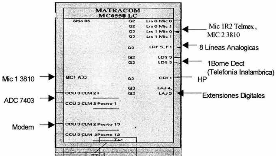
Figura 4.12 Conexiones Colima
