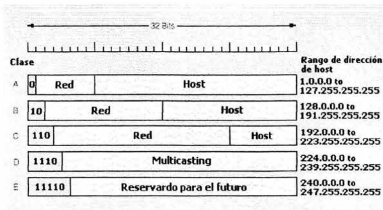
Fig. 2.6 Formatos de dirección IP
