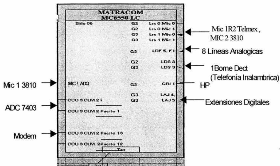
Figura 4.8 Conexión Morelos
