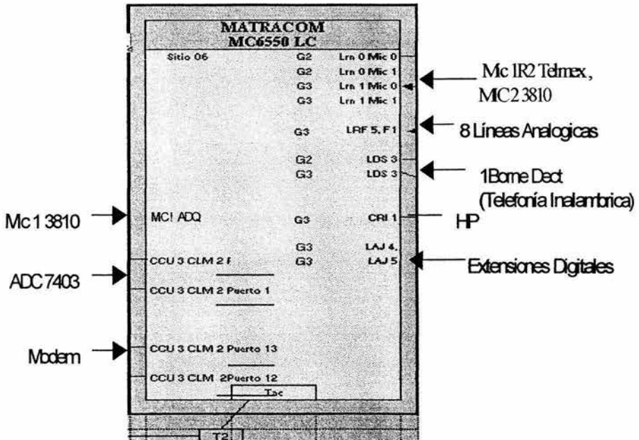
Figura 4.10 Conexión Oaxaca
