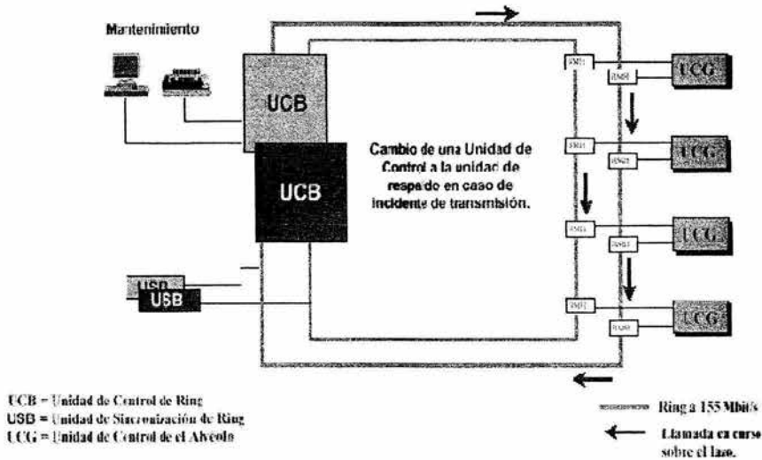
Figura 4.5 Estructura MC65650 (MATRA)
