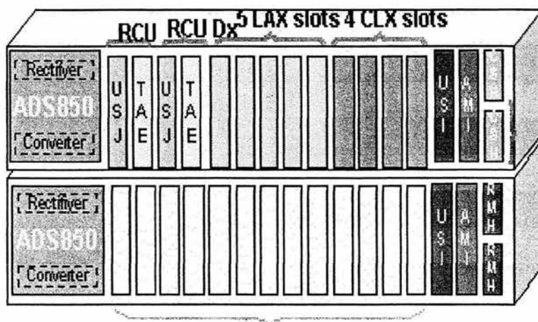
Figura 5.1 Equipo M6550 IP
