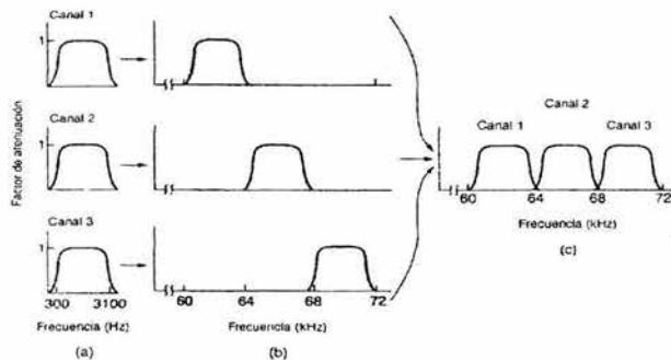
Figura 1.4 Multiplexación por División de Frecuencia (FDM)
