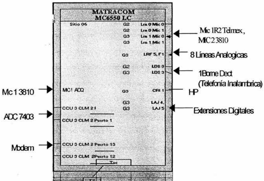
Figura 4.14 Conexiones Sinaloa
