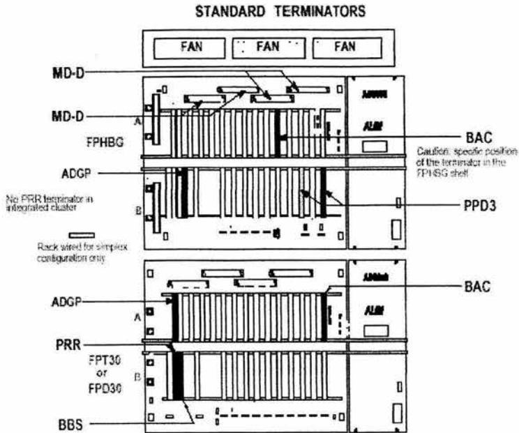
Figura 5.6 Parte posterior del equipo y sus adaptadores
