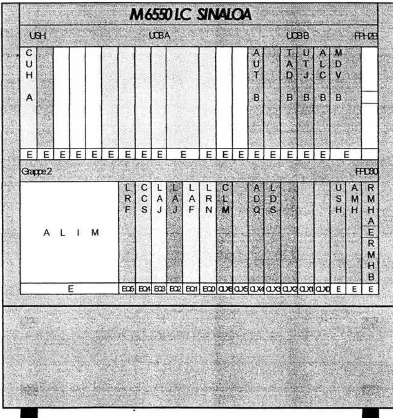
Figura 4.13 Bastidor Sinaloa
