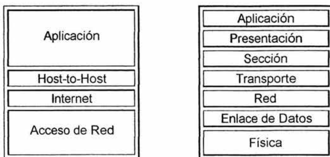
Figura 2.1 Demostración de las capas del modelo DOD y OSI.
