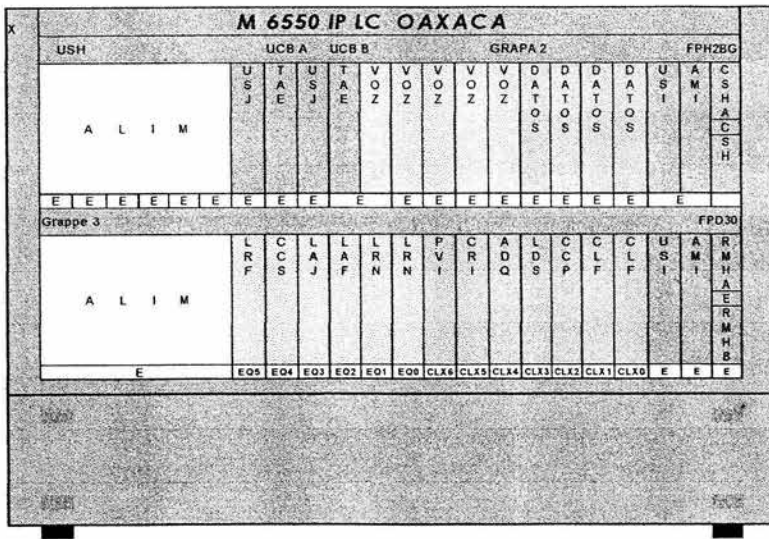
Figura 5.7 PABX M6550 IP Oaxaca
