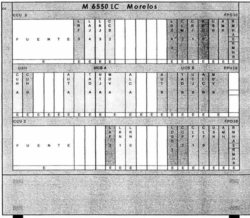
Figura 4.7 Bastidor Morelos
