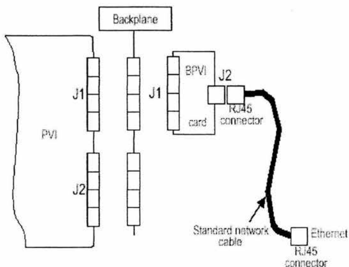
Figura 5.5 Adaptador Ethernet
