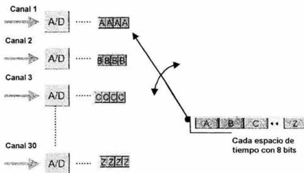
Figura 1.5 TDM (Multiplexación por División de Tiempo)
