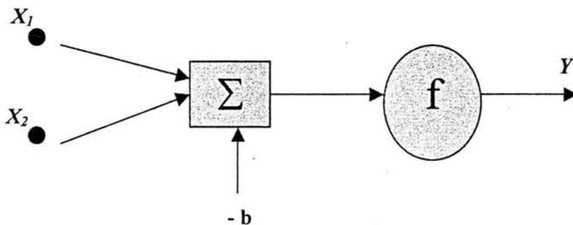
Figura 4.7 Estructura de una red tipo perceptrón
