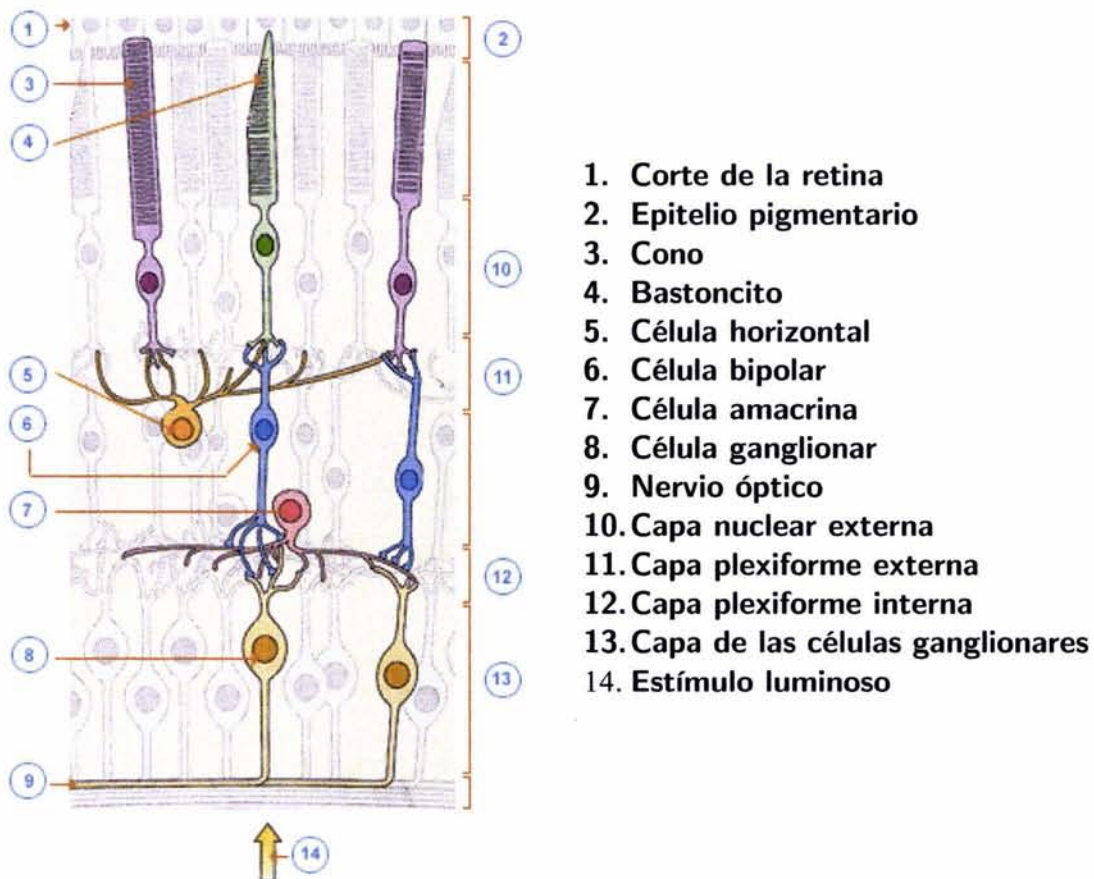
Figura 1.4 Estructura de la retina
