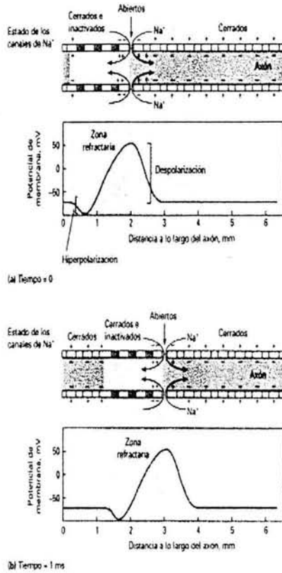
Figura 2.3 Potencial de acción
