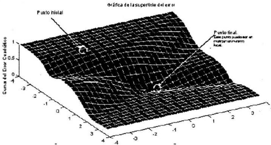
figura 4.12 Búsqueda del mínimo absoluto en la superficie de error
