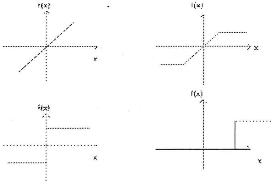
figura 4.5 funciones de activación usadas por una red neuronal artificial
