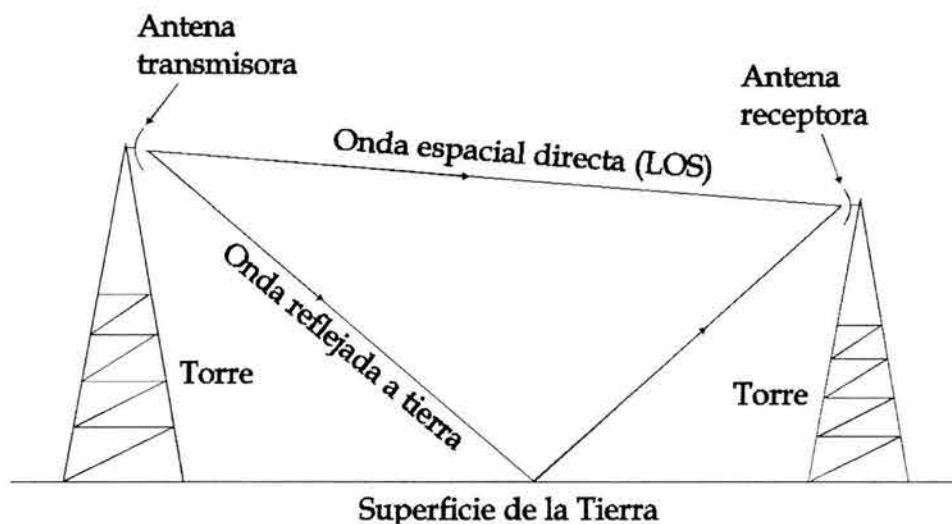
Fig. 2.6 Propagación de ondas espaciales.
