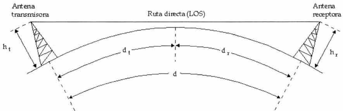
Fig. 2.7 Onda directa y curvatura de la Tierra.
