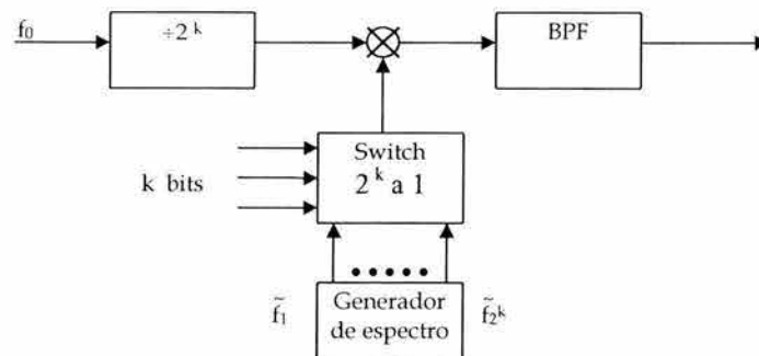
Fig. 3.19 Sintetizador de Frecuencia Directo.
