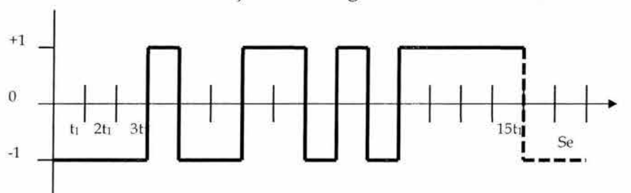
Fig. 3.17 Código de pseudo ruido con cuatro compuertas.
