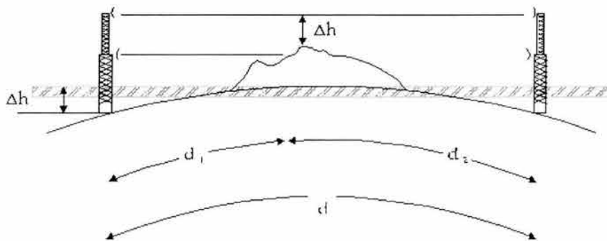
Fig. 2.10 Incremento de altura debido a la curvatura terrestre
