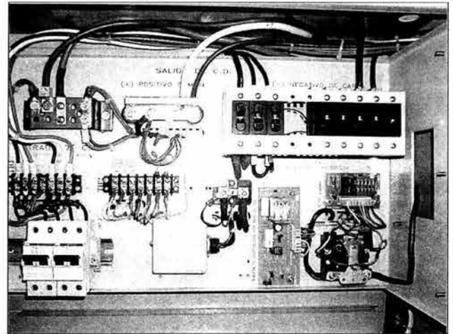
Posición asignada en el rectificador para aumentar el radio
