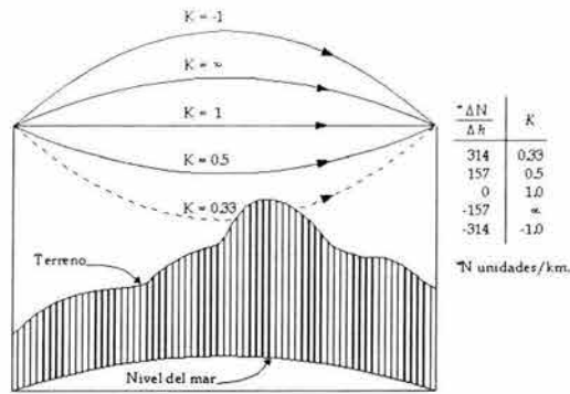
Fig. 2.9 Onda emitida con distintos valores de K.
