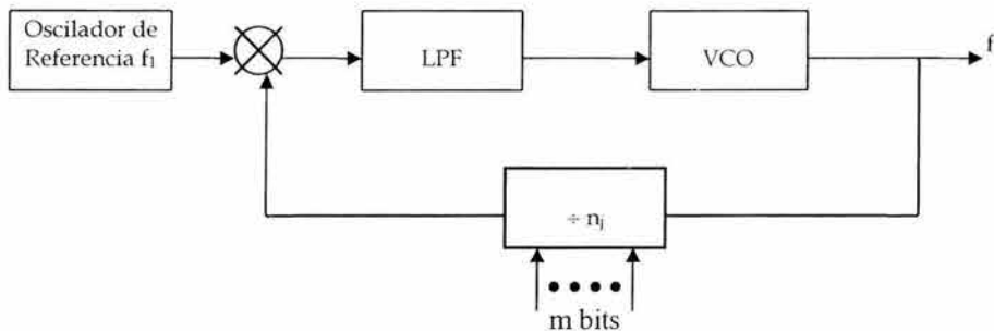
Fig. 3.20 Sintetizador de Frecuencia Indirecto.
