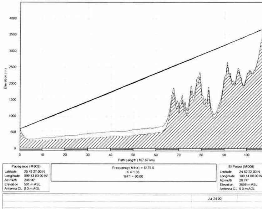
Fig. 5.1 Perfil utilizando el primer método de graficación, Criterio de libramiento 60% de la 1a zona de Fresnel con K=4/3 .
