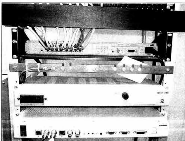
Barra de tierra donde se aterriza el Radio en el Bastidor
