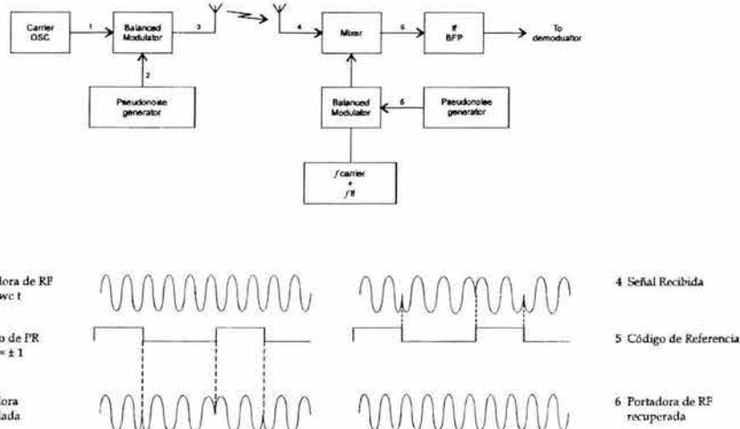
Fig. 3.7 Exhibición del sistema de Secuencia Directa mostrando las formas de onda.
