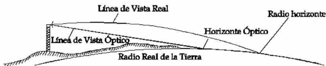
Fig. 2.8 Curvatura del Haz y radio horizonte.
