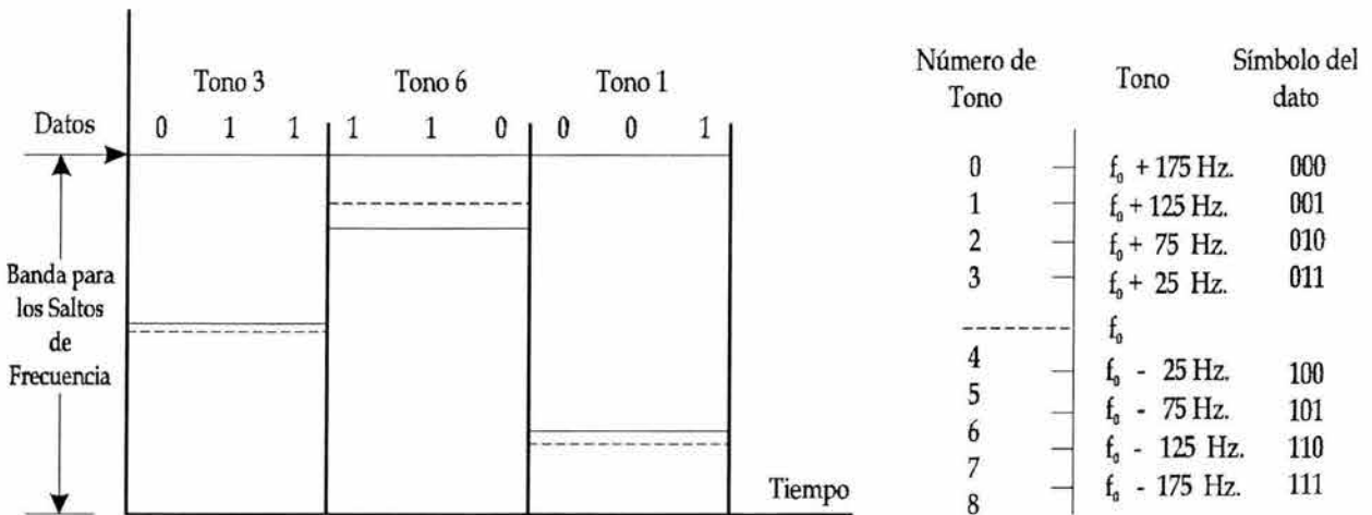
Fig. 3.11 Ejemplo de Saltos de Frecuencia utilizando una modulación 8-ary FSK.
