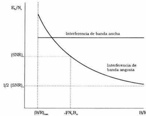
Fig. 3.22 Energía y utilización del Ancho de Banda Para un sistema de espectro disperso.
