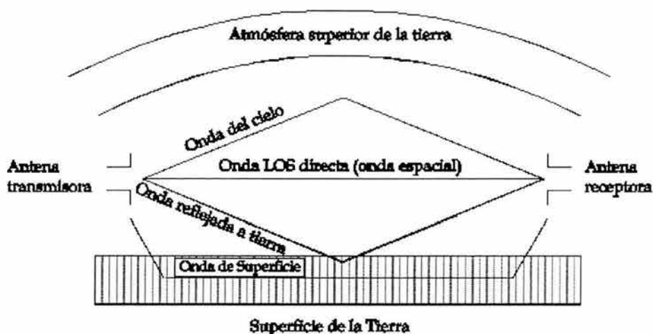
Fig.2.5 Modos normales de la propagación de ondas.
