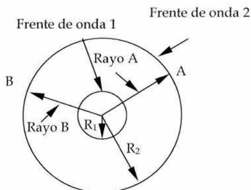
Figura 2.1 Fuente de onda esférica de una fuente isotrópica
