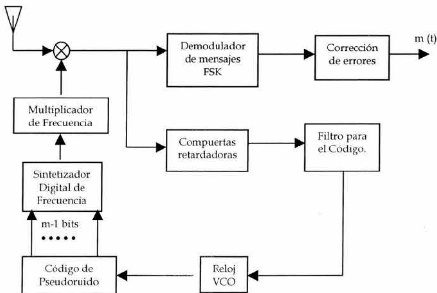
Fig. 3.21 Receptor No coherente para Saltos de Frecuencia.
