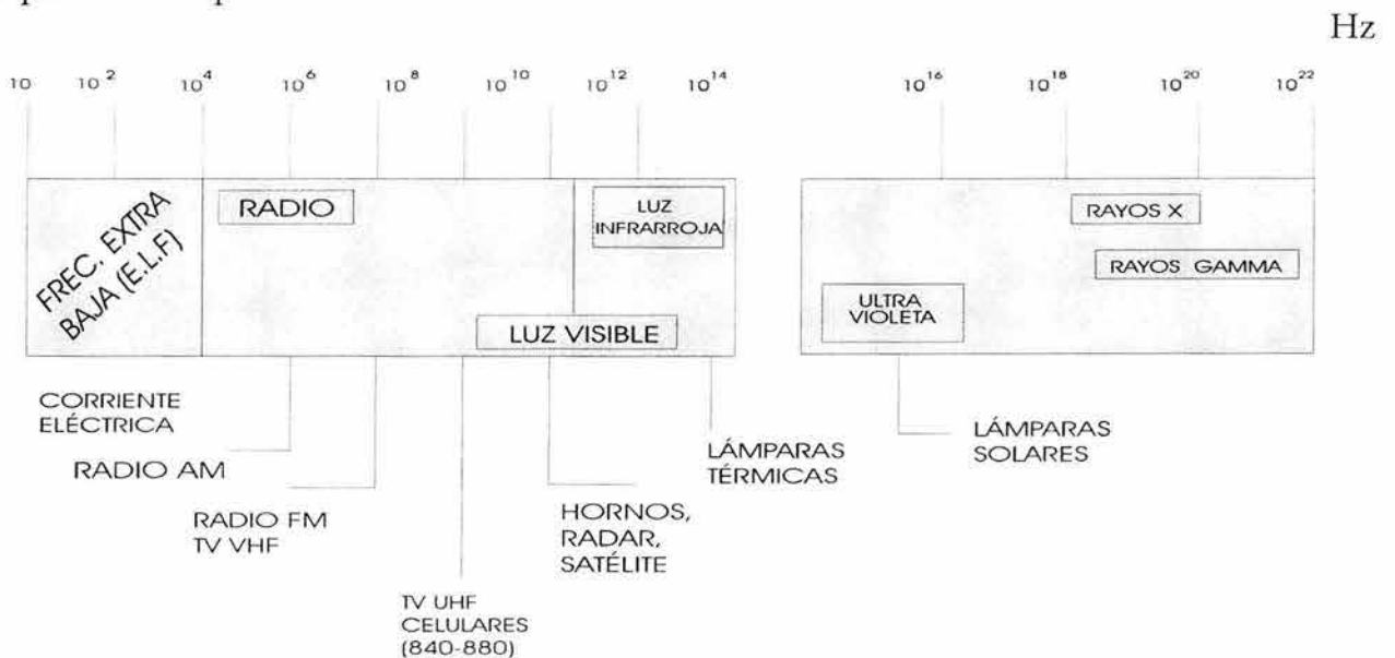
Fig. 1.1 Espectro radioeléctrico
