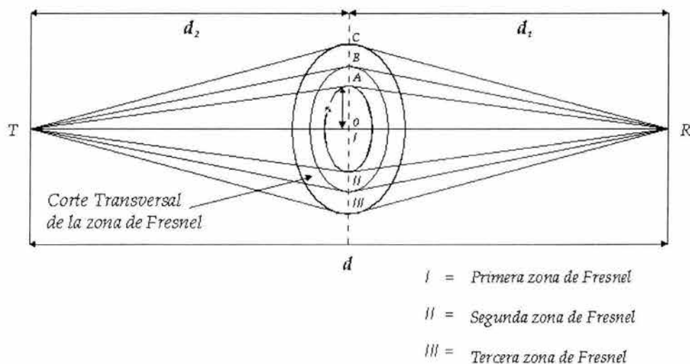
Fig. 2.11 Zonas de Fresnel.
