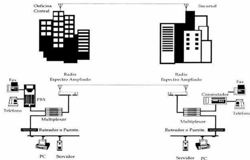
Fig. 4.1 Ejemplo de una aplicación real con radios de espectro disperso.
