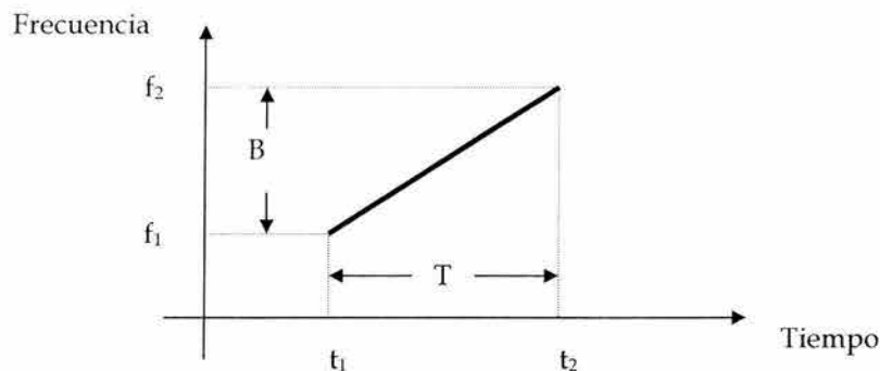
Fig. 3.15 Señal Chirp.
