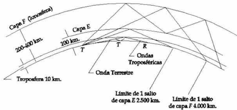
Figura 2.3 Algunas líneas de propagación posibles
