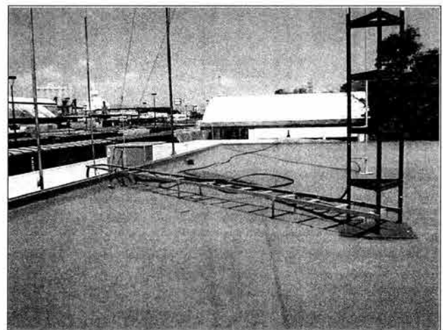
Recorrido de la escalera de Pie de Torre a Pasamuros externo
