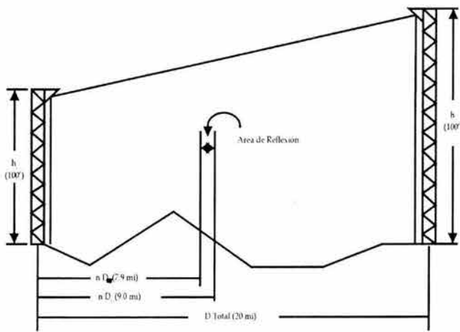
Fig. 5.5 Ejemplo del cálculo del punto de reflexión.
