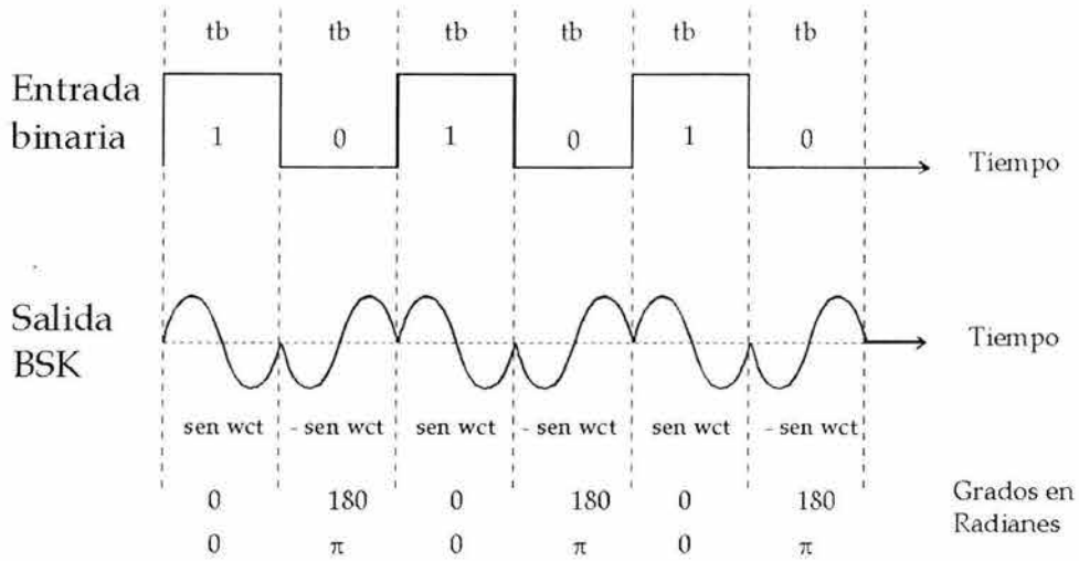
Fig. 3.5 Relación de la fase de salida contra tiempo para un modulador de BPSK
