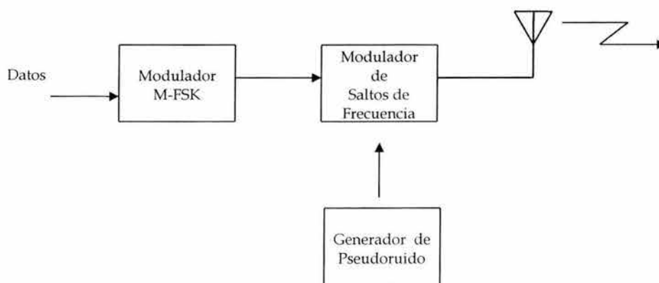
Fig. 3.9 Sistema Transmisor de Saltos de Frecuencia
