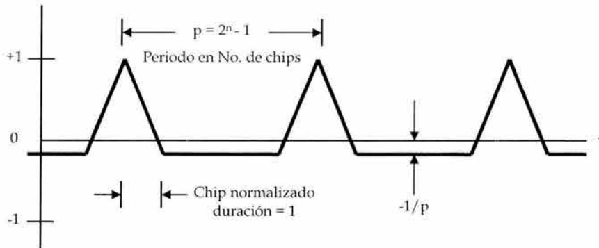
Fig. 3.18 Función de Autocorrelación para el Código de pseudo ruido.
