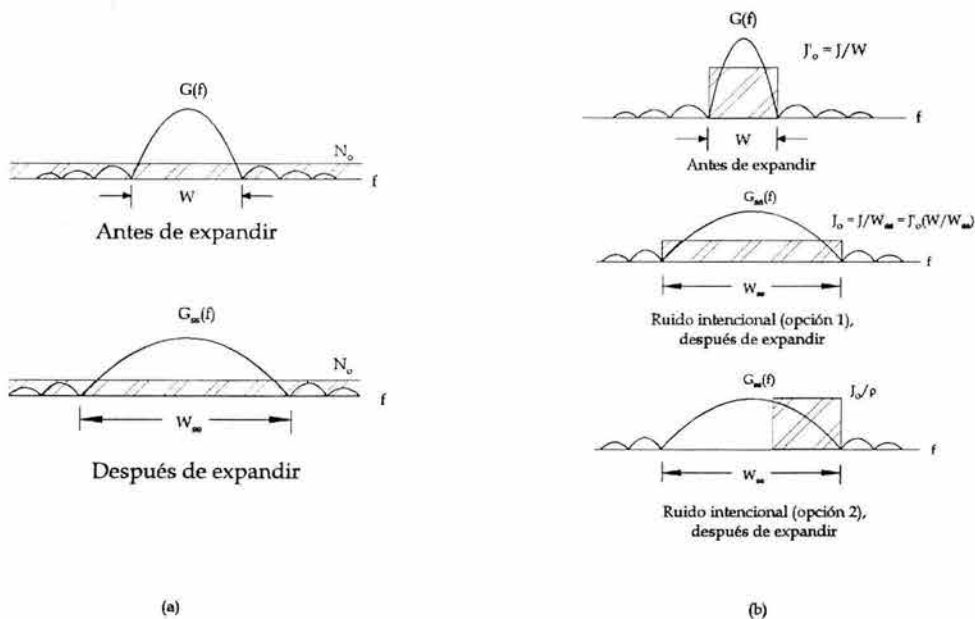
Fig. 3.2 Efecto del espectro disperso. (a) Espectro disperso en presencia de ruido blanco.
