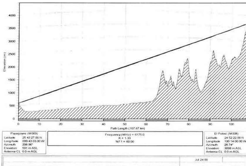
Fig. 5.1 Perfil utilizando el segundo método de graficación, Criterio de libramiento 60% de la 1a zona de Fresnel con K=4/3 Papel curvo.
