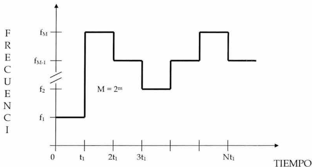
Fig. 3.8 Señal de Saltos de Frecuencia
