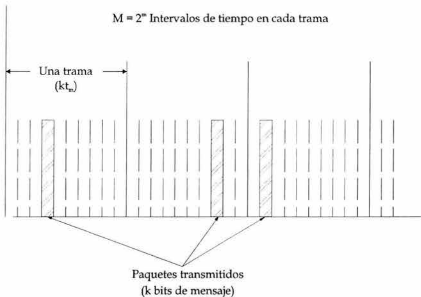
Fig. 3.13 Forma de onda para Saltos de Tiempo.
