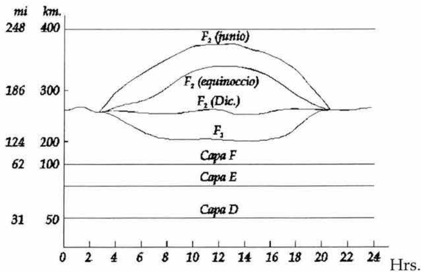
Figura 2.4 Capas Ionosféricas
