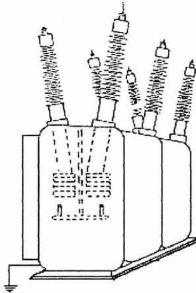
Fig. 3.1 El interruptor
