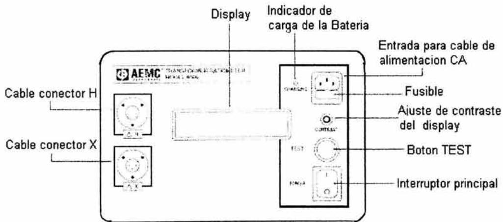
Fig. 2.17 Esquema superior del DTR Mod. 8500
