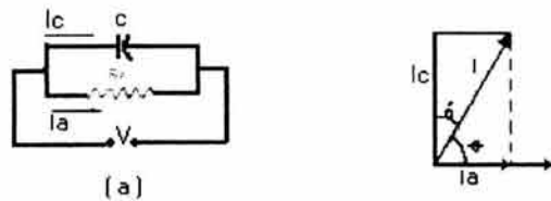
Fig. 2.15 Diagrama vectorial de pérdidas
