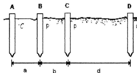
Fig. 5.3 Método del electrodo central 31
