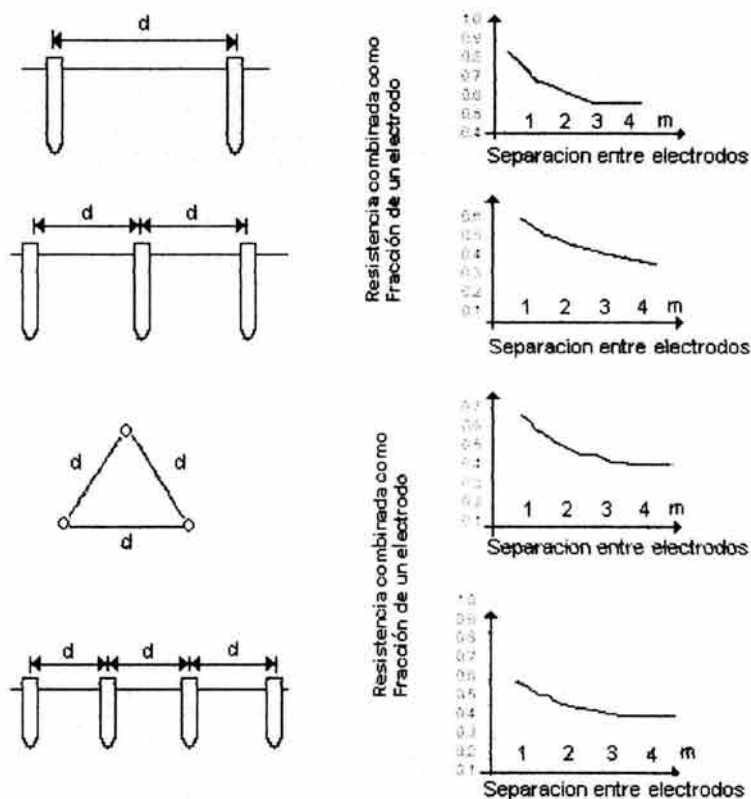
Fig. 5.10 Electrodos múltiples
