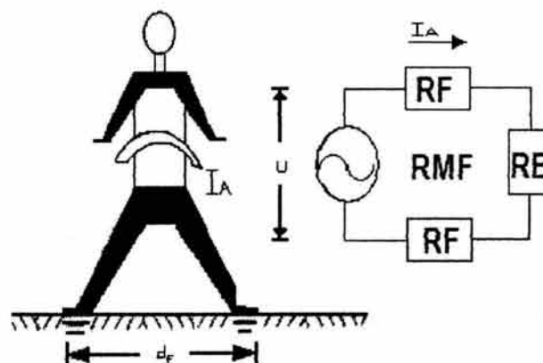
Fig. 5.6 Potencial de paso
