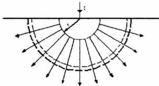
Figura 5.9 Electrodo hemisférico
