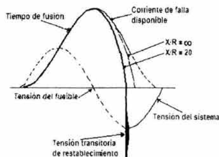
Fig. 3.5 Oscilograma de un fusible de expulsión
