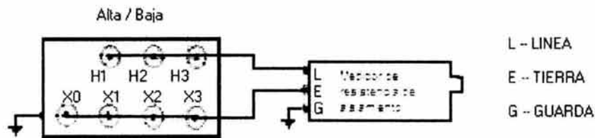
Fig. 2.11 Resistencia de aislamiento alta contra baja 3
