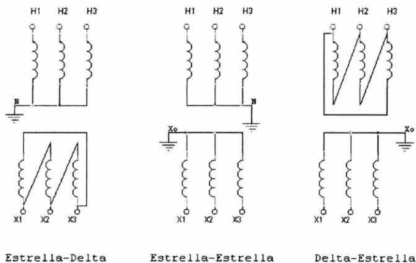
Fig. 2.5 Conexiones más utilizadas.
