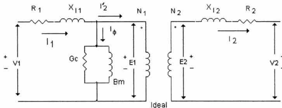
Fig. 2.3 Circuito equivalente del transformador
