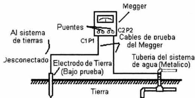
Fig. 5.13 Método de "dos puntos"
