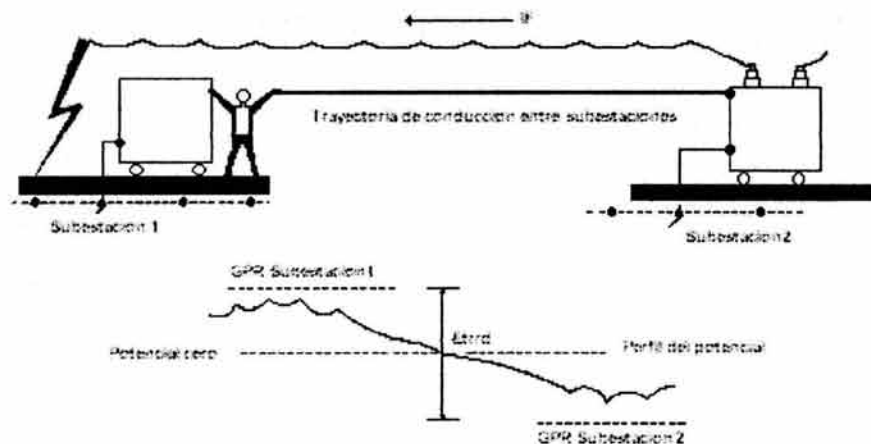
Fig. 5.7 Potenciales transferidos
