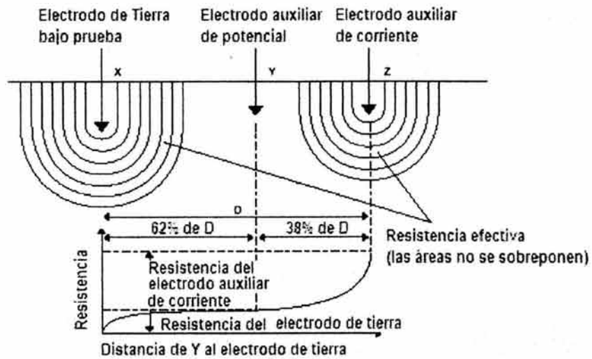
Fig. 5.12 Incremento gradual de la resistencia
