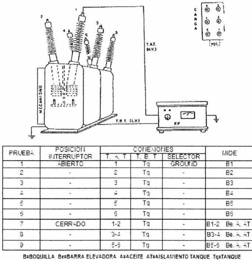
Fig. 3.12 Conexiones de la prueba de factor de potencia
