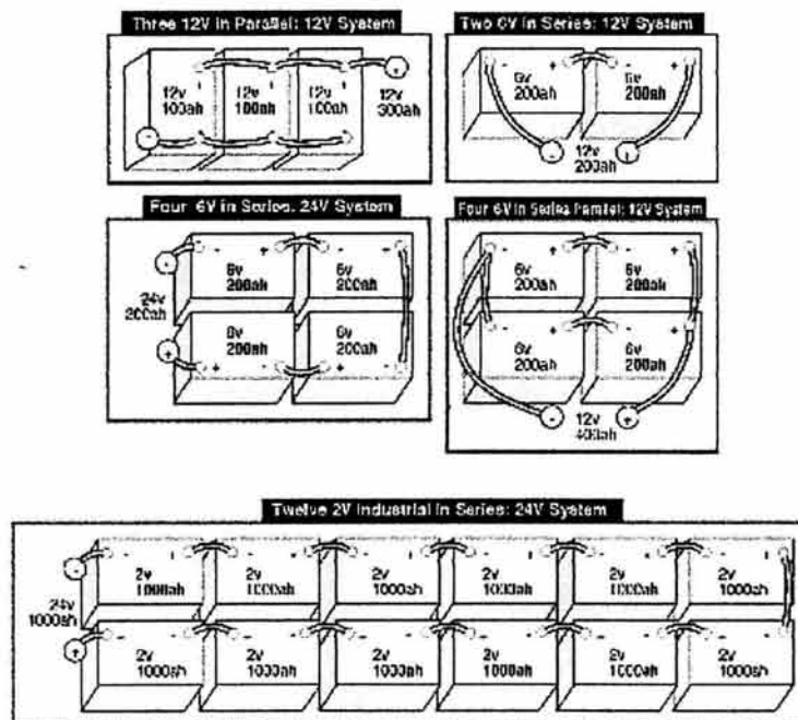
Fig. 4.2 Banco de baterías
