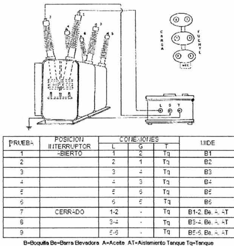
Fig. 3.8 Conexiones de la prueba de resistencia de aislamiento
