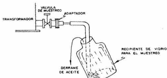
Fig. 2.20 Muestra de aceite
