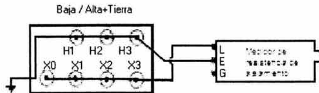
Fig. 2.13 Baja contra alta + tierra
