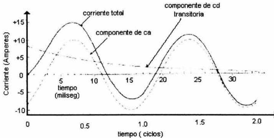
Fig. 3.2 Oscilograma de la corriente de cortocircuito.
