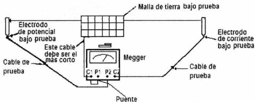
Fig. 5.14 Medición de la malla a tierra
