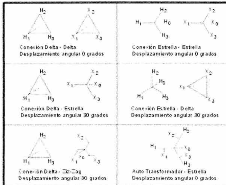
Fig. 2.6 Tipos de conexiones
