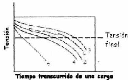
Fig. 4.4 Curvas características de descarga de baterías
