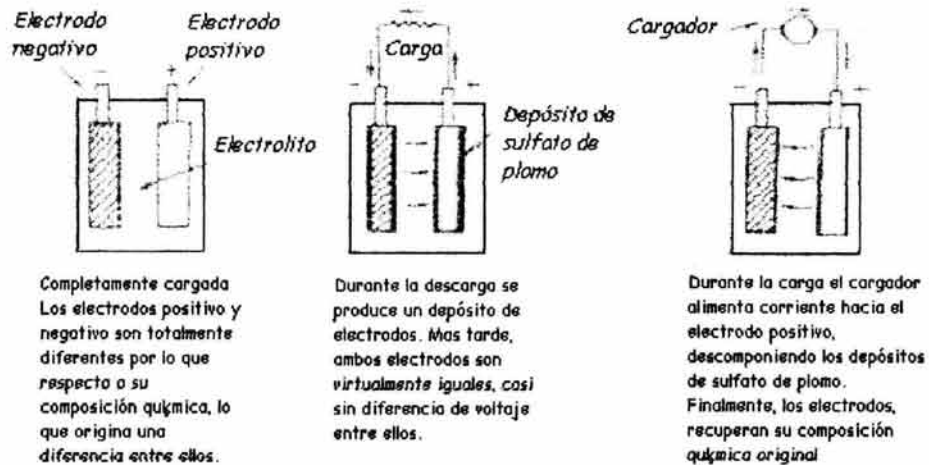
Fig. 4.5 Proceso para la carga de acumuladores
