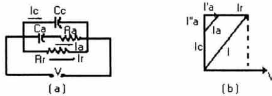
Fig. 2.14 Componentes de corriente alterna
