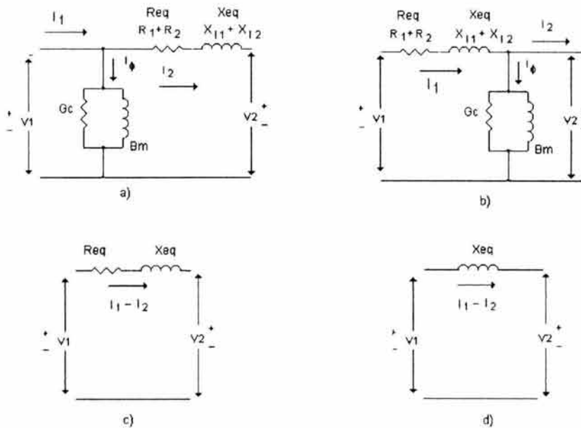
Fig. 2.4 Circuitos equivalentes aproximados del transformador
