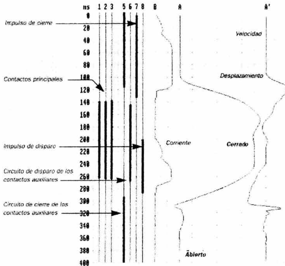
Fig.3.11 Gráfica de tiempos del interruptor (cierre y apertura).
