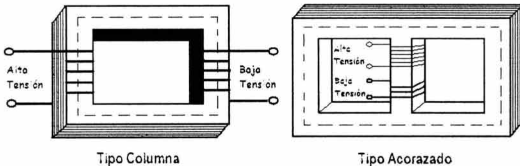
Fig. 2.1 Núcleos del transformador
