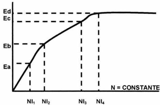
Fig. 2.23 Curva típica de saturación
