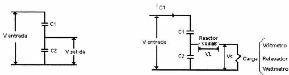
Fig. 2.9 Divisor de tensión
