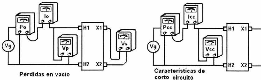
Fig. 2.22 Diagrama de conexiones para la determinación de las pérdidas en vacío y en cortocircuito.
