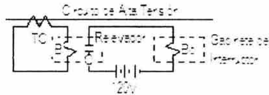
Fig.3.4 Circuito elemental de protección por sobrecorriente
