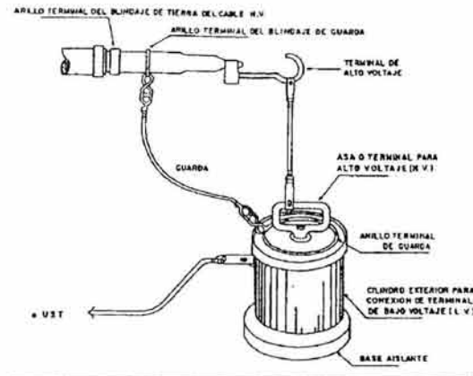
Fig. 2.21 Prueba de factor de potencia al aceite
