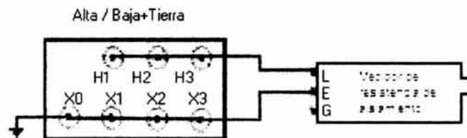
Fig. 2.12 Resistencia de aislamiento alta contra baja + tierra
