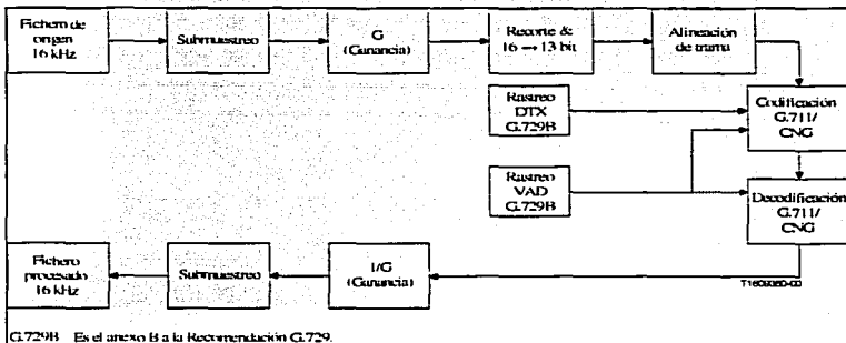
Figura III.46. – Procesamiento G.711 con CNNG.
