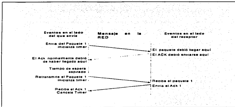
Figura 11.20.- Transmisión de Paquetes en Red.
