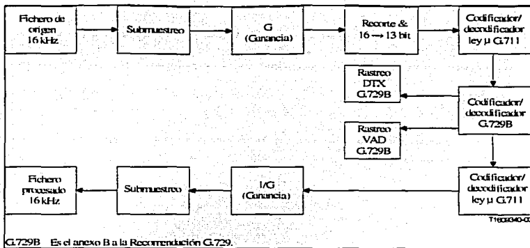
Figura III.45. – Procesamiento G.729B para Obtener Archivos de Rastreo VAD/DTX.
