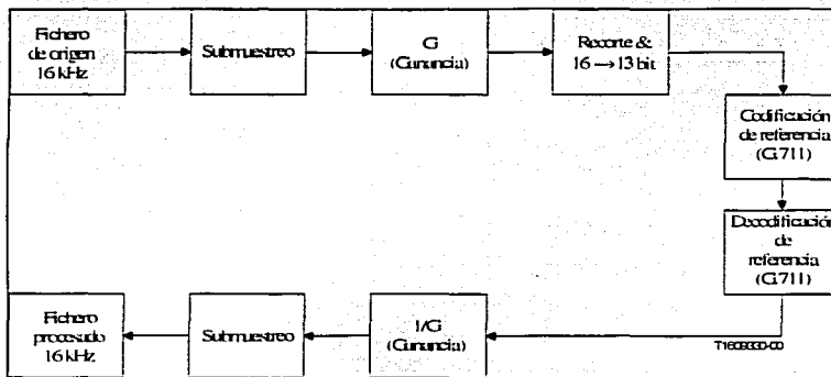
Figura III.44. – Procesamiento G.711 sin CNG.
