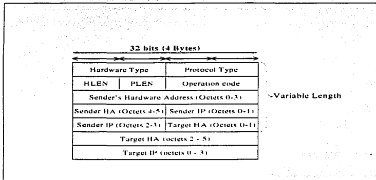
Figura II.6.- Formato de un Mensaje ARP.
