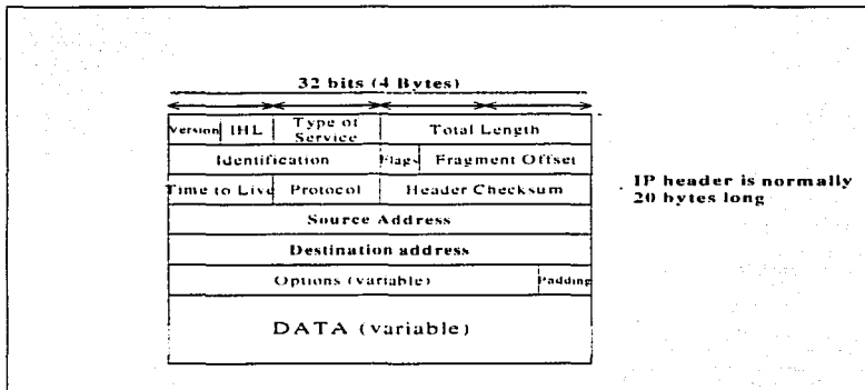
Figura II.4.- Campos del Datagrama.
