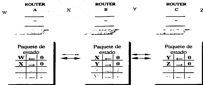
Figura II. 15.- RIP.
