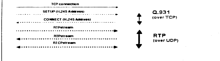
Figura III.25.- H.323 – FastStart.
