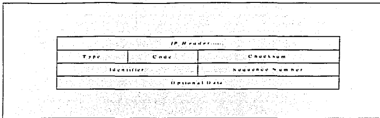
Figura II.7.- Formato del Paquete ICMP para Respuesta a Solicitud.
