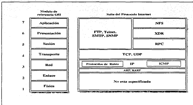
Figura II.2.- Familia de Servicios y Protocolos.
