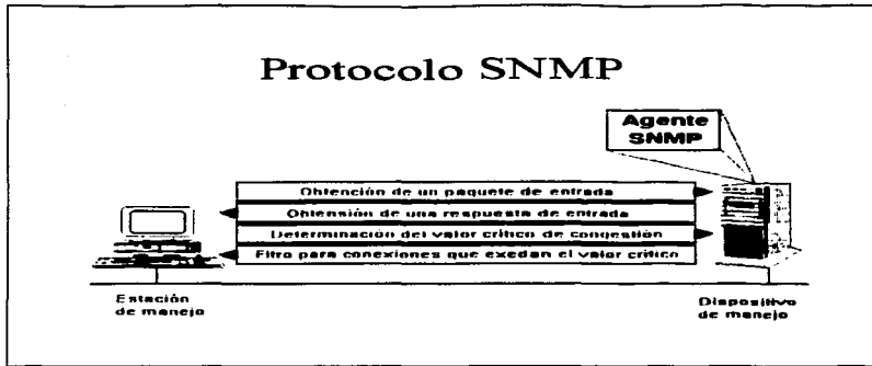
Figura II.31.- Protocolo SNMP.
