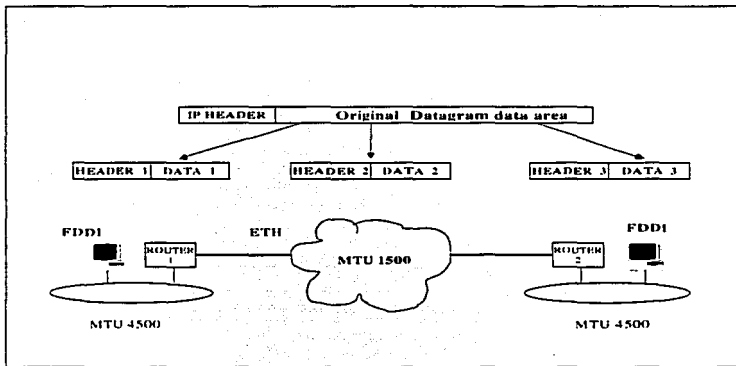
Figura II.5.- Fragmentación.
