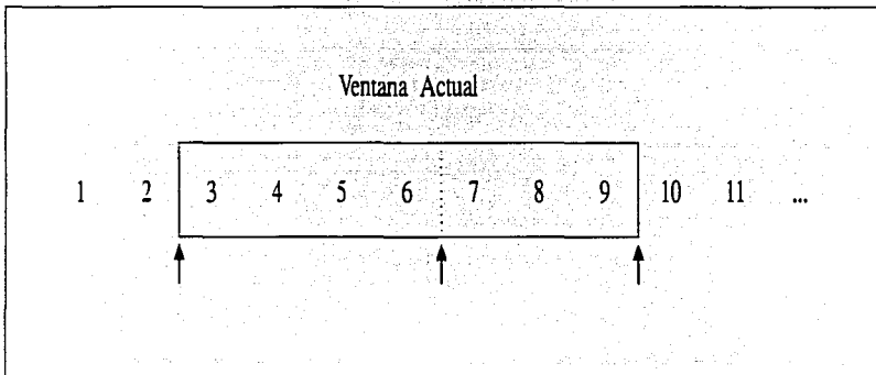
Figura II.23.- Ventana Actual.
