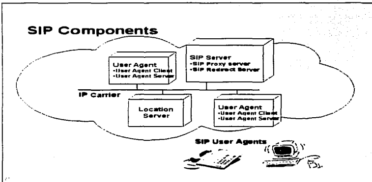
Figura III.54.- SIP Componentes.
