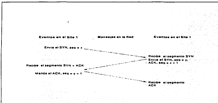
Figura II.26.- Conexión Orientada.
