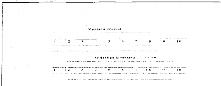
Figura II.21.- Ventanas Deslizantes.
