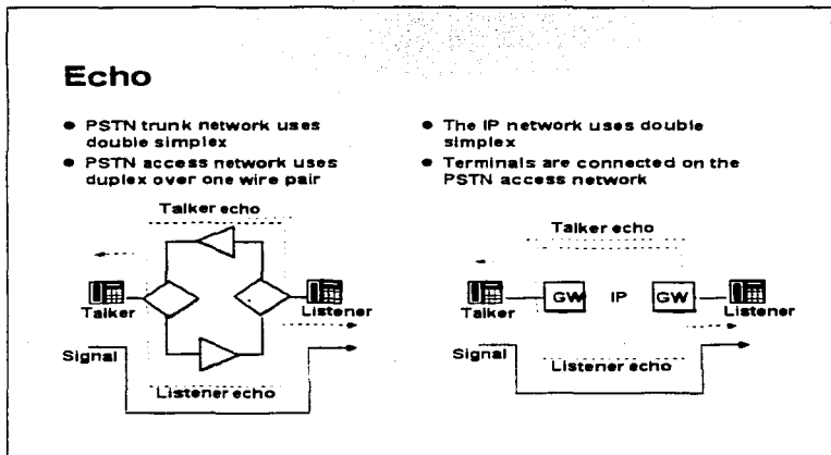
Figura III.40. ECHO.
