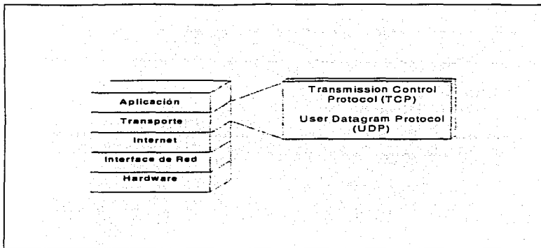
Figura II.18.- TCP.
