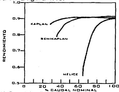
Figura 4.13: Curva de Rendimiento de las Turbinas Hélice, Semikaplan y Kaplan.
