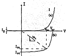
Figura 2.6: Características ideales de una celda solar.
