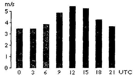
© 1998 www.WINDPOWER.org 3.11. Variaciones diurnas del viento
