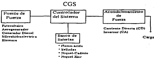
Figura 6.1. Diagrama de bloques de un sistema híbrido.
