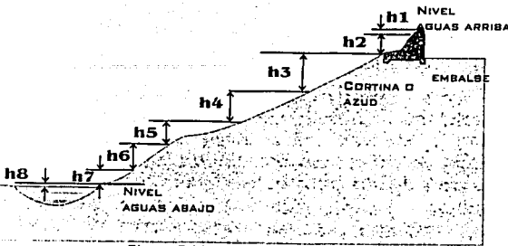
Figura 7.11: Método del Carpintero.
