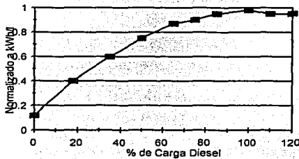
Figura 5.9. Consumo de combustible de un generador diesel de 30 kva. (Novel Wind/Diesel/Battery Hybrid Energy Sistem).
