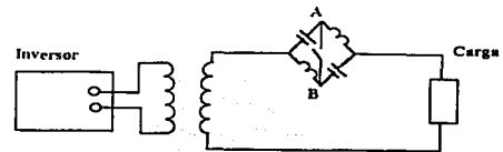
Figura 6.15. Limitación de corriente por resonancia.
