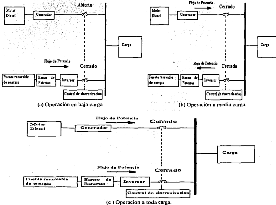
Figura 6.18. Operación del sistema híbrido en paralelo. (Novel Wind/Diesel/Battery Hybrid Energy System).
