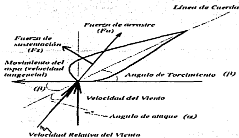
Figura 3.19. Diagrama Vectorial de un perfil aerodinámico.
