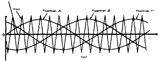
Figura 6.12. Formas de onda para un inversor PWM: ángulo del factor de potencia de la carga = $30^\circ$ de retraso. (Power Electronics: Converters, Applications and Design).
