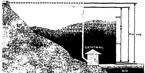
Figura 4.3 Esquema General de un Salto de Agua.
