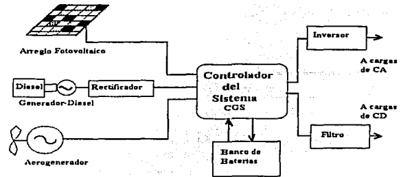
Figura 6.2. Sistema híbrido eólico-diesel-fotovoltaico.
