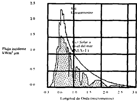
Figura 2.1. Espectro de radiación.
