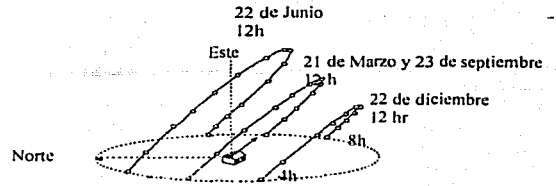
Figura 2.2. Trayectorias estacionales del sol a 40^\circ N de latitud.
