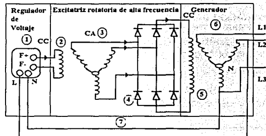
Figura 5.5. Diagrama esquemático del circuito eléctrico del generador de ca sin escobillas.
