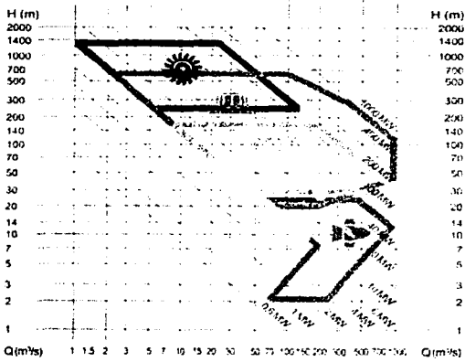
Figura 7.12: Diagrama de Selección de Turbinas.
