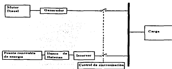
Figura 6.5. Sistema híbrido en paralelo. (Novel Wind/Diesel/Battery Hybrid Energy System).
