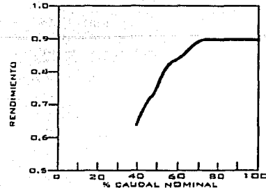
Figura 4.11: Curva de Rendimiento de la Turbina Francis.
