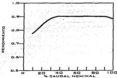
Figura 4.7: Curva de Rendimiento de la Turbina Pelton.
