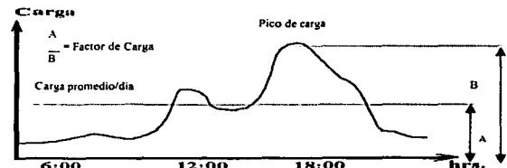
Figura 7.5: Factor de Carga F_c .
