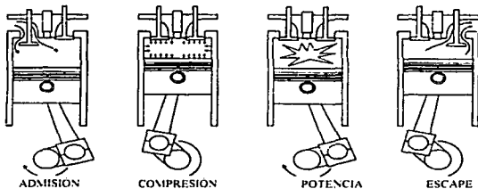
Figura 5.2. Conversión de energía química a energía mecánica. (Instituto Selmecc de Capacitación)
