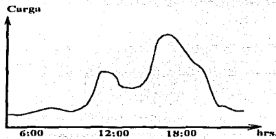
Figura 5.10. Perfil de carga típico de una comunidad rural. (Novel Wind/Diesel/Battery Hybrid Energy Sistem).
