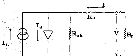
Figura 2.7 Circuito Equivalente de la Celda Solar.
