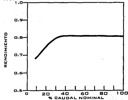
Figura 4.9: Curva de Rendimiento de la Turbina de Doble Impulsión.
