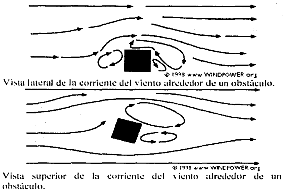
Figura 3.13. Obstáculos del viento.
