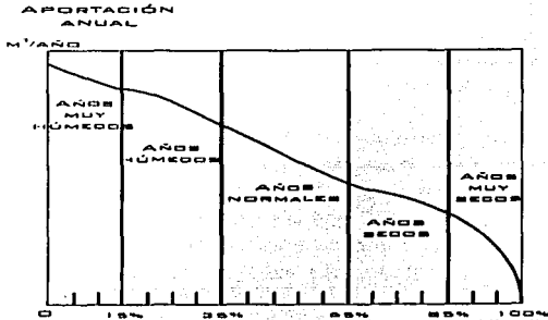
Figura 4.4: Frecuencia de Aparición Dentro de la Serie Anual Estudiada.
