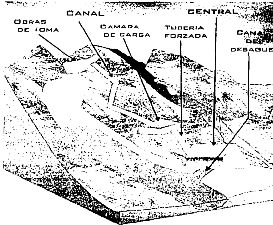
Figura 4.1 Esquema de una Central Hidroeléctrica de Tipo Fluyente.
