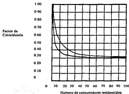
Figura 7.6: Límites de variación del factor de coincidencia para grupos diversos de consumidores residenciales.
