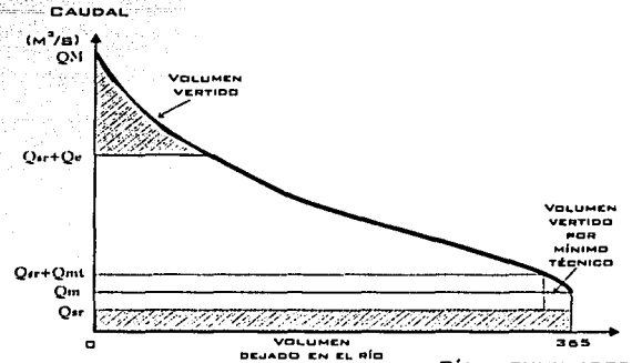
Figura 4.5: Construcción de una Curva de Caudales Clasificados.
