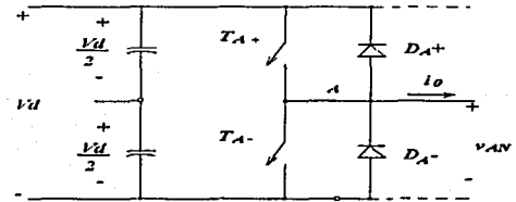
Figura 6.6. Inversor conmutado de una pierna. (Power Electronics: Converters, Applications and Design).
