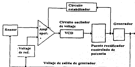
Figura 5.6. Diagrama de bloques del regulador de voltaje.
