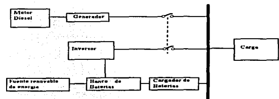
Figura 6.4. Sistema híbrido de alimentación alternada. (Novel Wind/Diesel/Battery Hybrid Energy System).
