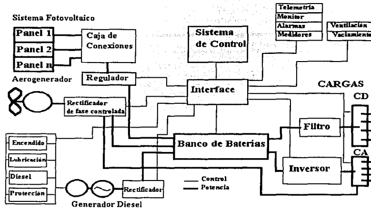
Figura 6.17. Sistema de control para el sistema híbrido. (Integrated Power Corporation).
