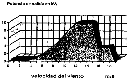
Figura 7.9 Curva de potencia de un aerogenerador
