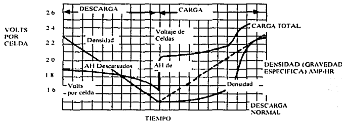
Figura 6.16. Características típicas de voltaje y densidad (gravedad), carga y descarga a régimen constante. (El Acumulador Eléctrico Tipo Plomo Ácido).
