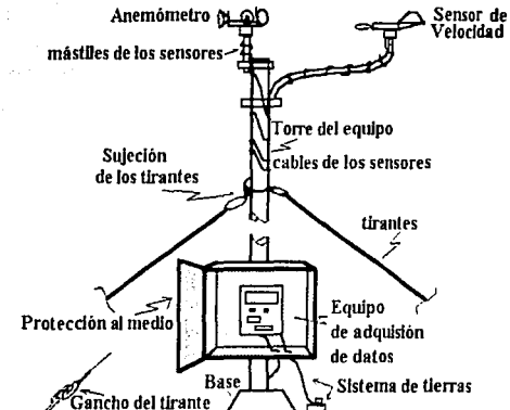
Figura 3.5: Instalación de un equipo de adquisición de datos. (NRG Logger).
