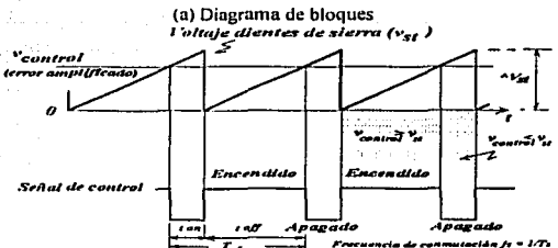
Figura 6.7. Diagrama de bloques de un modulador por ancho de pulsos (PWM). (Power Electronics: Converters, Applications and Design).
