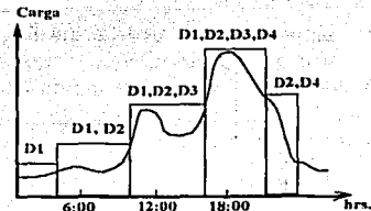
Perfil de la demanda diaria.
