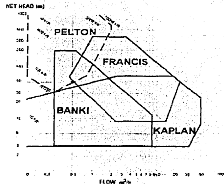
Figura 4.14: Campo de utilización de los diferentes tipos de turbinas.
