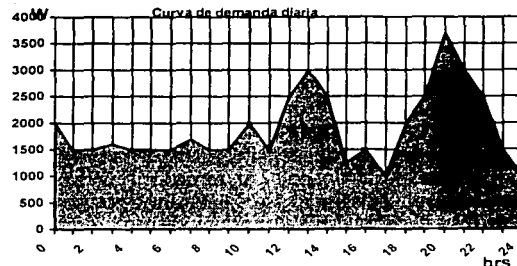
Figura 7.7 Curva de demanda diaria del Poblado de María Magdalena. (Westinghouse)
