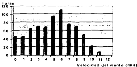
Figura 7.8 Histograma de velocidades de viento.
