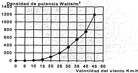
Figura 3.17: Ley del Cubo.
