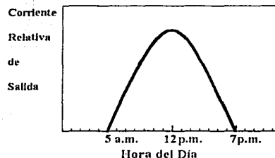
Figura 7.10: Corriente de salida de un sistema fotovoltaico en un día despejado.
