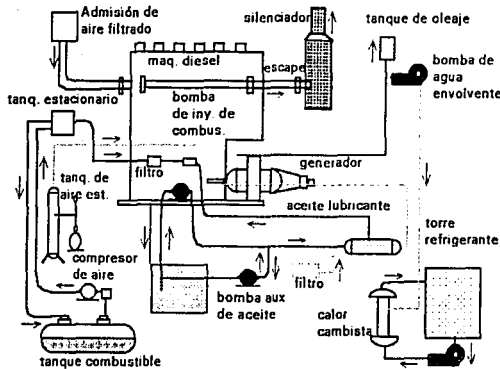
Figura 5.8. Elementos auxiliares de una planta generadora. (Instituto Selmecc de Capacitación).
