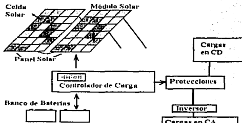
Figura 2.11: Configuración básica de un Sistema Fotovoltaico.
