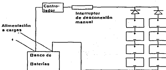
Figura 2.12: Conjunto Fotovoltaico con el uso de diodos de bloqueo.
