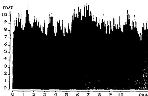
© 1998 www.WINDPOWER.org Figura 3.12. Turbulencia del Viento.
