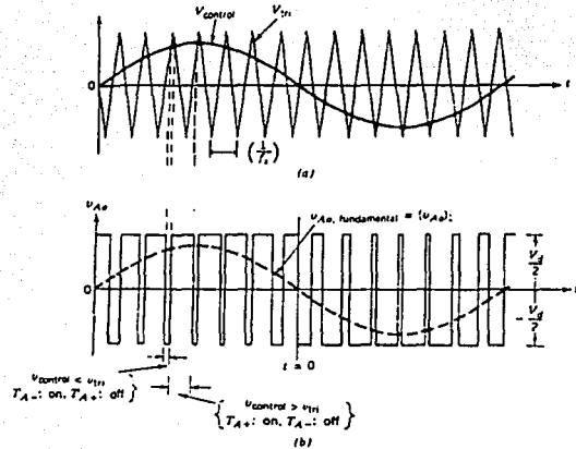
Figura 6.8. Modulación por ancho de pulso (PWM). (Power Electronics: Converters, Applications and Design).
