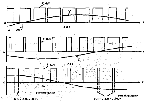
Figura 6.10. Formas de onda de un PWM trifásico. (Power Electronics: Converters, Applications and Design).
