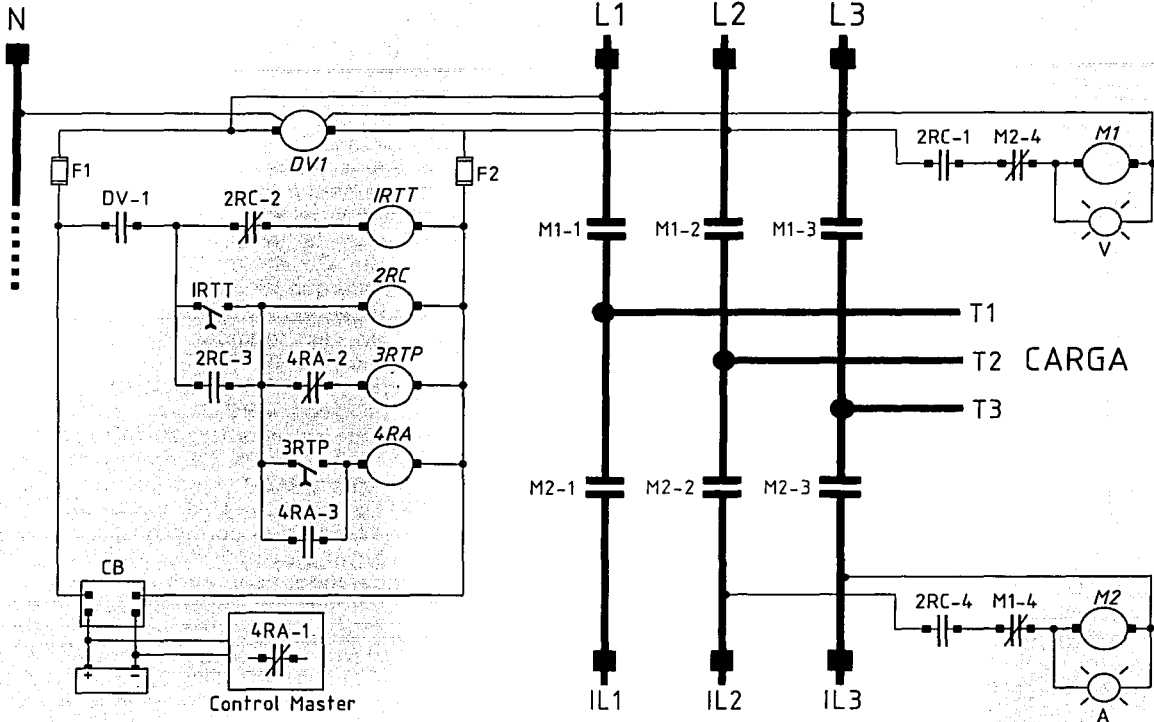
Figura 5.7. Diagrama elemental del circuito de control de transferencia y paro. (Instituto Selmecc de Capacitación).
