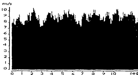
Figura 3.10. Variabilidad del Viento a Corto Plazo
