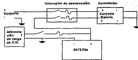
Figura 2.13: Protección a tierra.
