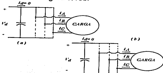
Figura 6.13. Estados de corto circuito para inversores PWM trifásicos. (Power Electronics: Converters, Applications and Design).
