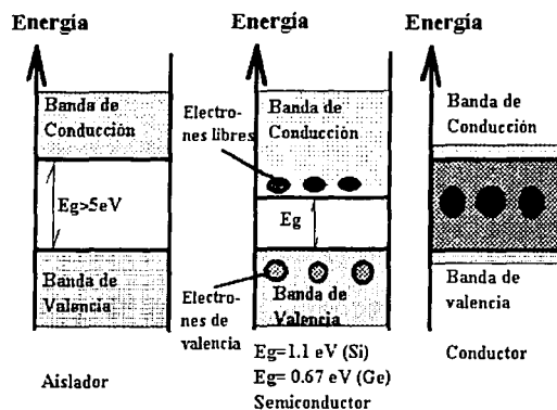
Figura 2.4: Bandas de valencia.
