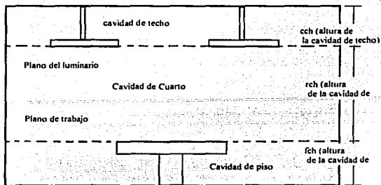
Figura 7.3: Método de cavidad zonal.
