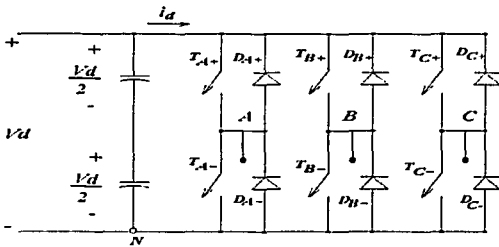
Figura 6.9. Inversor trifásico
