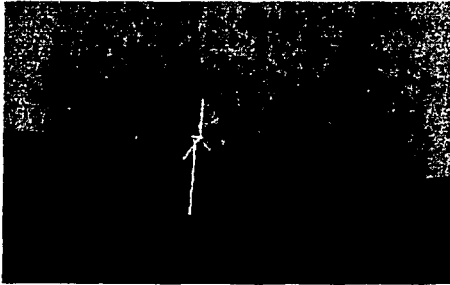
Figura 3.15.- Efecto Túnel
