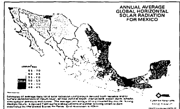
Figura 2.14: Mapa de Insolación solar.
