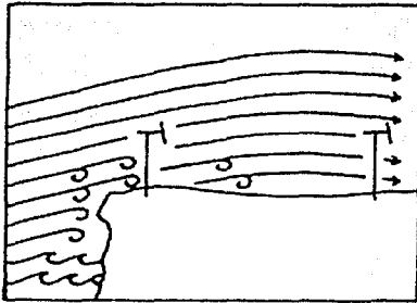
Figura 3.9. Escarpas
