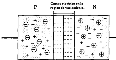
Figura 2.5. Unión p-n sin polarización externa
