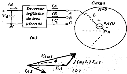
Figura 6.11. Inversor trifásico: (a) Diagrama del circuito, (b) Diagrama fasorial (de la frecuencia fundamental).
