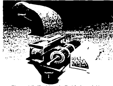
Figura 4.8: Turbina de Doble Impulsión.
