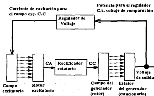
Figura 5.4. Diagrama de bloques para el sistema de generación.
