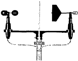
Figura 3.3: Sensores de medición de viento, Wind Speed and Directions Sensors, Campbell Scientific.
