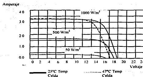
Figura 2.10: Características de módulos solares.
