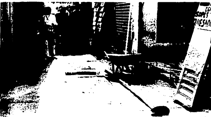
Colado de techo (planta baja) de la Casa de la Cultura, 60% de avance en obra negra.
