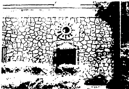
IMPERMEABILIZACION DE LA BIBLIOTECA DE STA. MARIA CUEVAS 184 M2. DE IMPERMEABILIZACION, CON RECURSOS CODEM.
