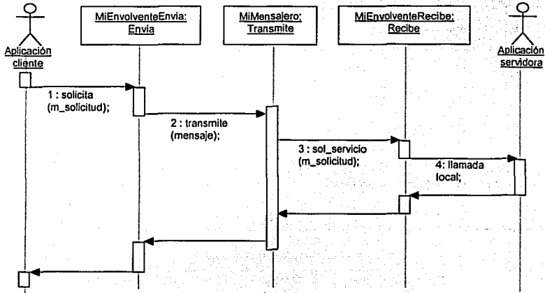
Figura 4.20. Diagrama de secuencia "Solicitud - respuesta".
