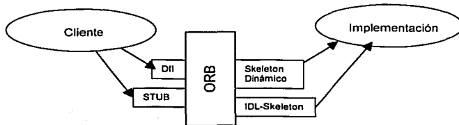
Figura 2.16. Interfaces estática y dinámica.
