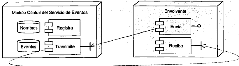
Figura 5.7. Diagrama general de componentes.
