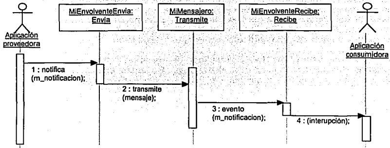
Figura 4.23. Diagrama de secuencia "Respuesta".
