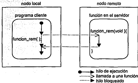
Figura 2.5. Llamada a una función remota.
