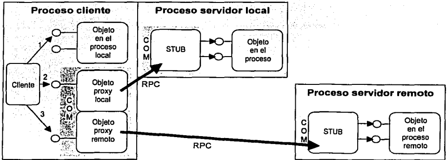
Figura 2.11. Arquitectura de COM - DCOM.
