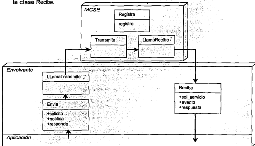
Figura 4.18. Diagrama de clases.
