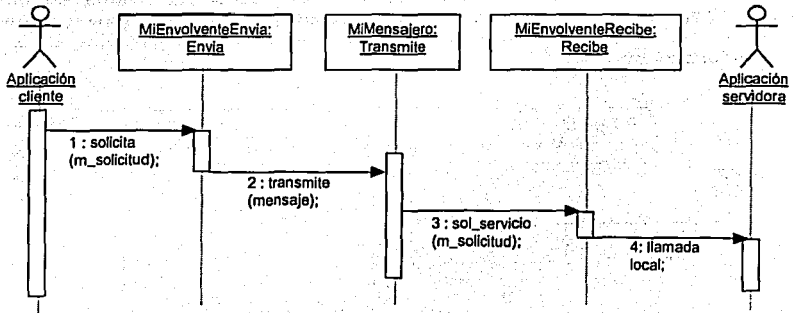
Figura 4.21. Diagrama de secuencia "Solicitud".
