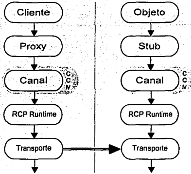
Figura 2.12. Flujo de comunicación entre un cliente y un servidor.
