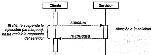
Figura 1.7. Solicitud - respuesta.
