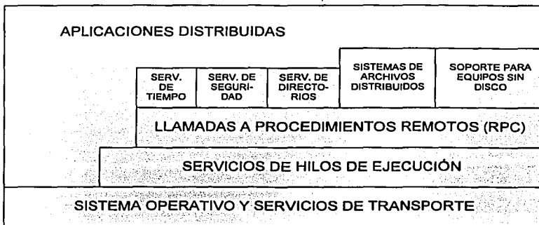
Figura 2.8. Arquitectura de DCE.
