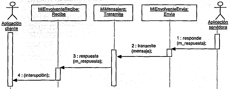
Figura 4.22. Diagrama de secuencia "Respuesta".
