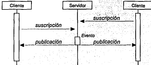
Figura 1.10. Publicación - suscripción.
