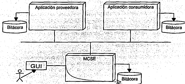
Figura 5.11. Archivos bitácora.
