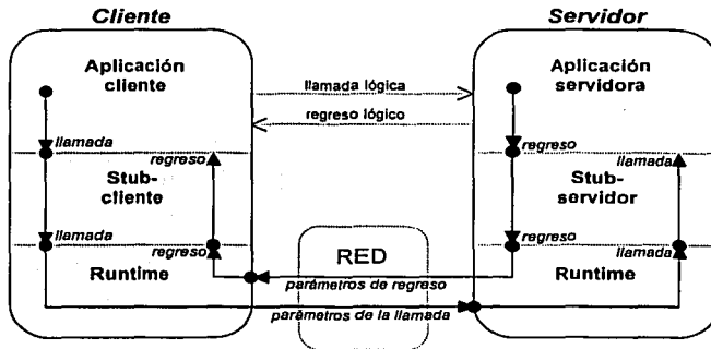
Figura 2.6. Modelo RPC.
