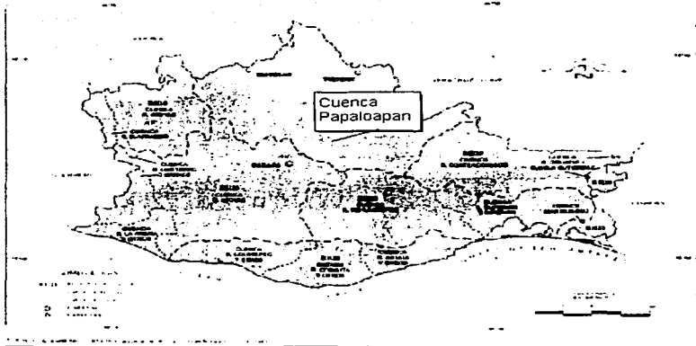
MAPA 5 CUENCAS HIDROLÓGICAS
