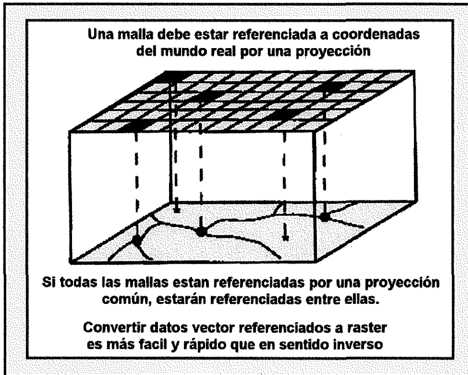
Figura 1.12 Esquema de conversión de datos vector-raster
