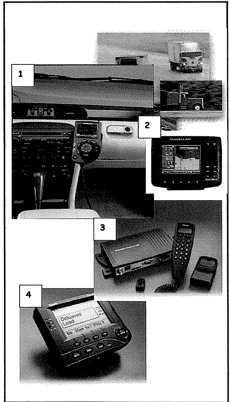
Figura 1. 44 Equipos con base en GPS para: 1 y 2 .sistema de información al conductor (Magellan 750Nav y Magellan Nav6510); localización y monitoreo de vehículos y para sistema inteligentes de transporte (3. Trimble CrossCheck y 4. terminal Echo RTX) Fuente:www.MagellanGPS.com y www.trimble.com/transportation
