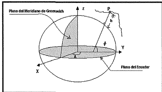
Figura 1.43 Transformación de coordenadas cartesianas en geodésicas.
