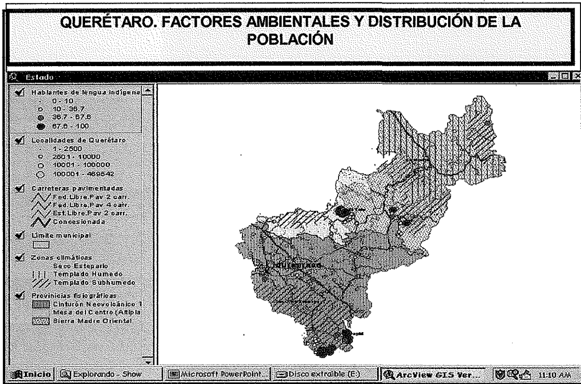
Figura 3.27 Provincias fisiográficas, zonas climáticas y distribución de la población en Querétaro. Fuente: INEGI, Síntesis geográfica de Qro. y Censo de Población 1995.
