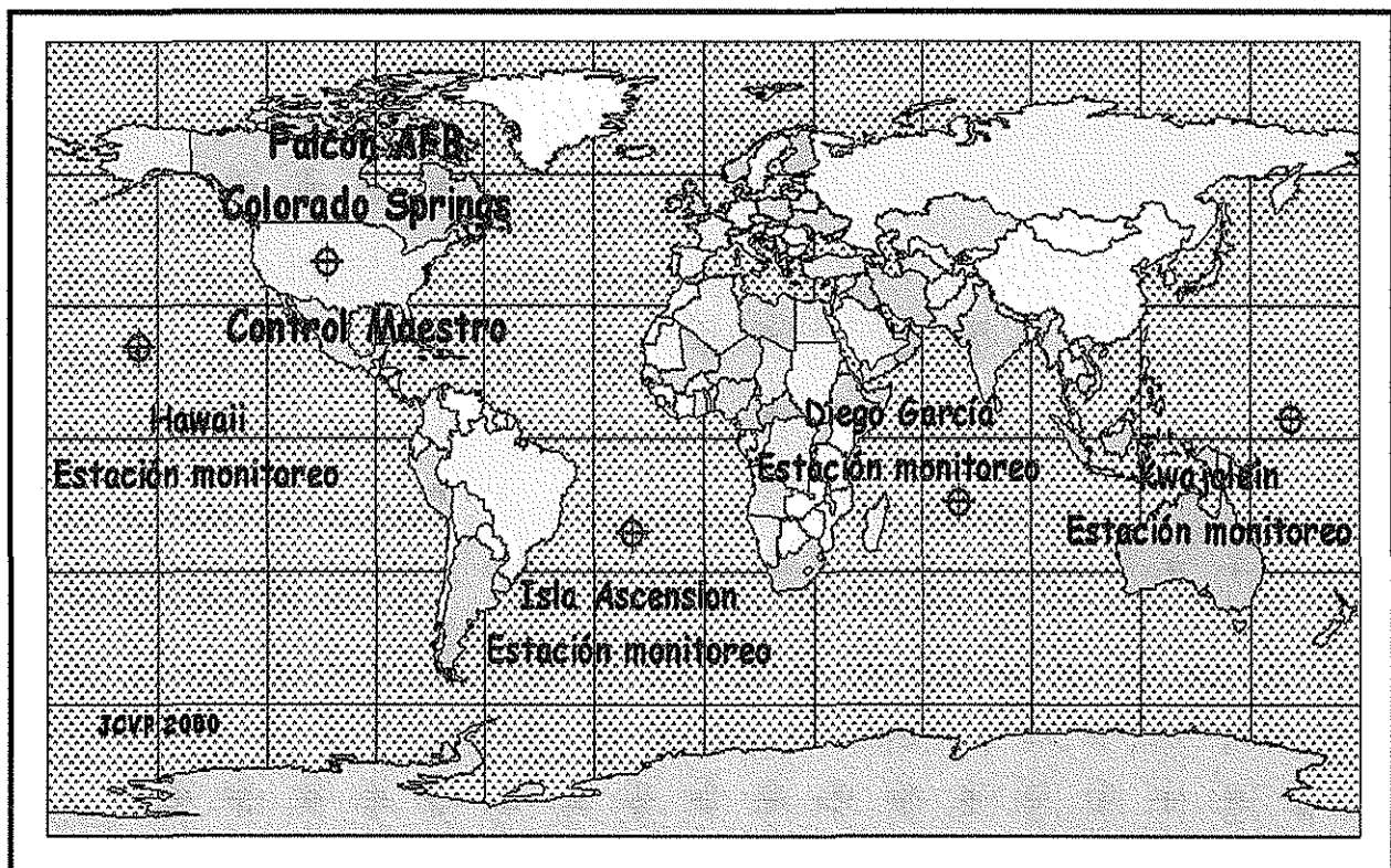
Figura 140 Control Maestro y red de estaciones de monitoreo GPS Fuente: Elaboración propia con base en Dana, P. op. cit.
