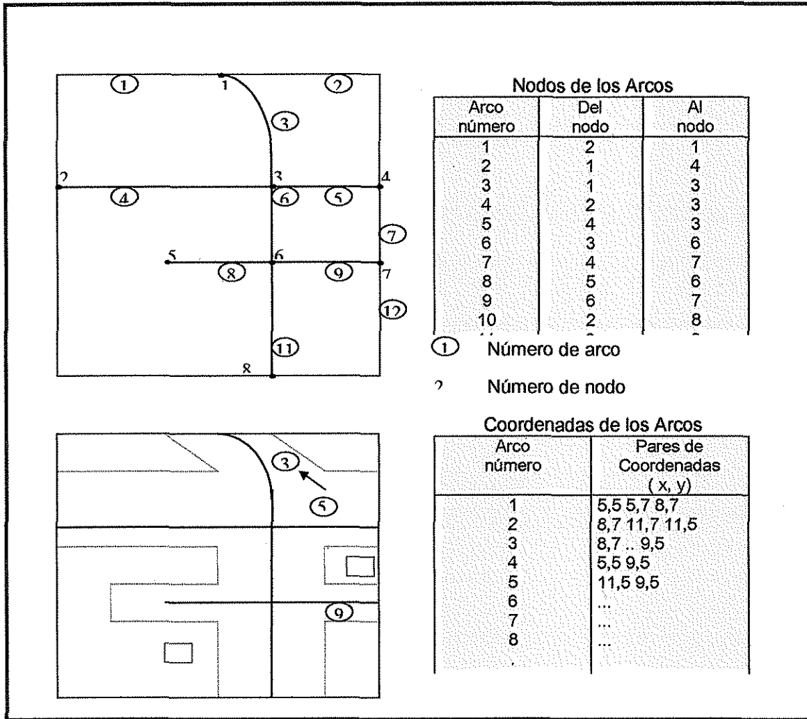
Figura 1.25 Conectividad . Esquema diagramático de la conexión topológica de arcos y nodos Fuente: ESRI. Understanding GIS. The ArcInfo Method, 1997
