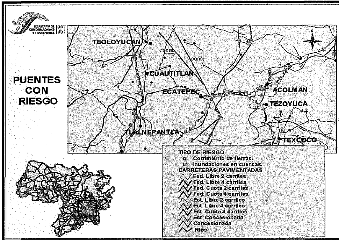
Figura 3.8 Puentes con riesgo de corrimiento de tierras o inundación en la zona de estudio Fuente: Instituto Nacional de Ecología, Semarnat. México, 2000.
