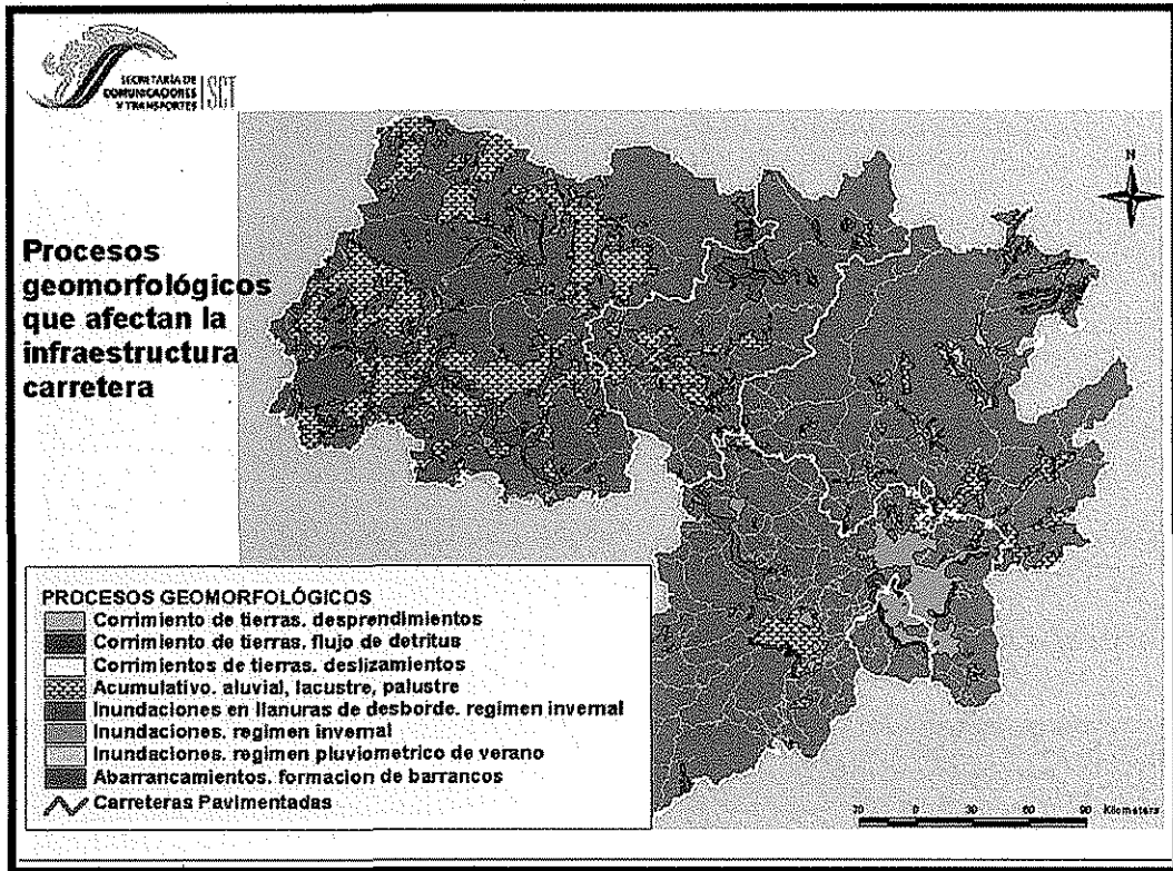
Figura 3.6 Procesos geomorfológicos que afectan la red carretera en la zona de estudio Fuente: Instituto Nacional de Ecología, Semarnat, México, 2000.
