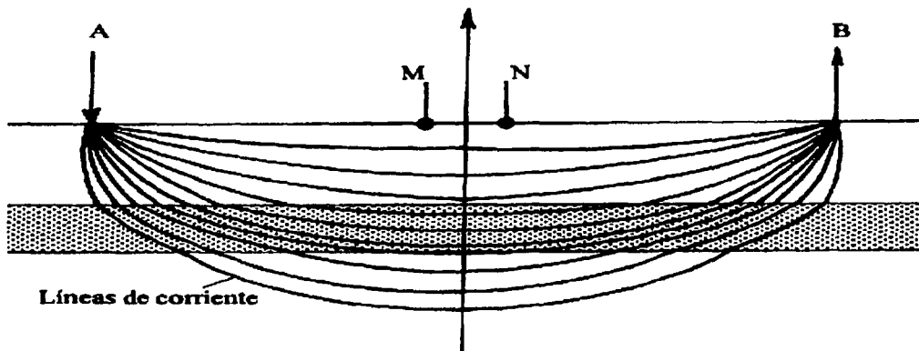
Figura 5.3. Diagrama del método de Schlumberger para medir resistividad. A y B: electrodos de inyección de corriente. M y N: electrodos de medición de potencial eléctrico producido por la corriente inyectada.
