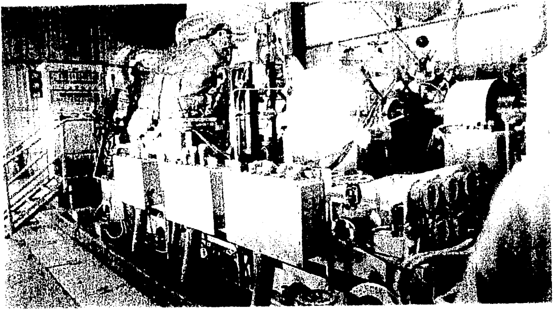
CASA DE MÁQUINAS DE UNA PLANTA DE GENERACIÓN DE 25 MW, LOS AZUFRES, MICH.
