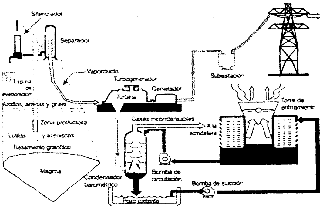
Figura 5.2. Geotermoeléctrica que a continuación se describe detalladamente.
