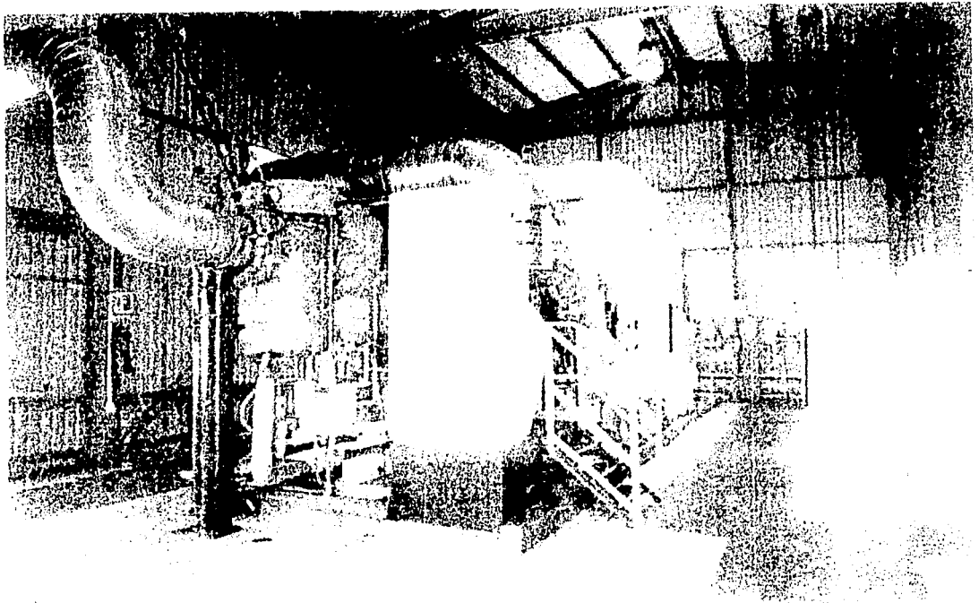
CASA DE MÁQUINAS DE UNA PLANTA DE GENERACIÓN DE 25 MW, LOS AZUFRES, MICH.
