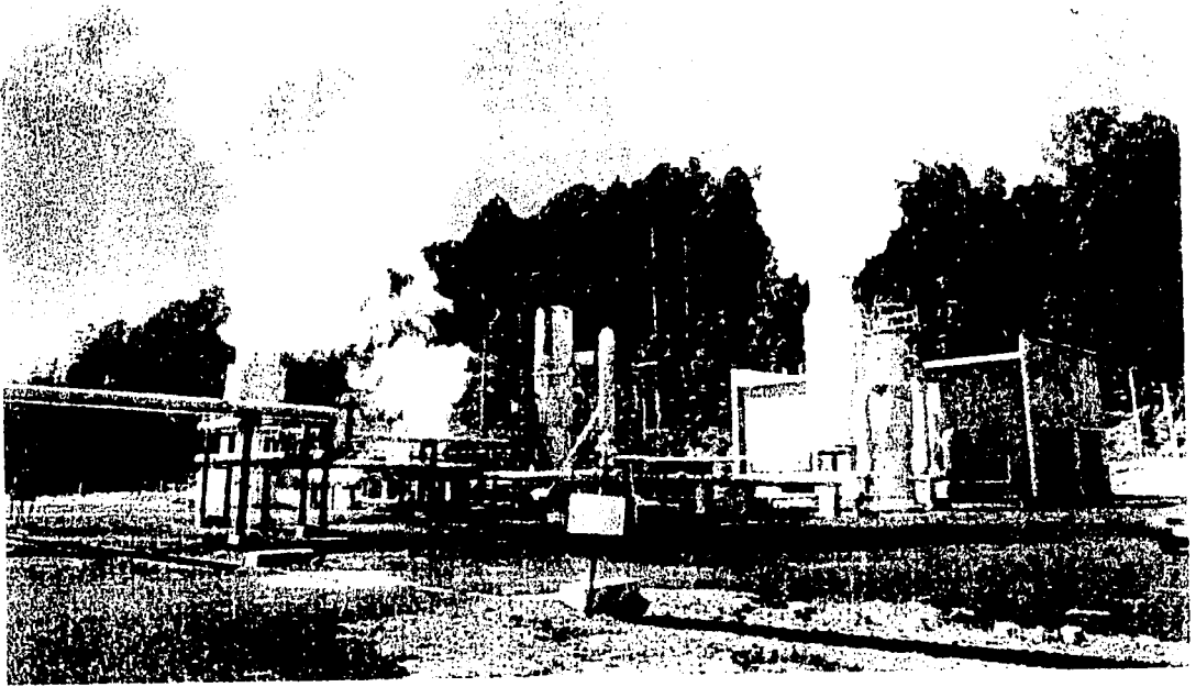
VISTA EXTERIOR DE UNA PLANTA DE GENERACIÓN DE 25 MW, LOS AZUFRES, MICH.
