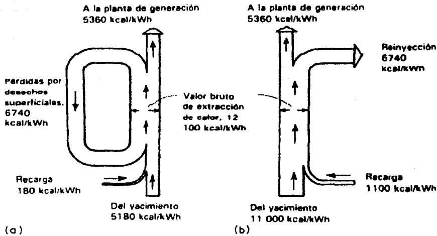
Figura 10.1. Balances de energía del yacimiento para un campo de agua dominante, estimado para Ahuachapán, El Salvador. De a cuerdo con la figura a) Vaporización de una etapa con reinyección; b) Vaporización de una etapa con desecho superficial de fluido.
