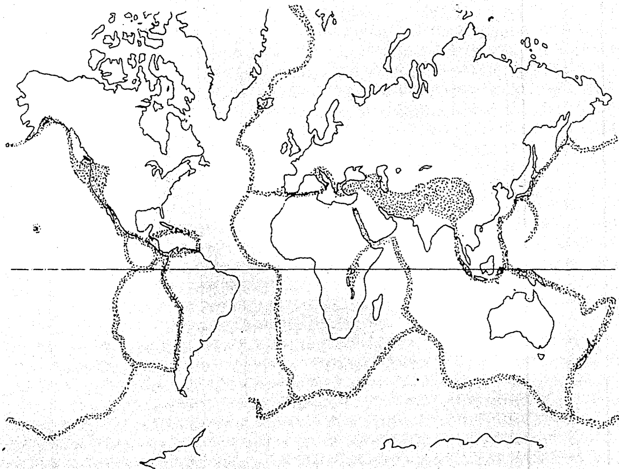
Figura I.3 Zonas principales de terremotos del mundo. (Tomado del mapa de World Seismicity, 1961-9, publicado por el National Earthquake Centre, Washington D.C.)
