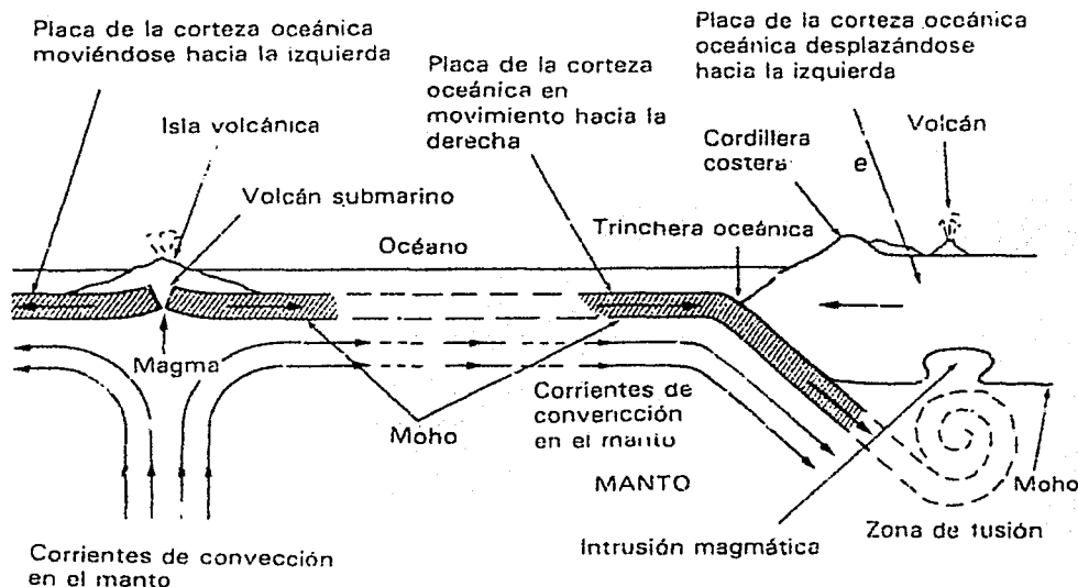
Figura 1.4 Movimientos de las placas de la corteza (no están a escala)
