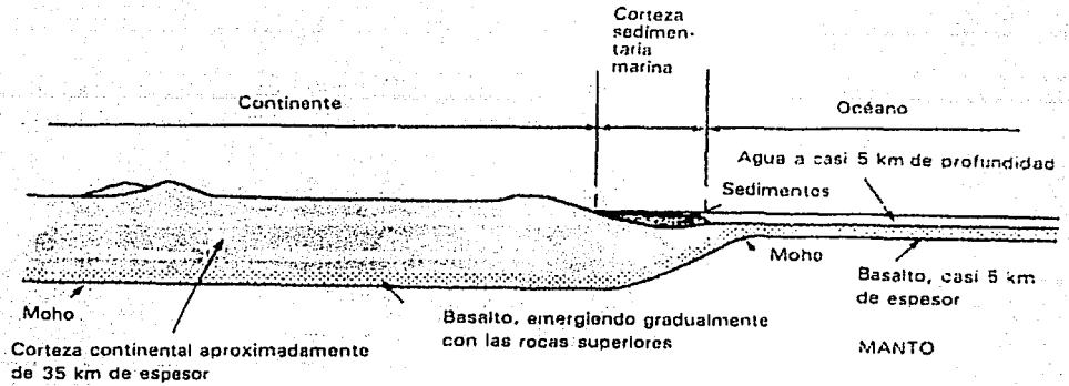
Figura 1.2 Sección esquemática de la corteza terrestre en un litoral inactivo (por ejemplo, el litoral oriental de América del Norte).
