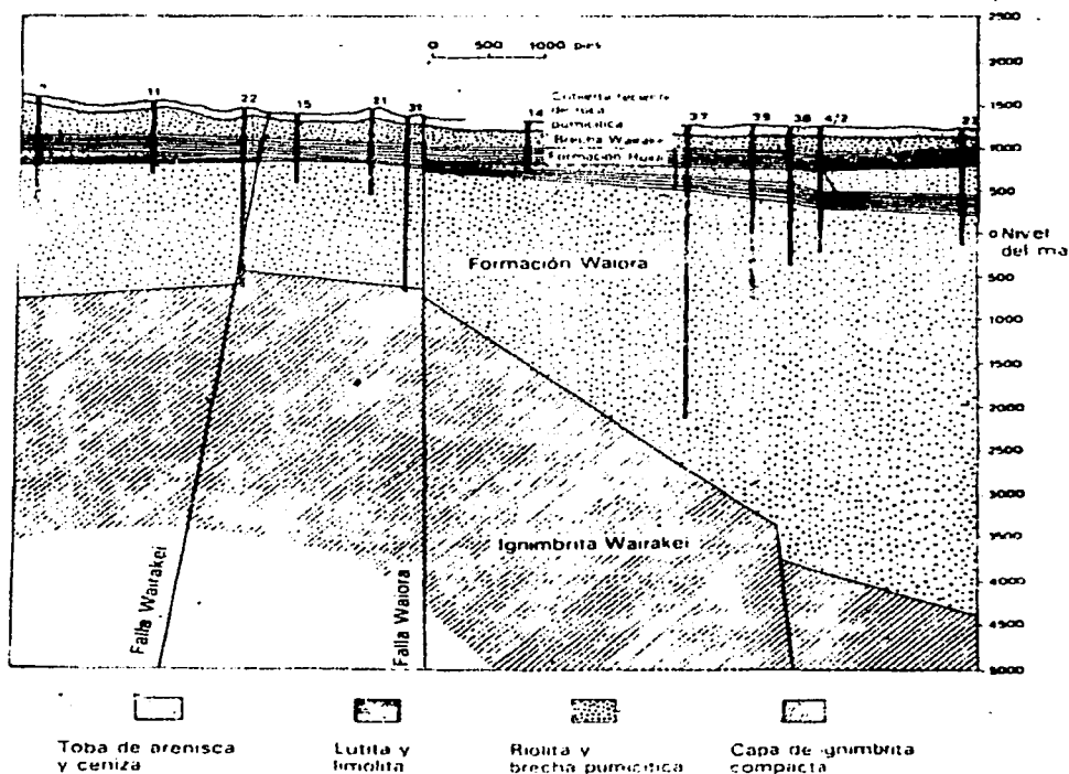
Figura 5.1. Corte geológico del campo termal de Wairakei. Nueva Zelanda.
