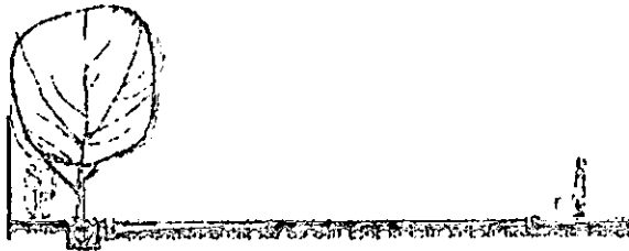
Sección Vial de Avenida Juárez (inicio de calle peatonal)
