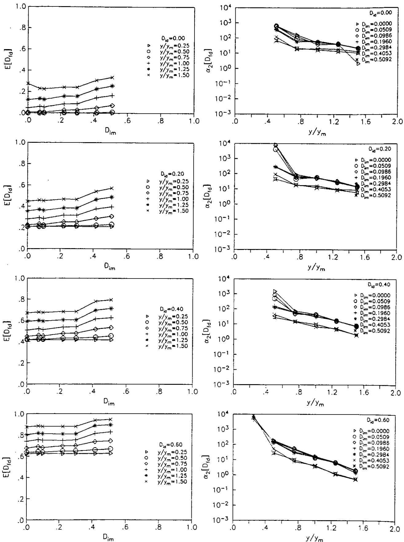
Fig. 6.52 Daño medio en dissipador de marco equivalente con \eta_k=\tau_R=0.5 , T=1.5 s, c_s=0.4 para diferentes intensidades normalizadas de los sismos ( y/y_m ).
