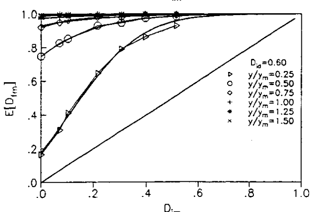
Fig. 6.57 Daño medio en marco equivalente con \eta_k = \tau_R = 0.75 , T = 1.5s , c_s = 0.4 para diferentes intensidades normalizadas de los sismos ( y/y_m ) y sus curvas ajustadas.
