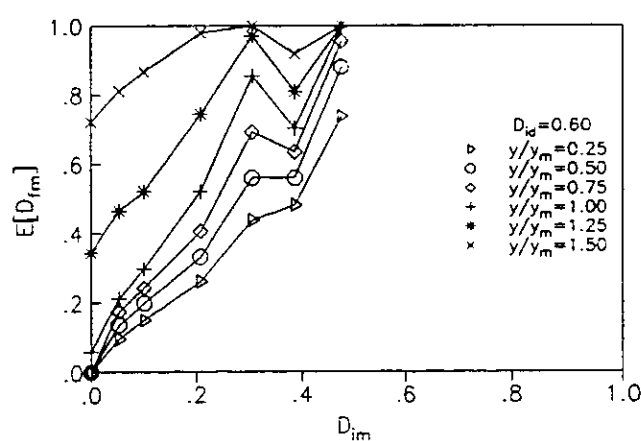
Fig. 6.29 Daño medio en marco equivalente con \eta_k = \eta_R = 0.5 , T = 0.5 s, c_s = 0.6 para diferentes intensidades normalizadas de los sismos ( y/y_m ).
