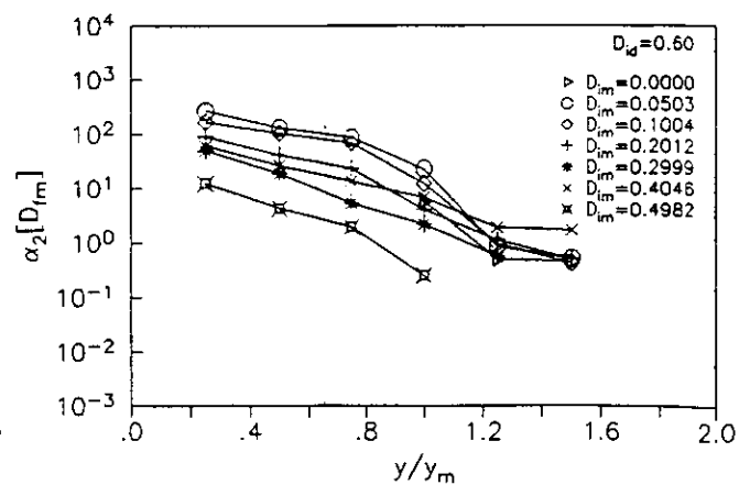
Fig. 6.29 Daño medio en marco equivalente con \eta_k = \eta_R = 0.5 , T = 0.5 s, c_s = 0.6 para diferentes intensidades normalizadas de los sismos ( y/y_m ).
