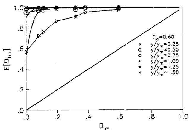
Fig. 6.55 Daño medio en marco equivalente con r_k=r_R=0.75 , T=1.5 s, c_s=0.2 para diferentes intensidades normalizadas de los sismos ( y/y_m ) y sus curvas ajustadas.
