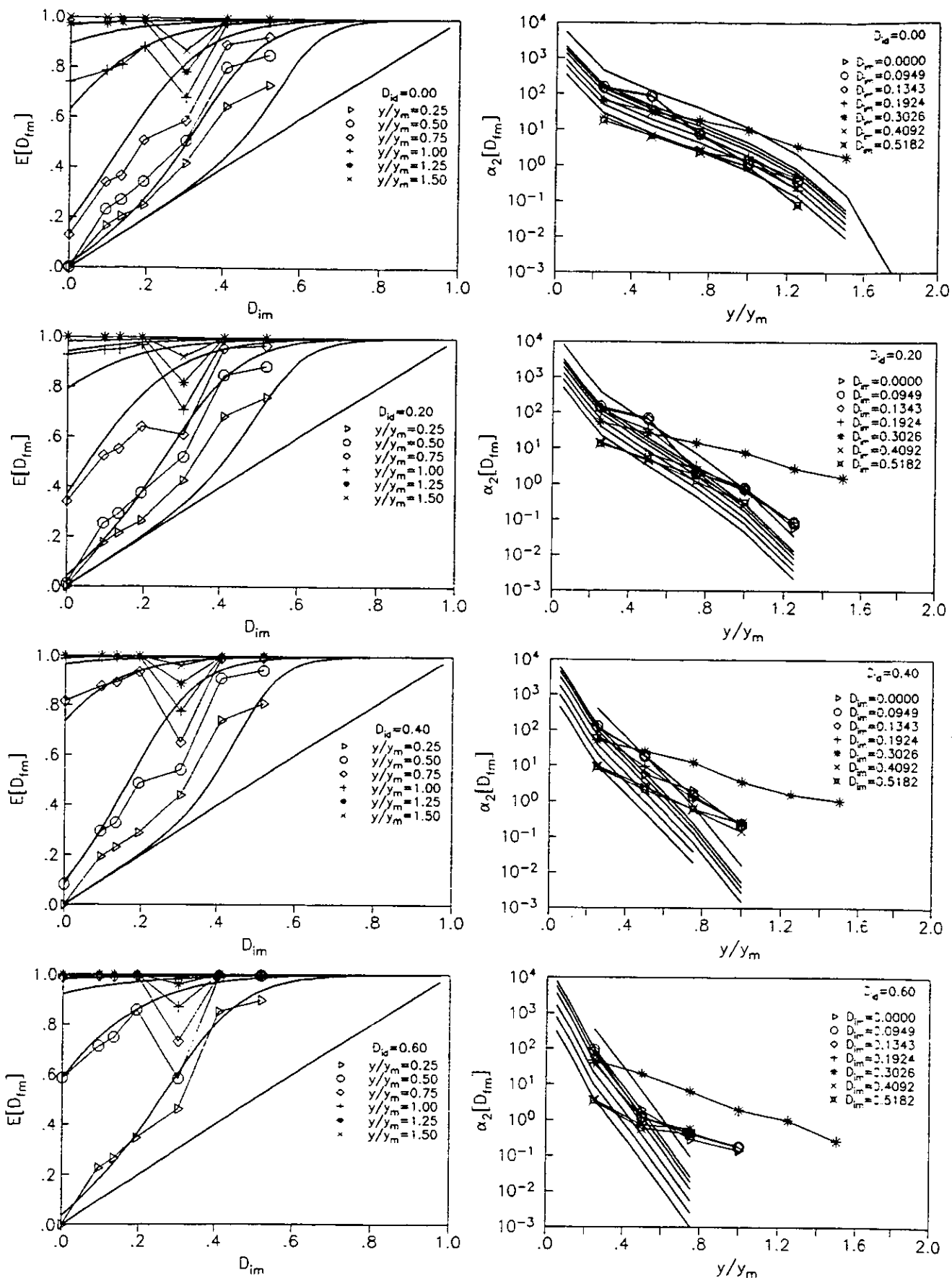
Fig. 6.43 Daño medio en marco equivalente con r_k=r_R=0.75 , T=1.0 s, c_s=0.2 para diferentes intensidades normalizadas de los sismos ( y/y_m ) y sus curvas ajustadas.
