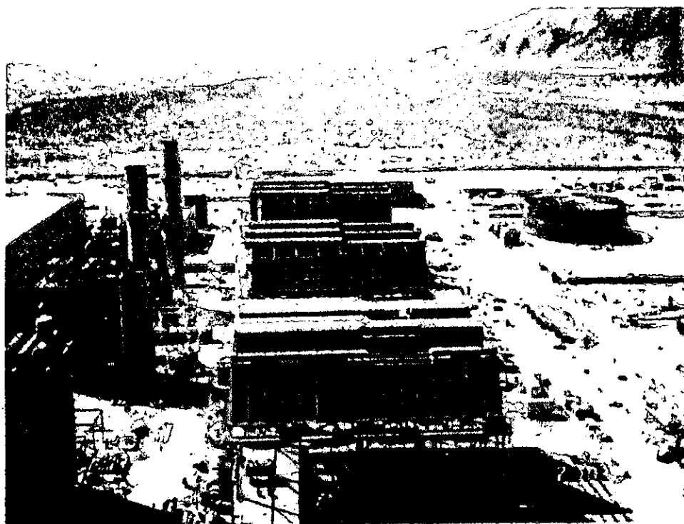
VISTA SUPERIOR DE LOS AEROCONDENSADORES
