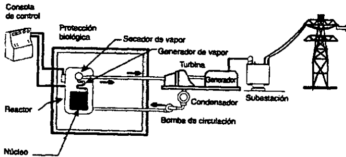
Diagrama esquemático de una central nucleoelectrónica tipo BWR
