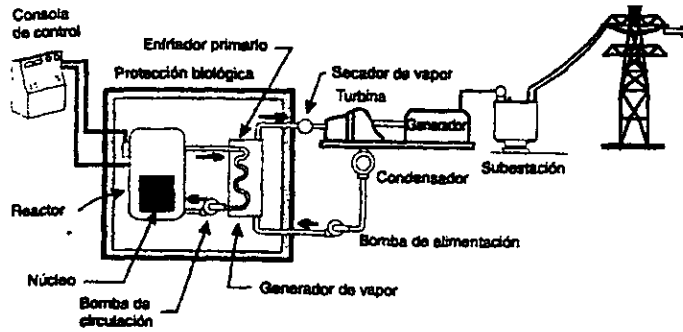
Diagrama esquemático de una central nucleoelectrónica tipo PWR
