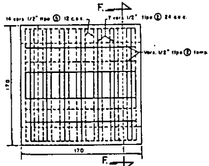
LOSA INFERIOR
