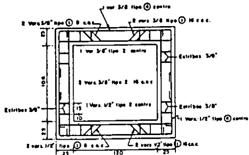
MARCOS AyB
