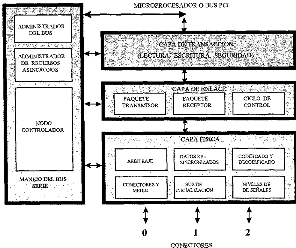
FIGURA 2.1.- DIAGRAMA BASICO DE LAS CAPAS QUE COMPONEN EL FIREWIRE.
