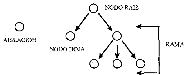
FIGURA 3.1.- TOPOLOGIA DEL SISTEMA FIREWIRE.
