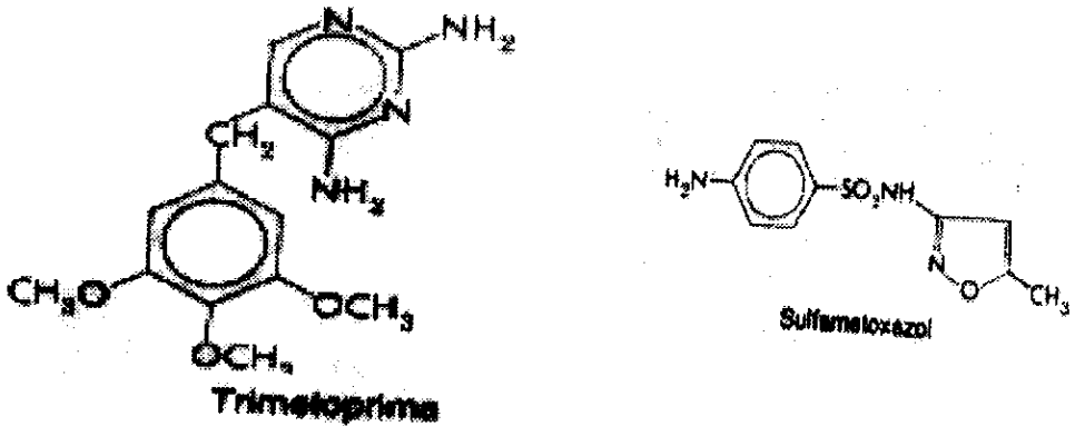
Figura 10. Estructura química del Trimetoprim y Sulfametoxazol.
