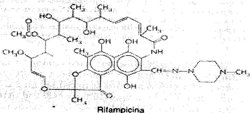
Figura 9. Estructura química de la Rifampicina.
