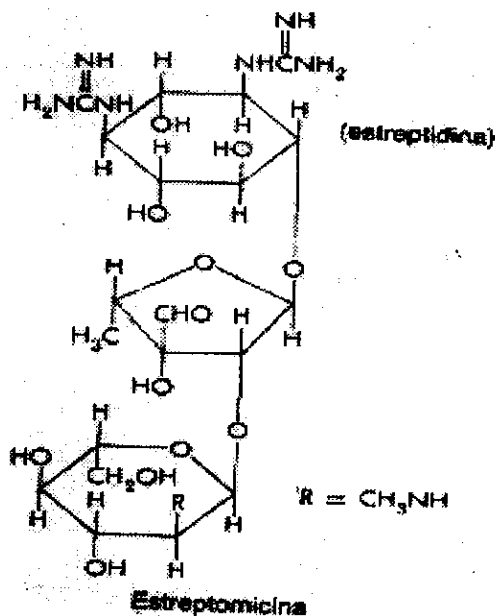
Figura 8. Estructura química de la Estreptomina.
