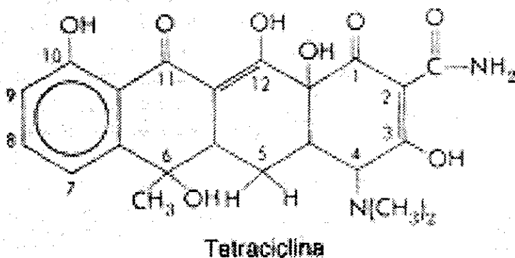
Figura 7. Estructura química de la Tetraciclina.
