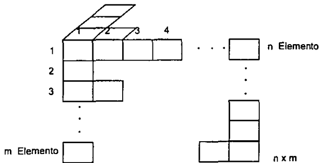
FIG. 2.25. Espacio n-dimensional.
