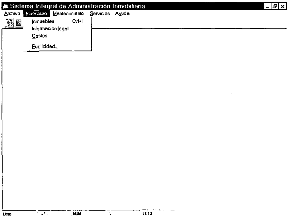
FIG. 8.6 Menú Inventario.
