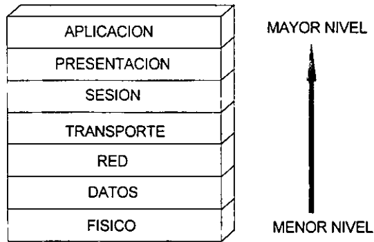
FIG. 2.32. Modelo OSI.
