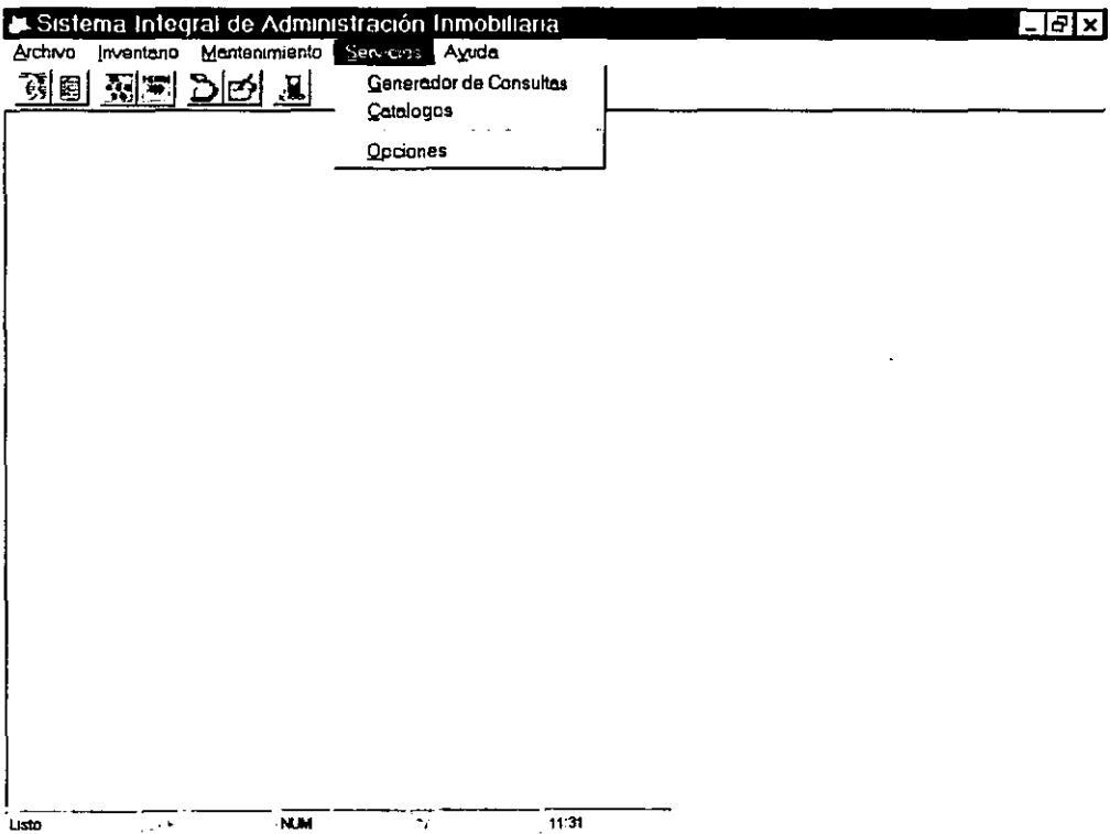
FIG. 8.8 Menú Servicios.
