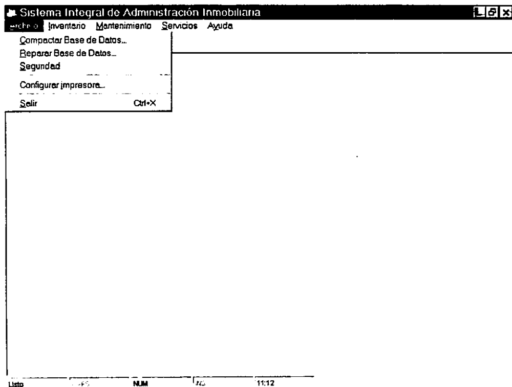
FIG. 8.5 Menú Archivo.
