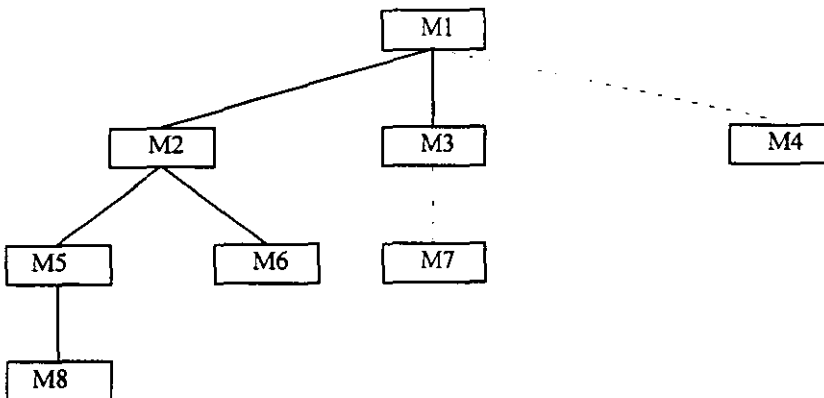
FIG. 2.42. Integración descendente.
