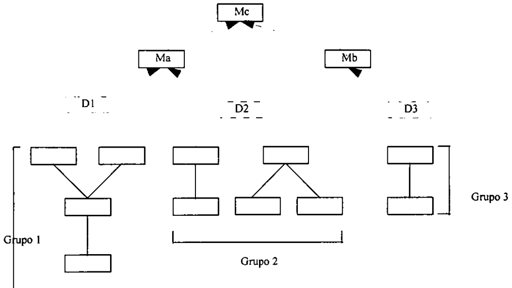
FIG. 2.43. Integración ascendente.
