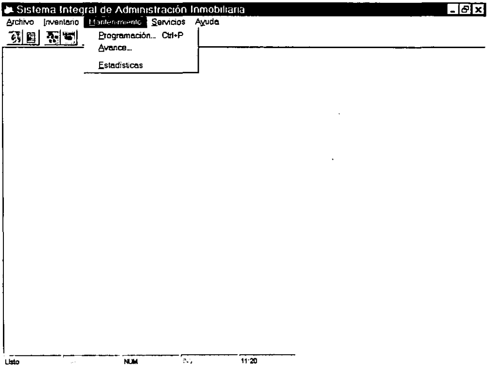
FIG. 8.7 Menú Mantenimiento.
