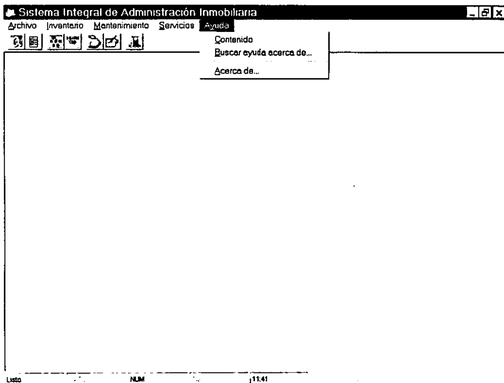
FIG. 8.9 Menú Ayuda.
