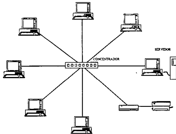
FIG. 2.28. Topología de Estrella.
