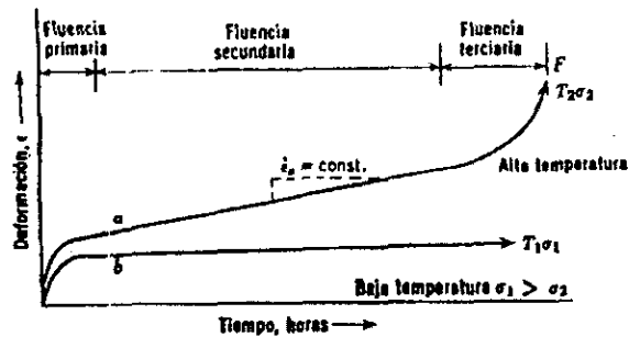
FIGURA 3.3.2 (a) las tres etapas de una relación entre la deformación y el tiempo, para fluencia a temperaturas elevadas; (b) la misma relación a baja temperatura
