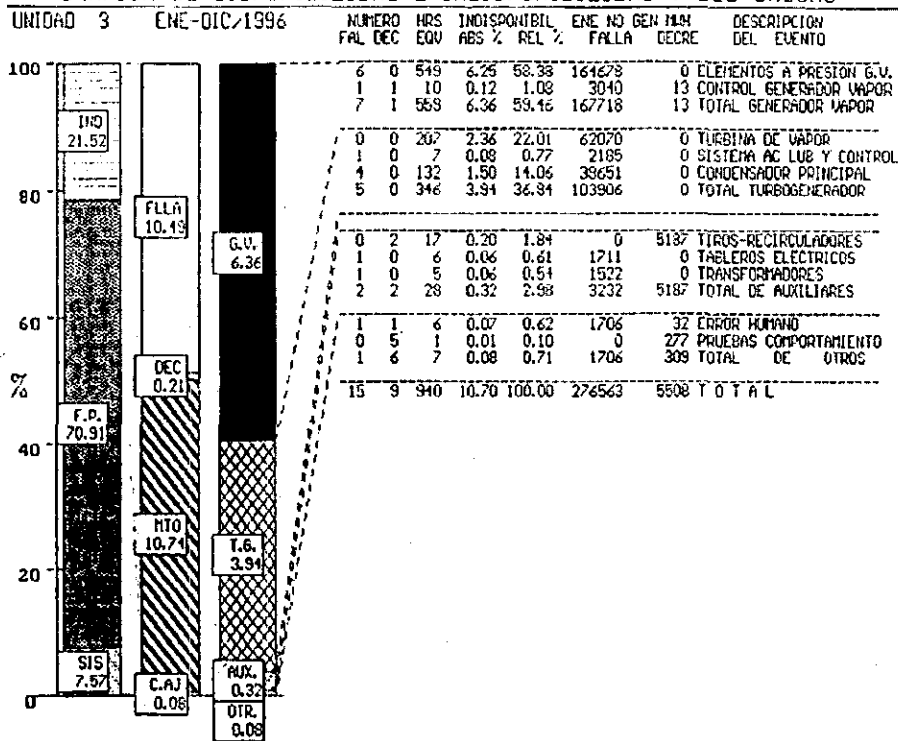
Figura V.5 Disponibilidad e Indisponibilidad de U-3 en 1996
