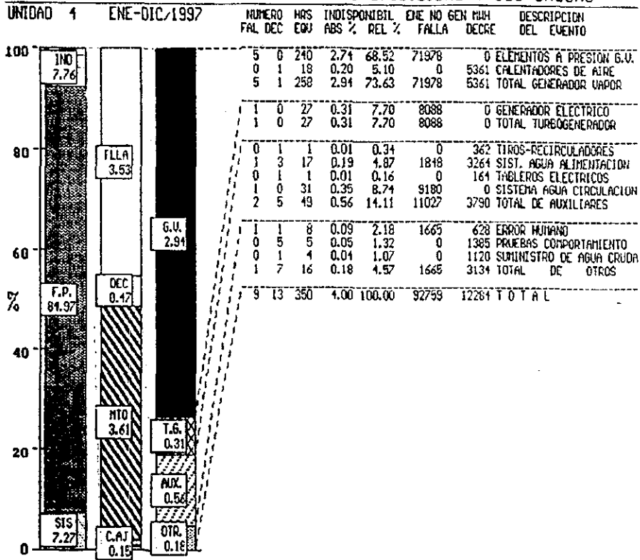
Figura V.11 Disponibilidad e indisponibilidad de U-4 en 1997
