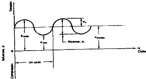
Fig. III.2 Esfuerzos cíclicos repetidos
