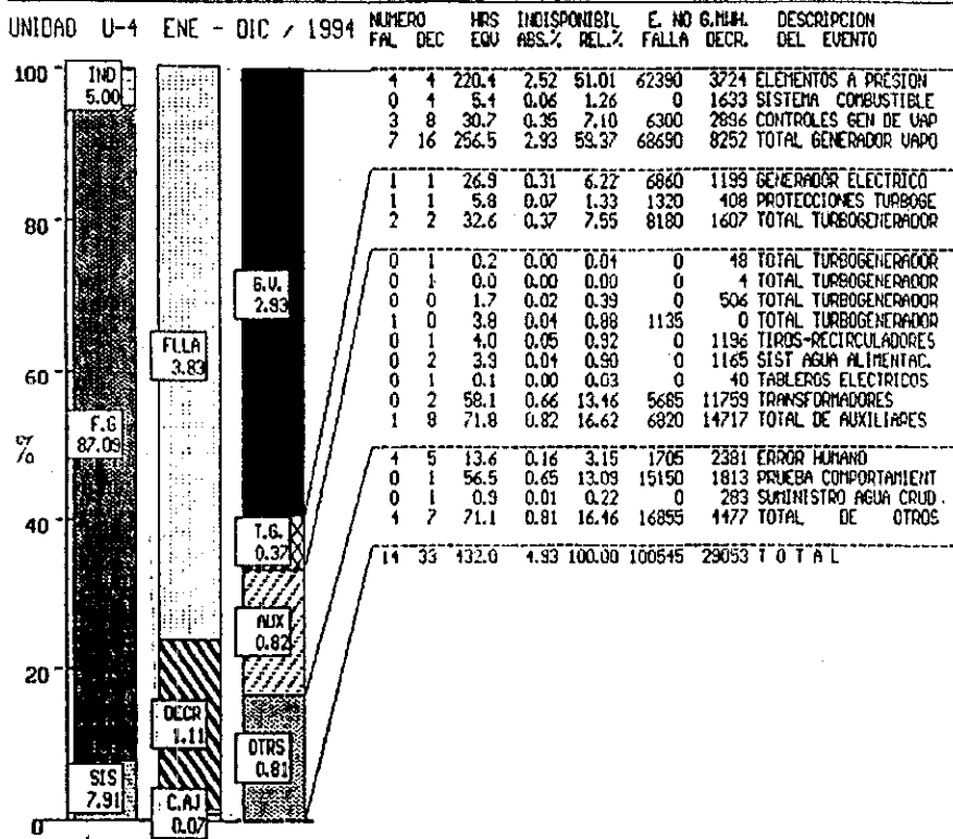
Figura V.8 Disponibilidad e Indisponibilidad de U-4 en 1994
