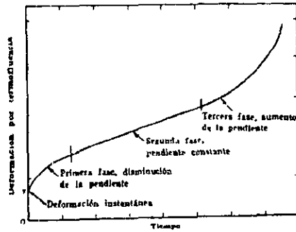
Fig. .III.7 las tres fases de la curva de Termofluencia.
