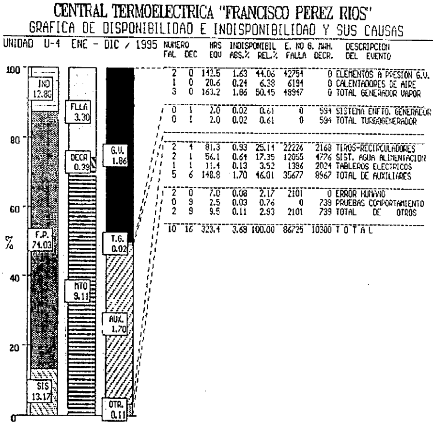
Figura V.2-9 Disponibilidad e indisponibilidad de U-4 en 1995
