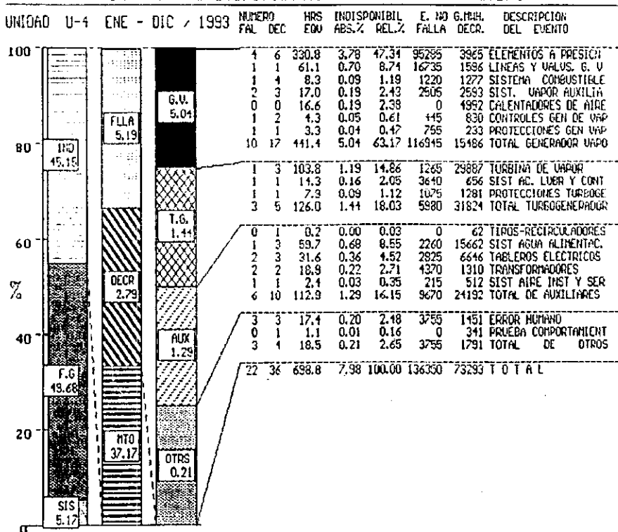
Figura V.7 Disponibilidad e Indisponibilidad de U-4 en 1993
