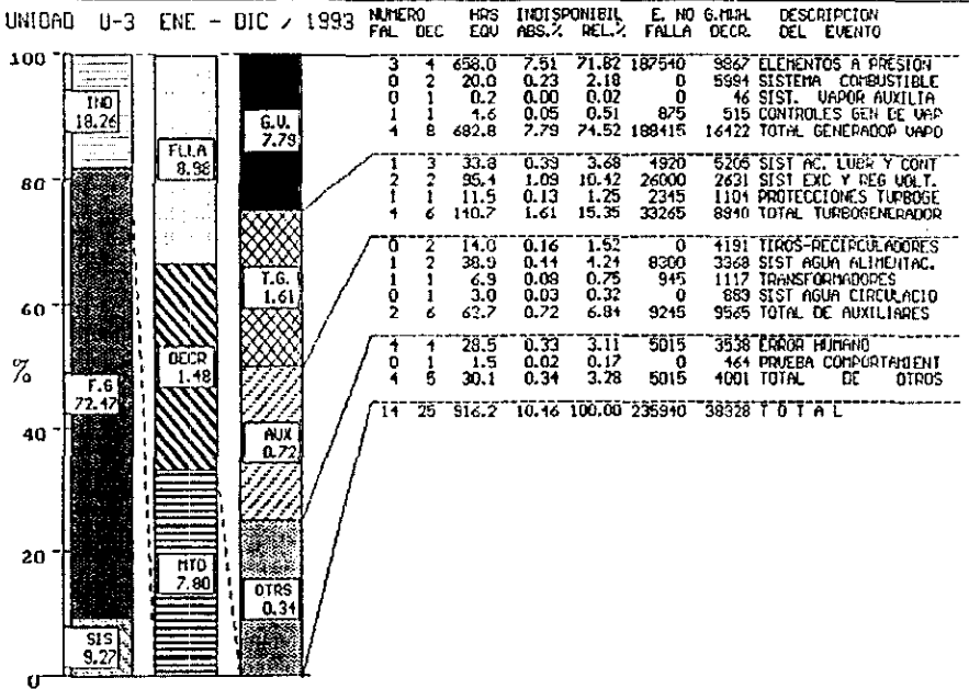
Figura V.2 Disponibilidad e Indisponibilidad de U-3 en 1993
