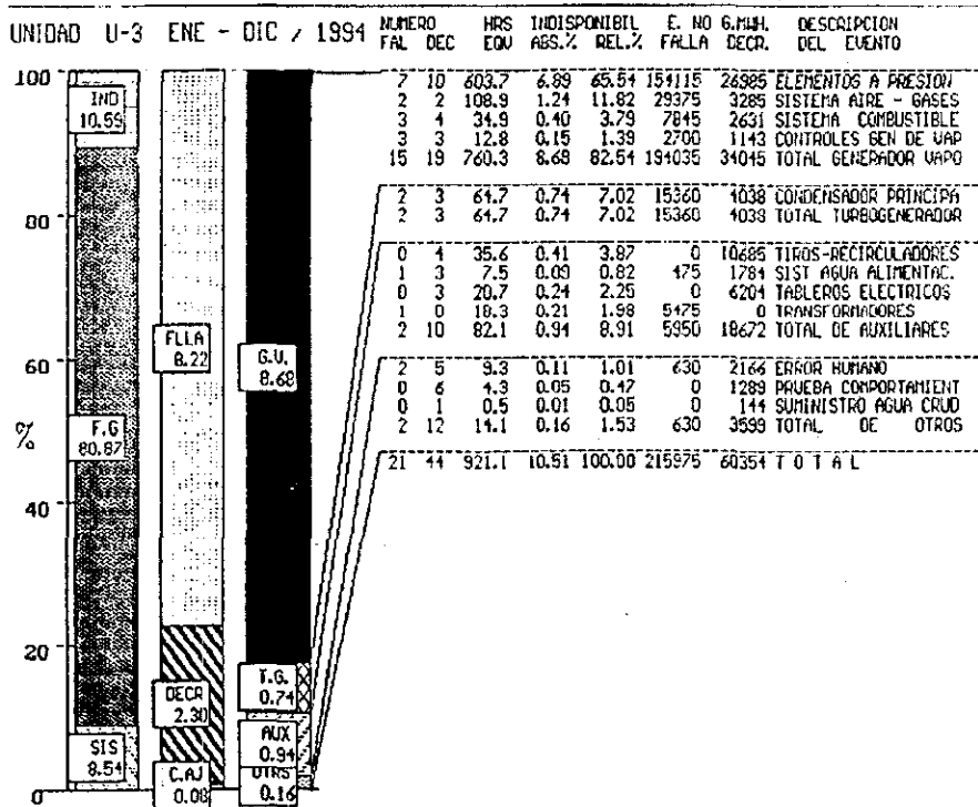
Figura V.3 Disponibilidad e Indisponibilidad de U-3 en 1994
