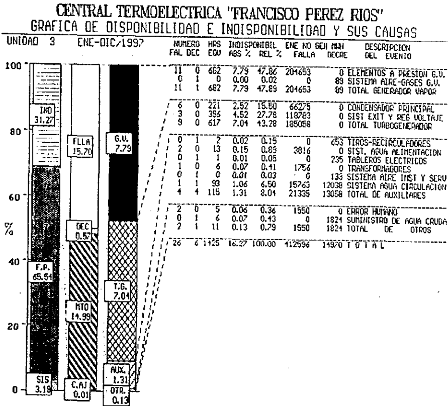
Figura V.6 Disponibilidad e Indisponibilidad de U-3 en 1997
