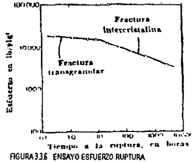
Figura III.9 Ensayo Esfuerzo Ruptura
