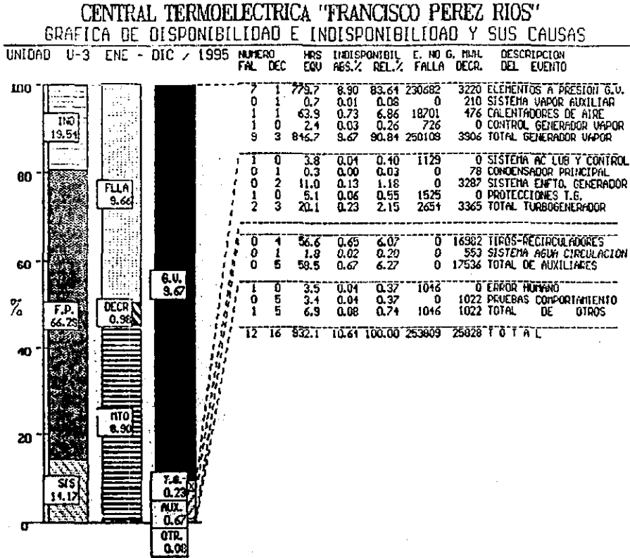
Figura V.4 Disponibilidad e Indisponibilidad de U-3 en 1995
