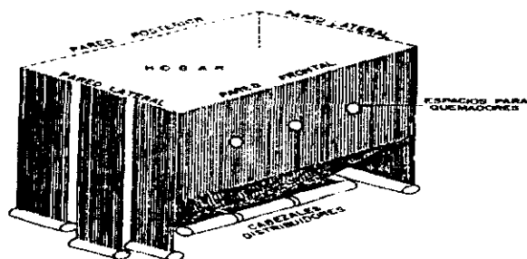
Figura V.1 Distribución de tubería en las paredes de agua de una caldera
