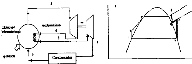
Fig. I.2. Diagrama de bloques y diagrama T-S de ciclo Rankine con recalentamiento.
