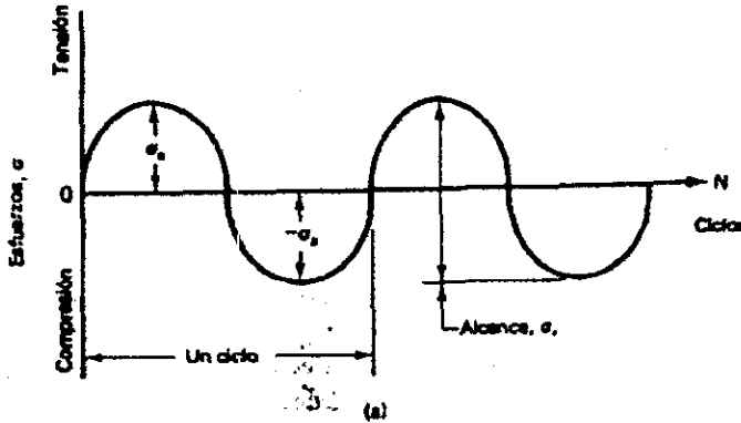
Fig. III.1 Diagrama de Esfuerzos cíclicos
