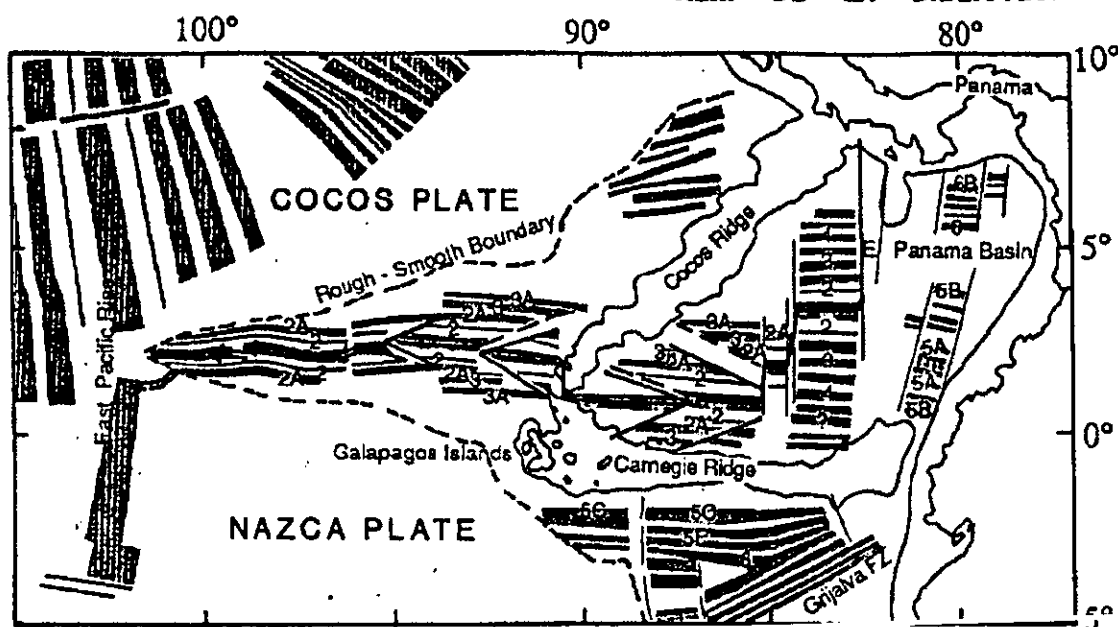
Figura 5.11: Anomalías magnéticas generadas por el esparramiento del piso oceánico entre las Placas de Cocos y Nazca, desde hace 25 m.a hasta el presente. Se observan las anomalías 5A, 5B, 6, 6B junto a la Trinchera de Colombia. También se observa un centro de esparramiento a la altura de la latitud 2° N. tomado de Atwater[1989]
