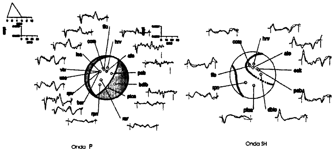
Figura 3.7: Parámetros focales del sismo del 8 de Febrero de 1995. El mecanismo focal y la profundidad fueron determinados usando una función formal de inversión de forma de ondas telestsmicas P y SH, [Nábelek , 1984]. Los mecanismos focales se muestran en el hemisferio inferior de la esfera focal. La línea sólida corresponde a la forma de onda observada y la línea punteada a la forma de onda sintética. La función de la fuente es de 8 segundos, se obtuvo un error cuadrático medio=0.57 \mu\text{m} .
