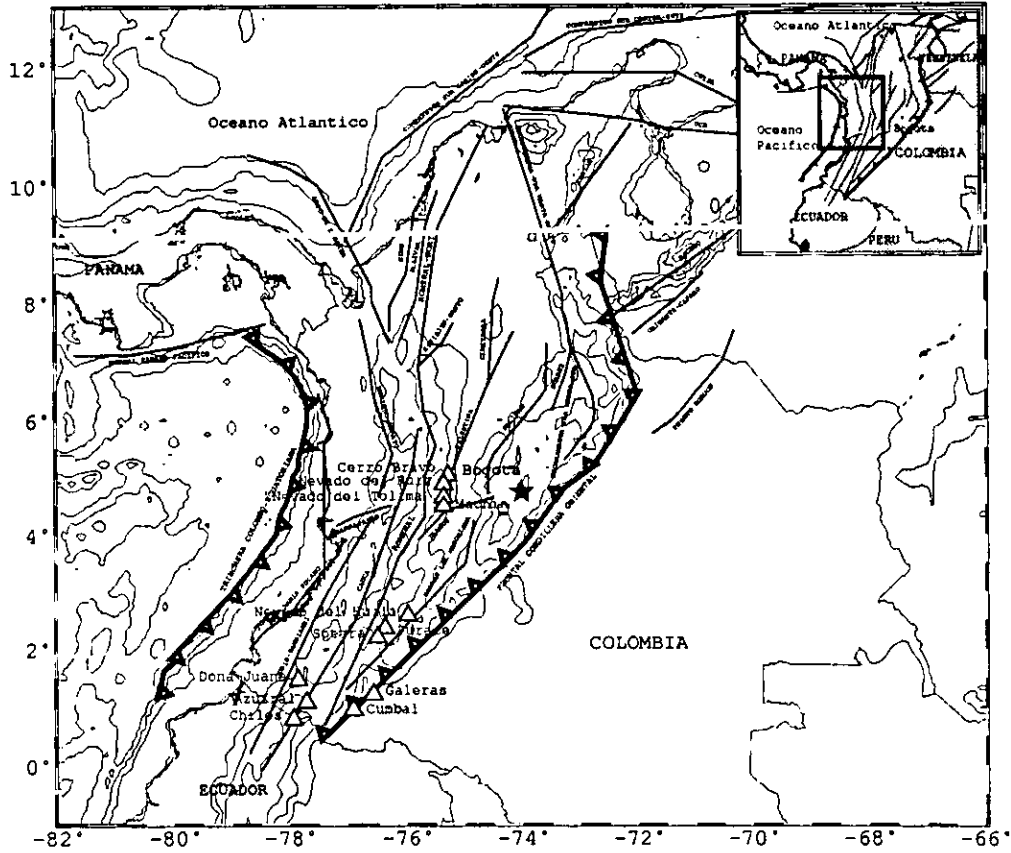
Figura 1.1: En el recuadro superior se señala la zona de estudio, ubicada entre las latitudes 4°N–9°N, que se ha denominado el Noroeste de Colombia. Se muestra la Trinchera Colombo-Ecuatoriana; los volcanes activos, señalados con triángulos, la topografía de la región Andina y el sistema de fallas geológicas que atraviesan la región Andina Colombiana.
