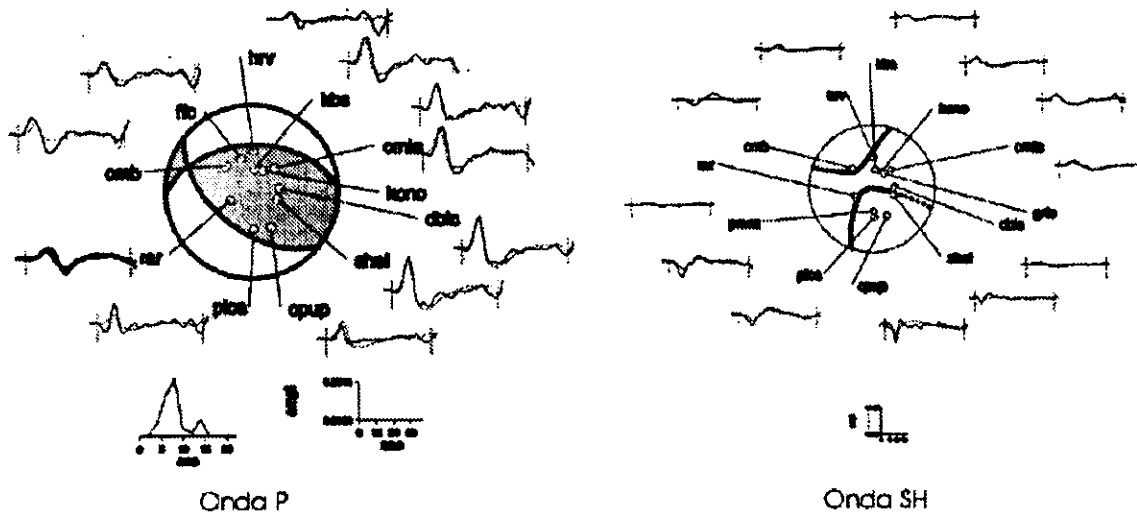
Figura 3.11: Parámetros focales de los sismos del 3 de Junio de 1994 y del sismo de 2 de Septiembre de 1997. Los mecanismos focales y la profundidad fueron determinados usando una función formal de inversión de forma de ondas telesísmicas P (lado izquierdo) y de SH (lado derecho) [Nábelek , 1984 ]. Los mecanismos focales se muestran en el hemisferio inferior de la esfera focal. La línea sólida corresponde a la forma de onda observada y la línea punteada a la forma de onda sintética.
