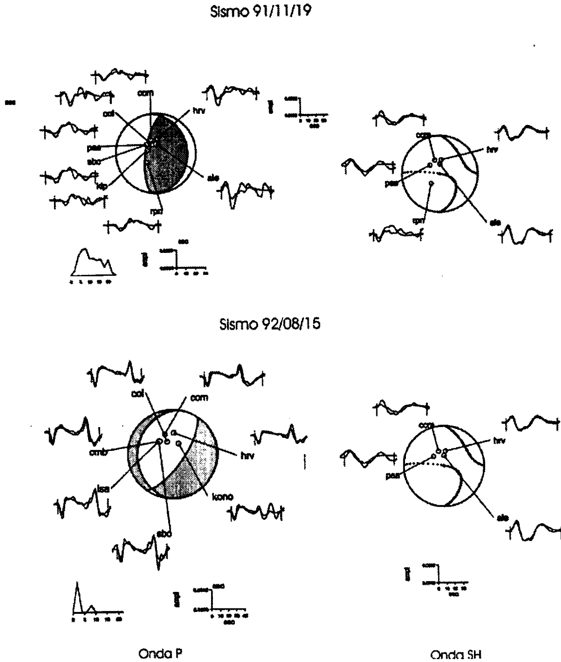
Figura 3.10: Parámetros focales del sismo del 19 de Noviembre de 1991 y del sismo de 15 de Agosto de 1992. Los mecanismos focales y la profundidad fueron determinados usando una función formal de inversión de forma de ondas telesísmicas P (lado izquierdo) y de SH (lado derecho) [Nábelek , 1984 ]. Los mecanismos focales se muestran en el hemisferio inferior de la esfera focal. La línea sólida corresponde a la forma de onda observada y la línea punteada a la forma de onda sintética.
