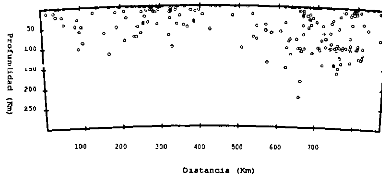
Figura 5.10: Perfiles transversales de las secciones hipocentrales del Segmento murindó y el Segmento Cauca a lo largo de la Trinchera. Los hipocentros representados corresponden al catálogo de eventos relocalizados con JHD, período Enero 1964- Abril 19948.
