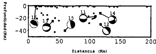
Figura 5.9: Perfiles transversal de las sección en la frontera Colombia-Panamá. Los hipocentros representados corresponden al catálogo de eventos relocalizados con JHD en el presente estudio, período Enero 1964- Abril 1998. Los cuadros sólidos son los eventos con mecanismos focales.
