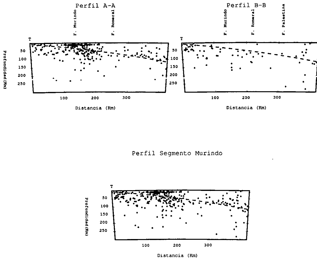
Figura 4.7: Perfiles transversales de las secciones hipocentrales del Segmento Murindó. Los hipocentros representados corresponden al catalogo de ISC, periodo Enero 1964- Diciembre 1994, a los que solo se les depuró los hipocentros de H=0 km y H=33.0 Km. Se puede observar que la sismicidad está muy difusa, se muestra la zona de Wadati-Benioff propuesta en este estudio.
