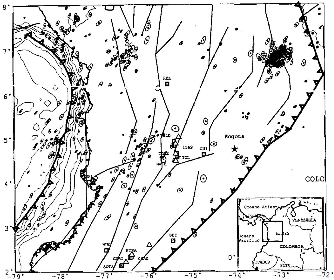
Figura 3.14: Se muestran las elipses de error para los 550 eventos relocados con JHD (Dewey, 1989).
