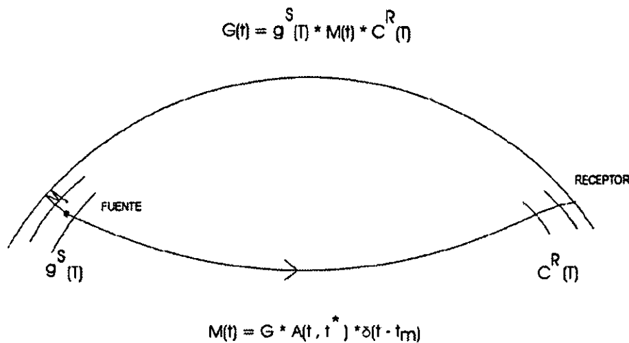
Figura 3.1: En forma esquemática se muestra la manera más simple de calcular las funciones de Green de ondas de cuerpo tele sísmicas. M(t) = Funciones de respuesta del manto, C^R(t) = Respuesta cortical en el receptor, g^S(t) = Funciones de respuesta de la fuente, G(t) = Función de Green .
