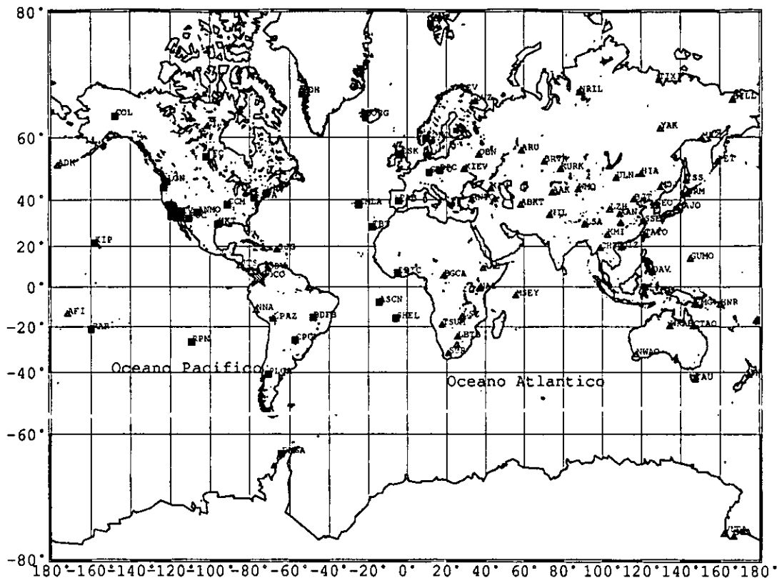
Figura 3.4: Estaciones de la Red Sismica Mundial. Las estaciones marcadas con rectángulo sólido corresponden a las estaciones en el rango 30^\circ \leq \Delta \leq 90^\circ y las marcadas con triángulos sólidos las que quedan fuera del rango apropiados para la inversión de forma de onda
