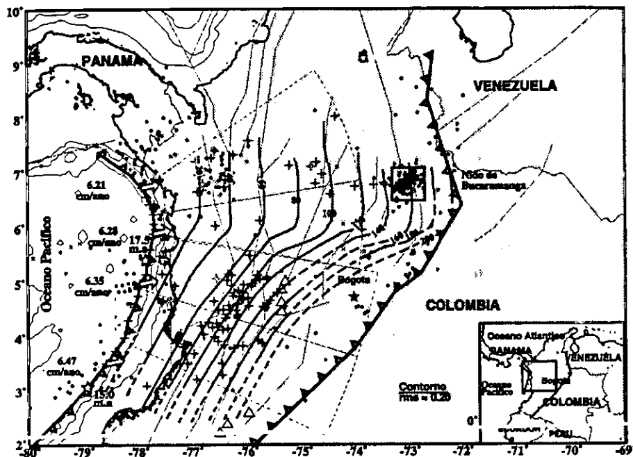
Figura 5.1: Contorno de isopropfundidades de la placa oceánica subducida bajo la placa de Suramérica en el Noroeste de Colombia, se dibujó usando splines de interpolación. Los eventos señalados con (+) son los eventos que se emplearon para la interpolación y corresponden a los que pertenecen a la placa subducida. Las líneas punteadas indican el contorno extrapolado por carencia de datos. Las flechas blancas indican la dirección de convergencia propuesta por DeMets et al [1990,1994]; las estrellas blancas en la trinchera son los puntos donde se proyectan las anomalías para obtener edades de la placa, [Atwater, 1989]
