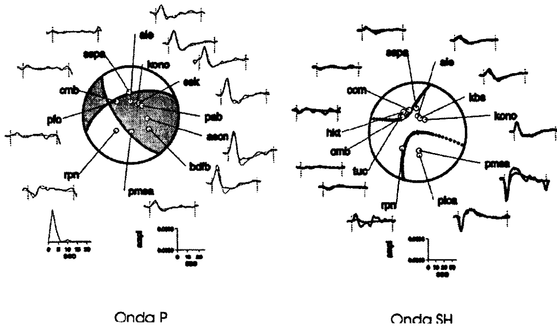
Figura 3.12: Parámetros focales del sismo del 11 de Diciembre de 1997. Los mecanismos focales y la profundidad fueron determinados usando una función formal de inversión de forma de ondas telúsmicas P (lado izquierdo) y de SH (lado derecho) [Nábelek, 1984]. Los mecanismos focales se muestran en el hemisferio inferior de la esfera focal. La línea sólida corresponde a la forma de onda observada y la línea punteada a la forma de onda sintética.
