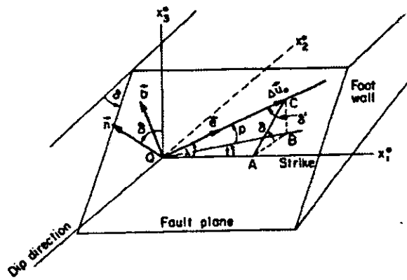
Figura 5.2: Convenciones para los ángulos y parámetros para los parámetros de la falla. Donde: \lambda = Deslizamiento a lo largo del vector de deslizamiento ( Rake), \delta =Buzamiento ( Dip), p = Inclinación ( Plunge), t = azimuth ( Trend), e, n, b son los vectores unitarios de deslizamiento, normal y nulo respectivamente, tomado de Ben-Menahem[1980].
