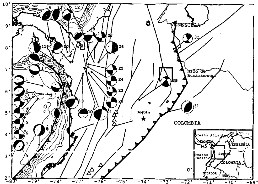
Figura 5.3: Mecanismos focales superficiales mostrados en la esfera focal inferior. Estos mecanismos corresponden a los eventos relocalizados con JHD y que quedarían en la corteza. Los mecanismos en rojo son los que se le hicieron inversión en este estudio, el resto son reportados por Harvard-CMT y Pennington[1981].
