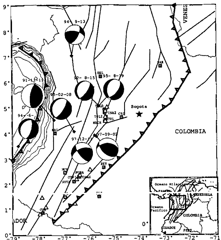
Figura 3.2: Localización de los eventos que se invirtieron en el presente estudio y las respectivas soluciones del plano de falla. Los cuadros sólidos representan las estaciones de la Red Sísmica Nacional de Colombia [RSNC], la cruz (+) es el evento relocado con JHD. La convención para los parámetros de falla es la misma que la de Aki y Richards[1980].
