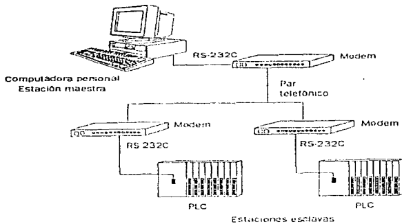
Esquema-Bus de comunicaciones multidrop implementado en la norma RS232-C y modems
