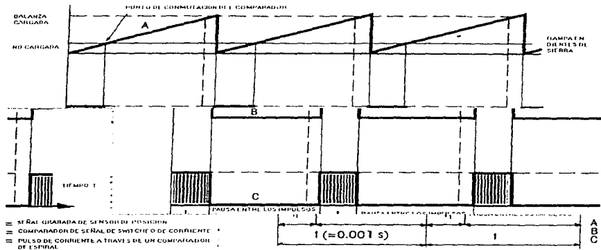
Compensación electromagnética de fuerzas
