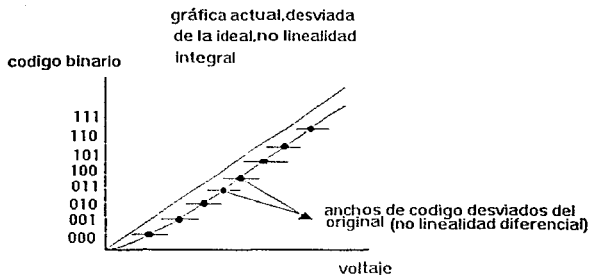
Figura 5 Gráfica de voltaje de código binario mostrando la no linealidad.
