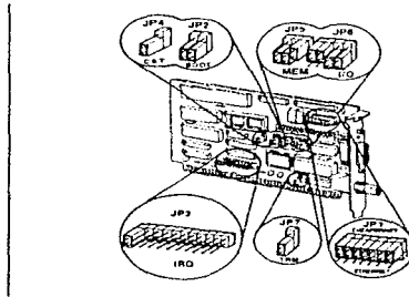
TARJETA ADAPTADORA DE RED
