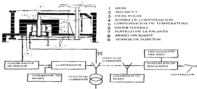
Figura: Principio de una balanza de compensación electromagnética de fuerza
