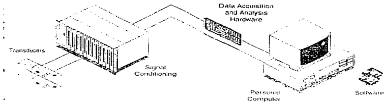
Un típico sistema de adquisición de datos
