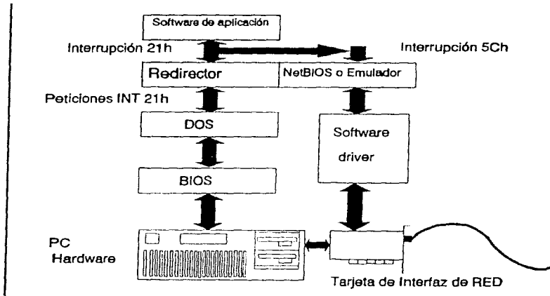
Diagrama de Bloques de una estación de Trabajo.
