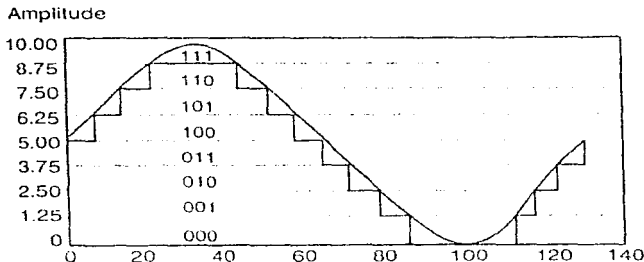
La figura nos muestra una onda senoidal digitalizada con una resolución de 3-bit
