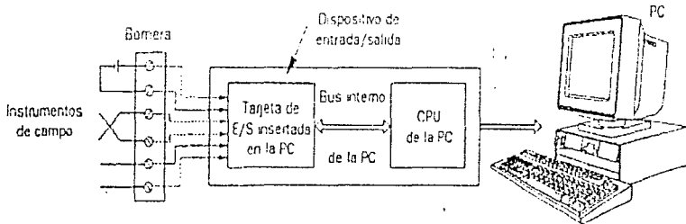
Esquema de un sistema interno
