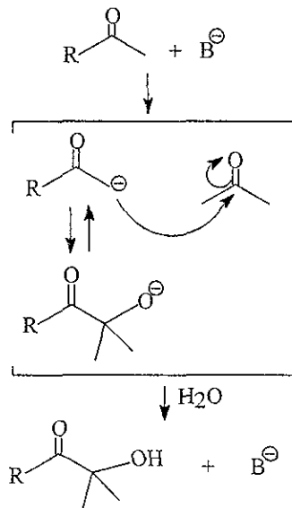
Esquema 2. Mecanismo de condensación carbonílica
