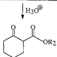
Esquema 3. Mecanismo de ciclación de Dieckmann
