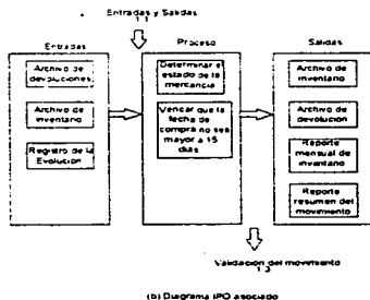
Figura 2.8b Diagrama asociado IPO del proceso 1.2 "Devolución de mercancía".
