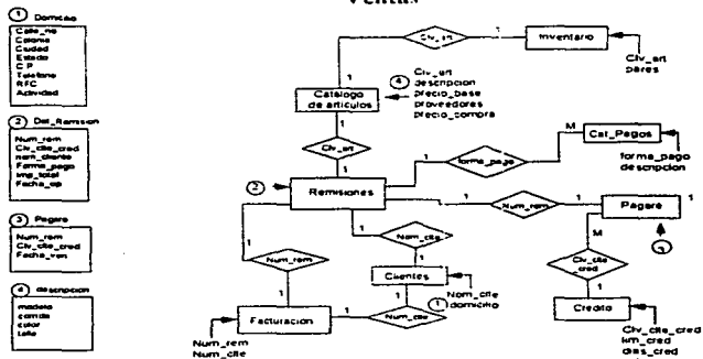
Figura 4.3 Modelo Entidad-Relación de Ventas.
