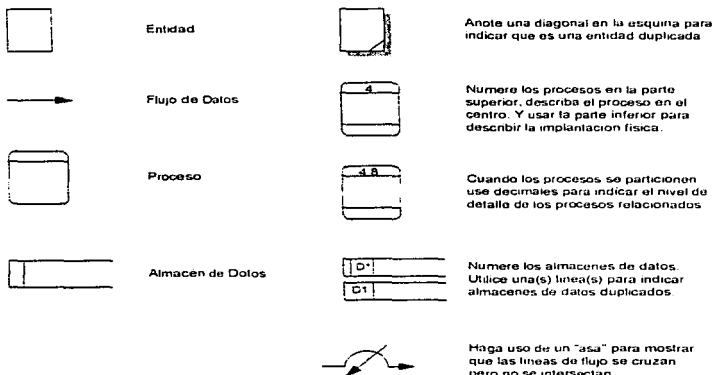
Fig. 2.4a Símbolos usados en adicionales los diagramas de flujo de datos.
