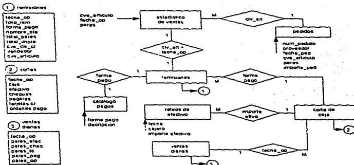
Figura 4.4 Modelo Entidad-Relación del Cierre del día.
