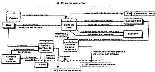
Figura 3.6 Diagrama del cierre del día.
