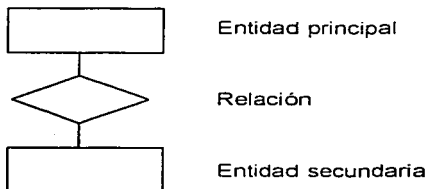
Figura 2.12 Elementos de un diagrama de relación-entidad (E-R).
