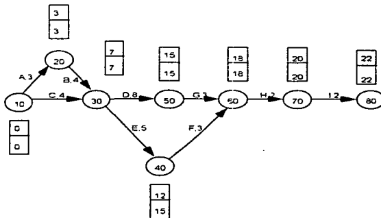
Figura 2.11. Una gráfica PERT, con la ruta crítica y los valores ECT, LAT, de cada evento.
