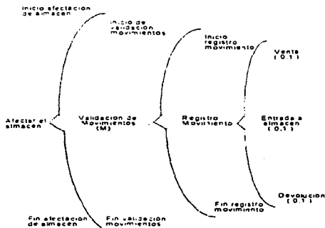
Figura 2.9 Ejemplo de diagrama de Warnier/Orr para el proceso "Afectación al almacén".
