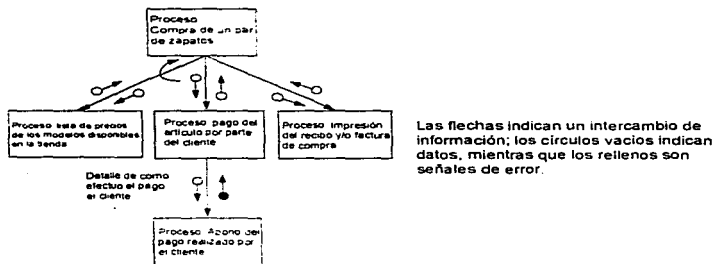
Figura 2.5 Ejemplo de diagrama estructurado.
