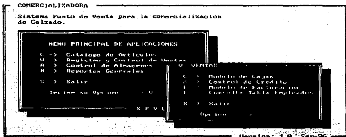
Figura 7.2 Pantalla general de acceso.
