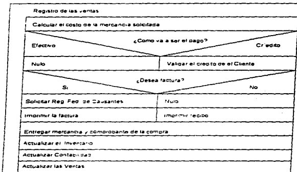
Figura 2.7 Ejemplo de un diagrama de flujo estructurado.
