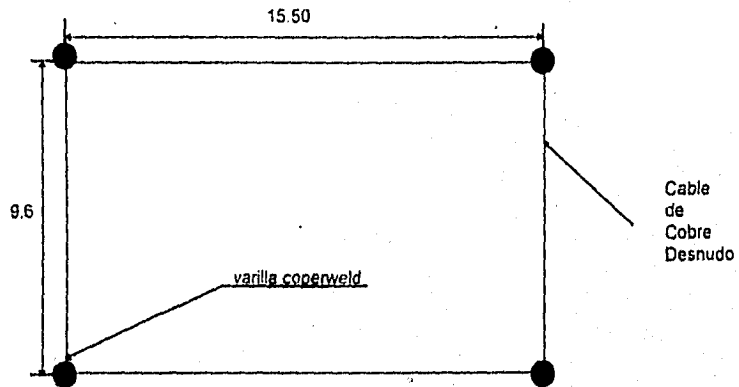
Figura 4.4.3 Diseño preliminar de la red.
