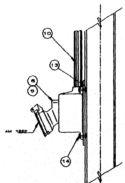
DETALLE No 2
