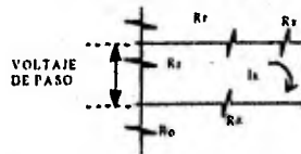
Circuito equivalente
