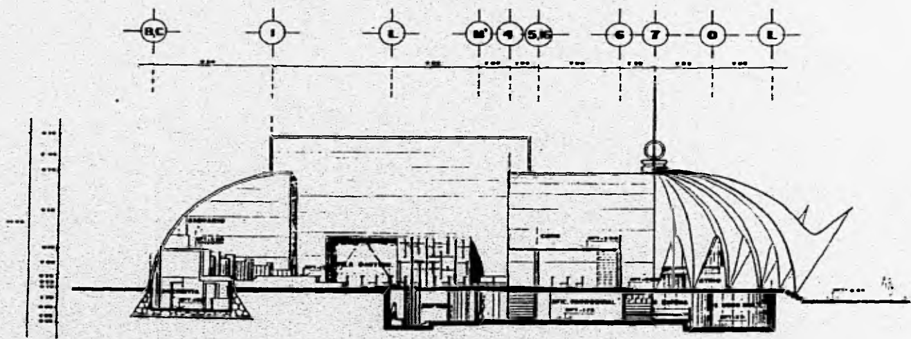
CORTE TRANSVERSAL X-X'
