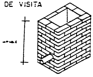
REGISTRO DE 60 x 90
