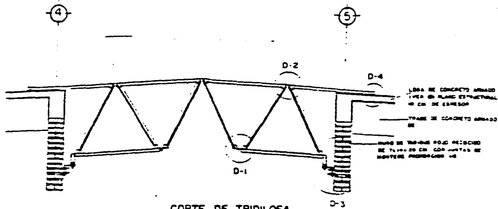
CORTE DE TRIDILOSA
