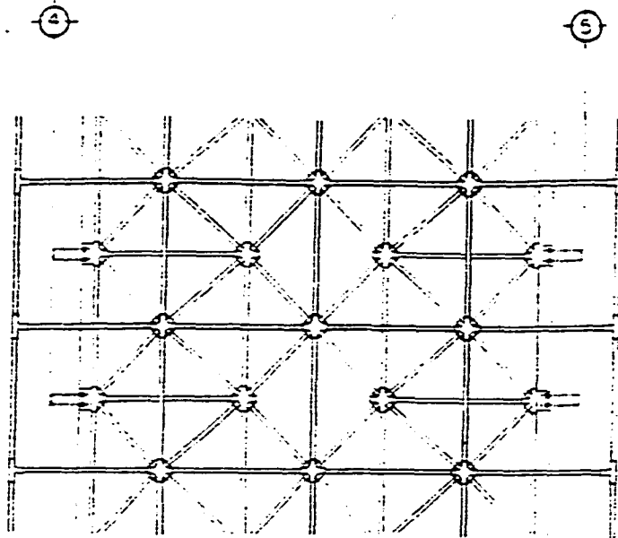
PLANTA DE TRIDILOSA
