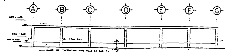
MARCO EN EJES 1 y 7
