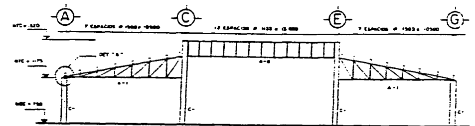
MARCO EN EJES 2 y 6
