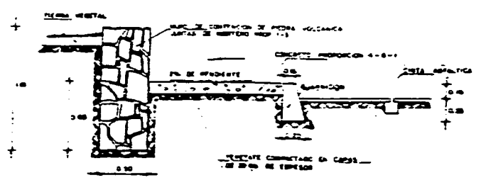
DETALLE JARDINERA - GUARNICION - CINTA ASFALTICA
