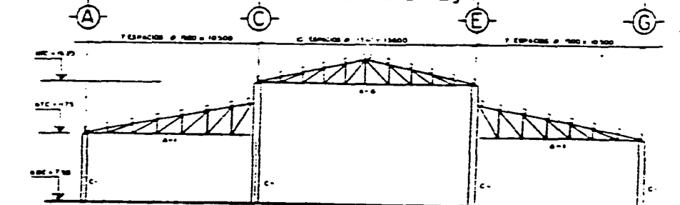
MARCO EN EJE 4
