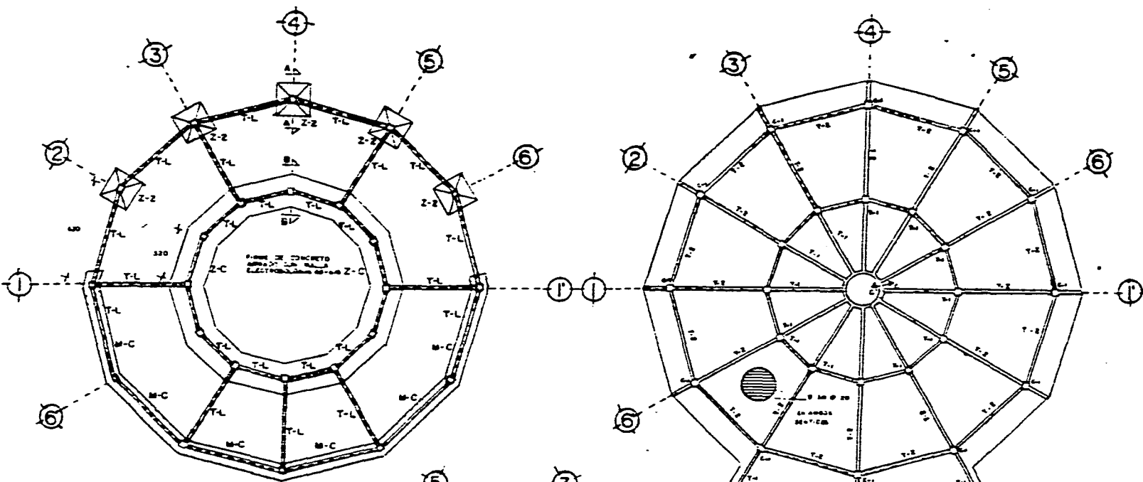
PLANTA DE CIMENTACION
