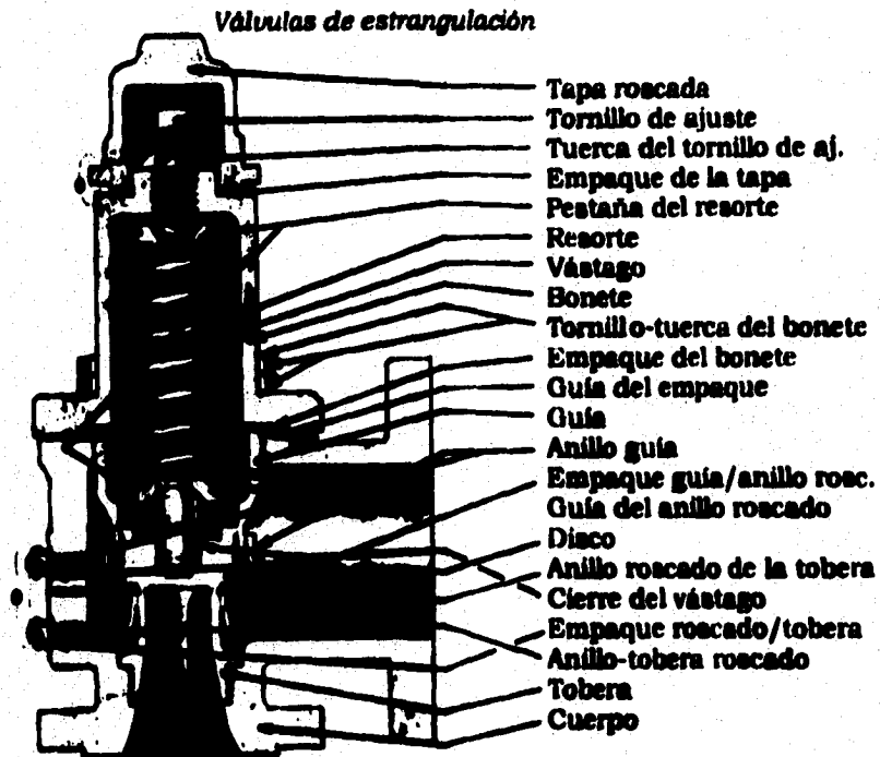
Figura 3-14. Válvula de seguridad
