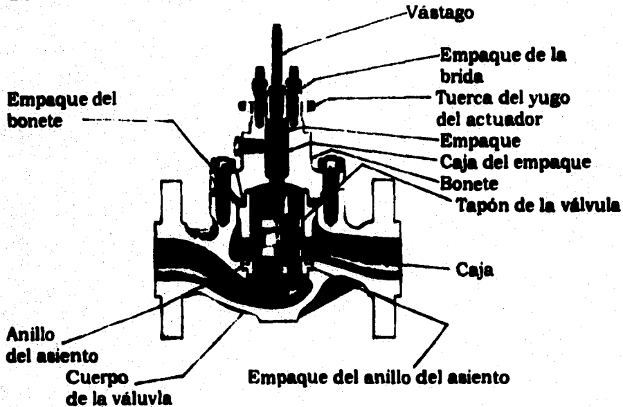
Figura 3-27. Válvulas de vástago deslizante.
