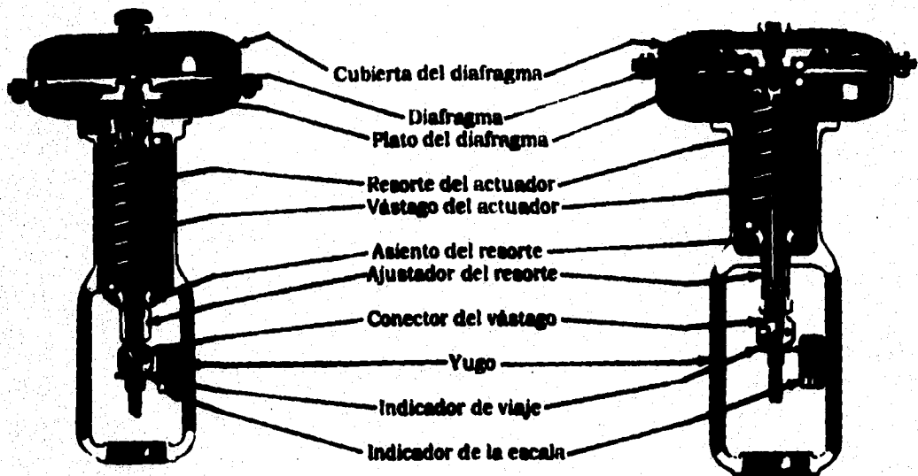
Figura 5-1. Actuador para válvulas de movimiento deslizante.
