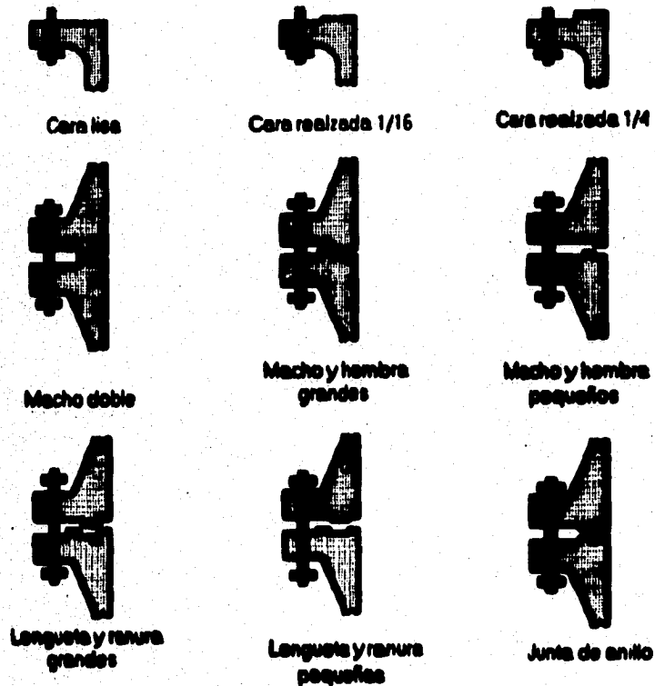
Figura 4-2. Caras de contacto de bridas estándar.
