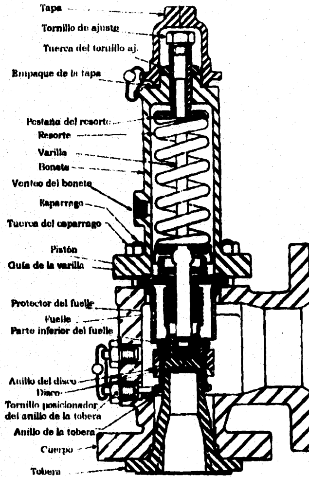
Figura 3-20. Válvula de desahogo tipo pistón.
