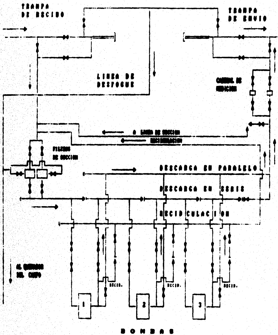
Figura 6-2 Diagrama de flujo de estación de bombas para gasolina
