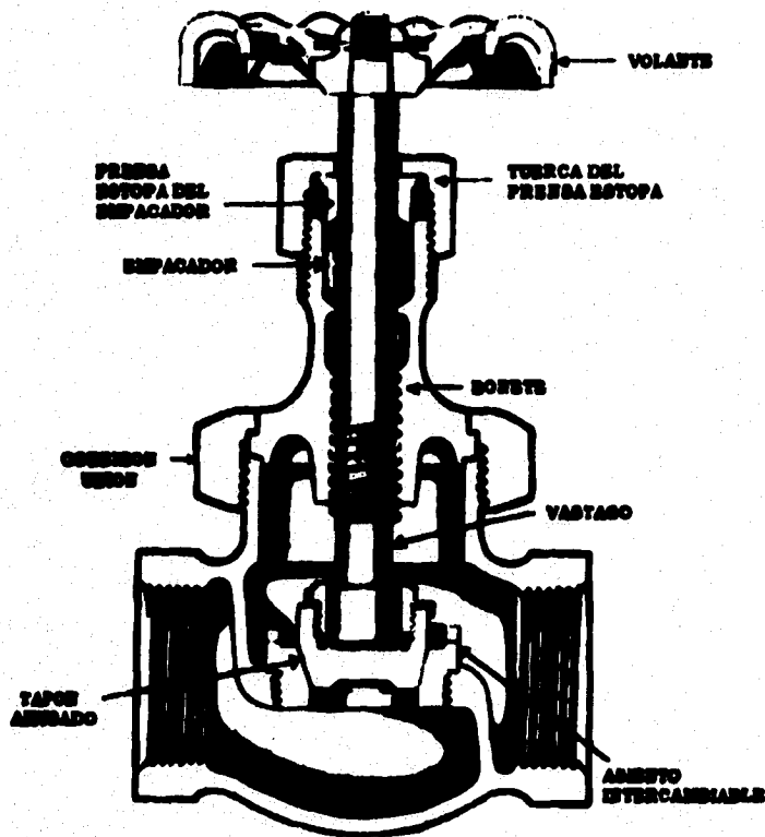
Figura 3-3. Válvula de globo con disco macho metálico.
