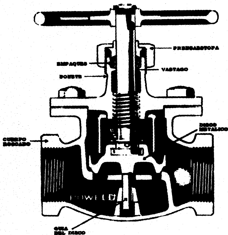
Figura 3-4. Válvula de globo con disco plano metálico o también conocido como disco de composición.
