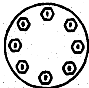
Figura 5-12. Secuencia de apriete de espárragos o tornillos.
