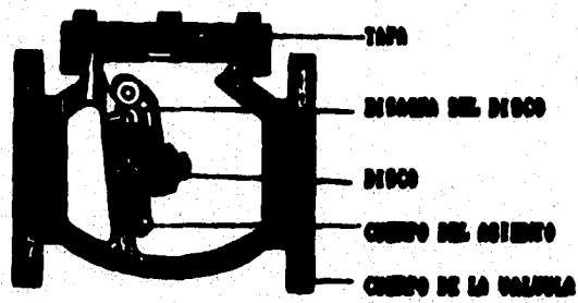
Figura 2-23 Válvula de retención tipo bisagra
