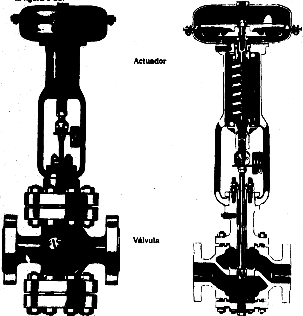
Figura 3-25. Elementos básicos de la válvula de control
