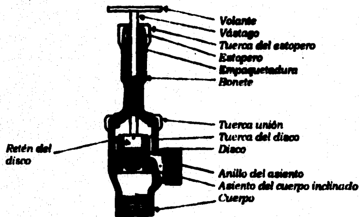
Figura 3-9. Componentes de una válvula de ángulo.
