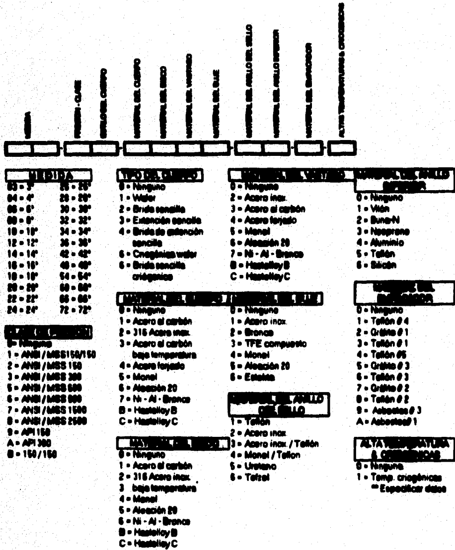
Figura 4-5. Código de productos para válvulas.
