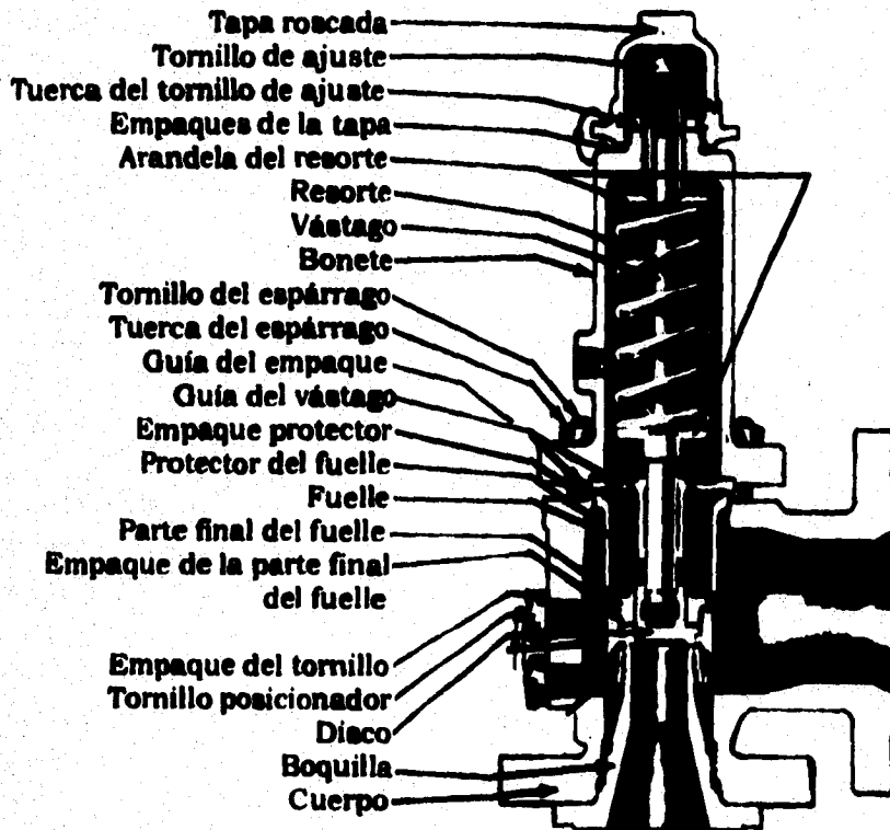
Figura 3-17. Válvula de seguridad-alivio balanceada con fuelle.
