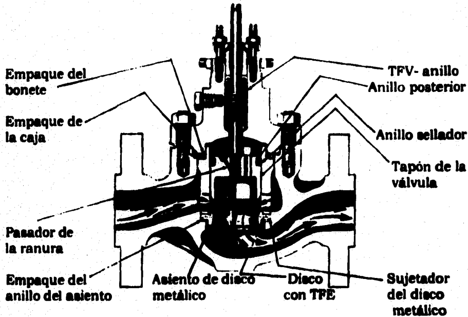
Figura 3-28. Válvula de puerto sencillo o único.
