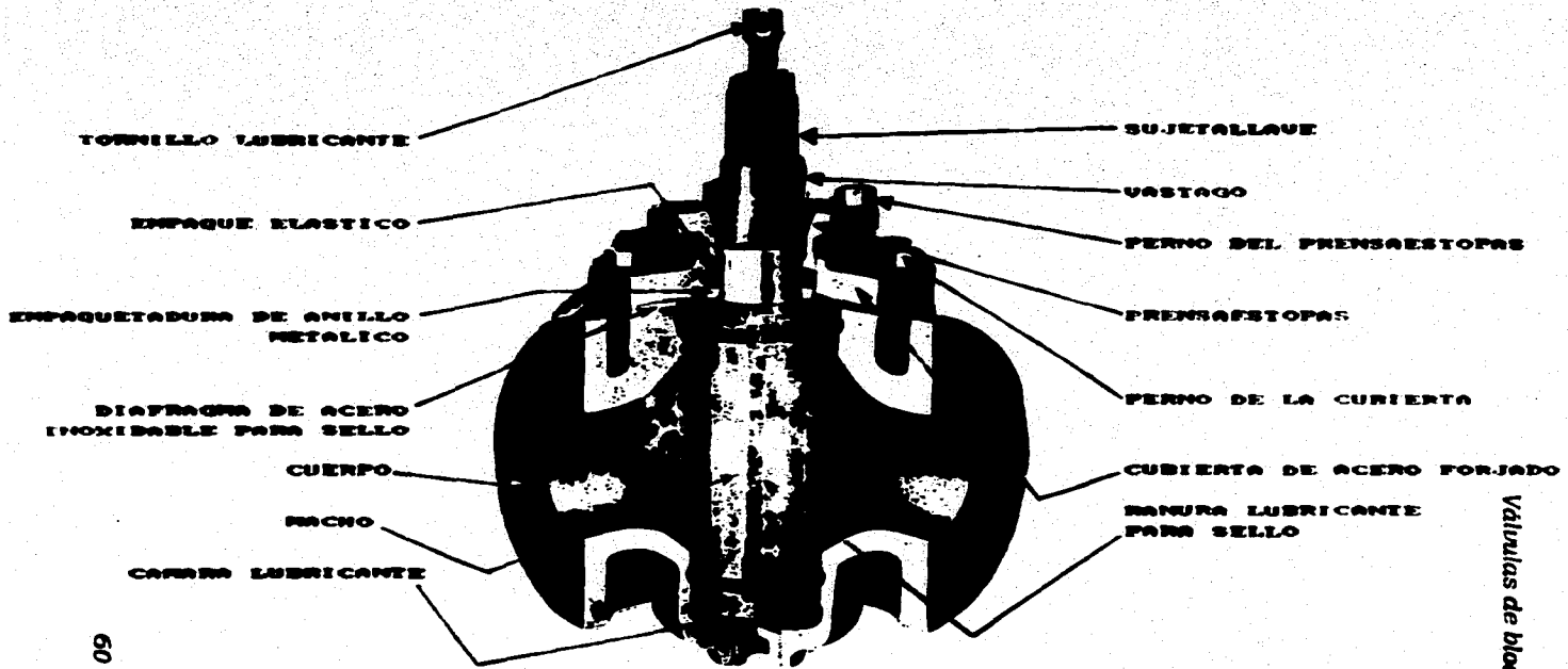
Figura 2-24 Válvula de macho "Nordstrom" tipo multipuertos
