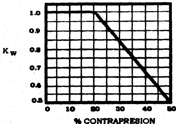
Figura 3-23. Gráfica para calcular el factor de corrección por capacidad, debido a la contrapresión, y es solo si se emplean válvulas de fule.
