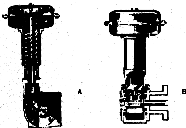
Figura 5-2. (A) y (B), Muestra un actuador de diafragma y resorte para válvulas convástago rotatorio.
