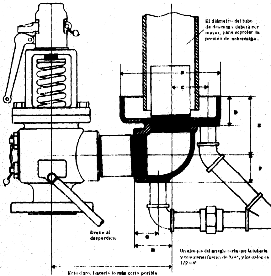
Figura 3-16. Diagrama de descarga de una válvula.
