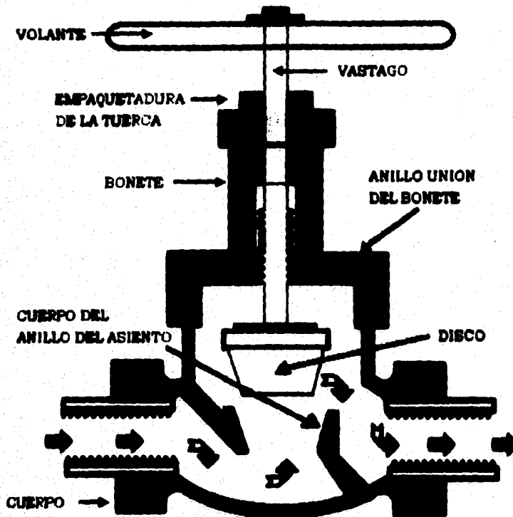
Figura 3-1. Válvula de globo.
