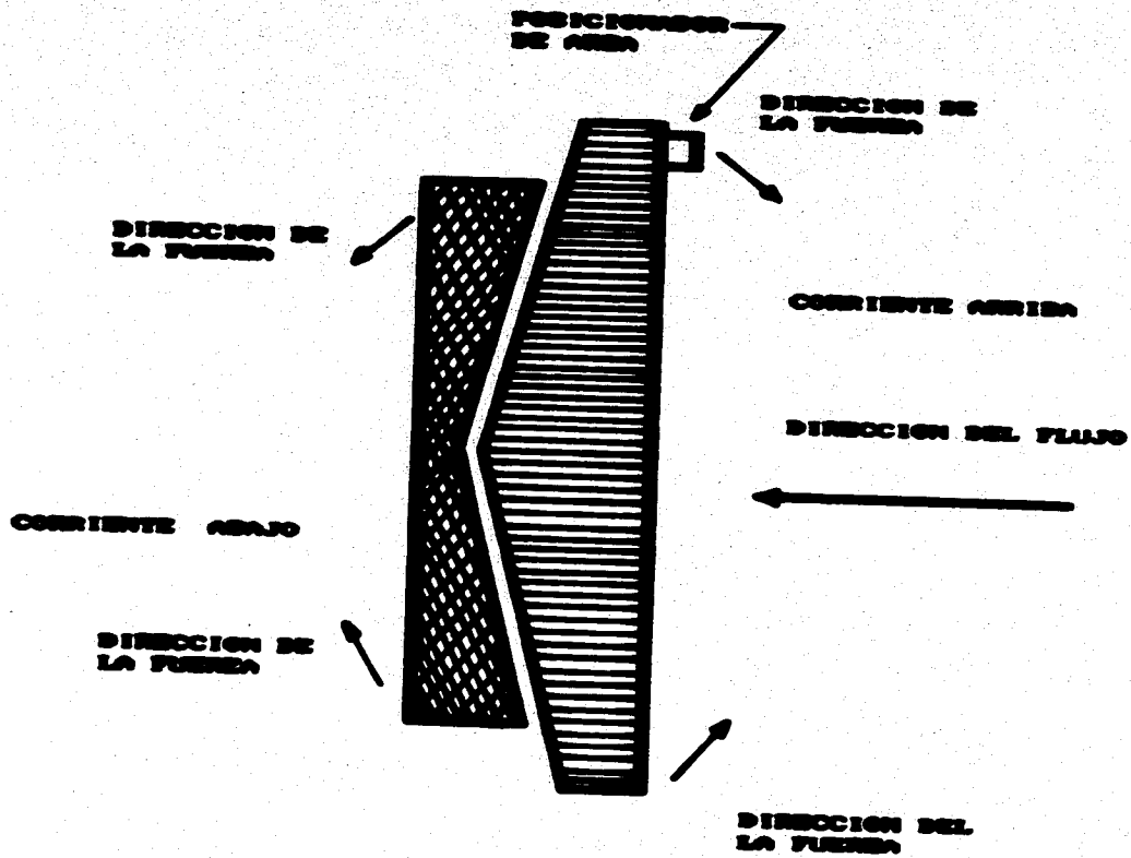
Figura 2-7 Ensamble de la compuerta de expansion paralela
