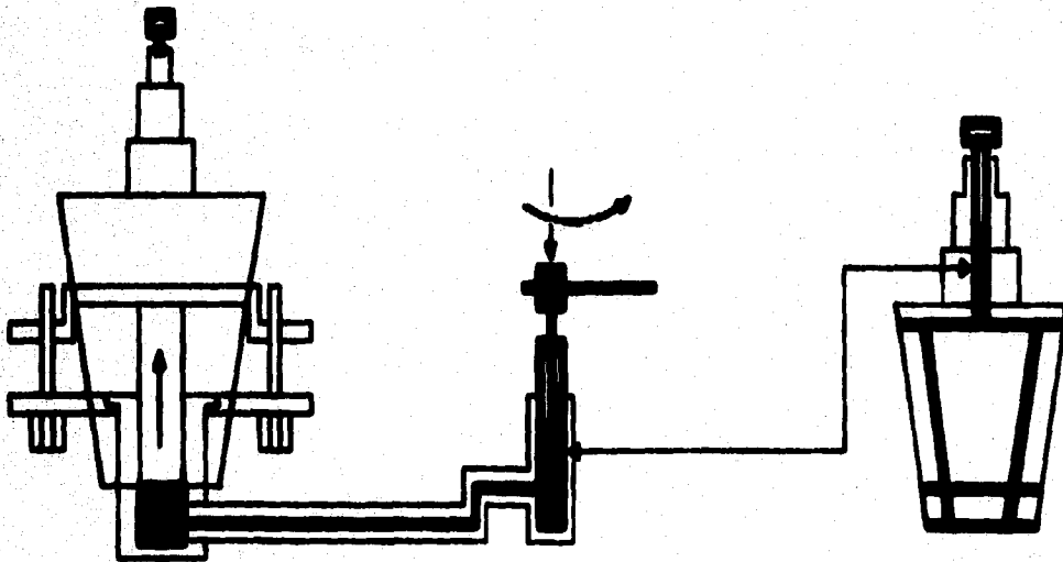
Figura 2-13 Principio de Pascal aplicado a Válvulas de Macho
