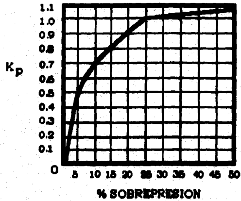
Figura 3-22. Gráfica por factor de corrección por capacidad, debido a la sobrepresión, para válvulas de seguridad y alivio que manejen líquidos.
