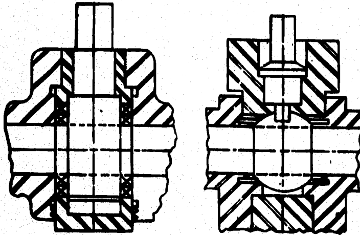
CILINDRICO
