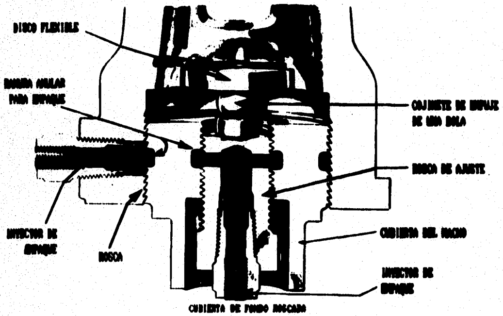
Figura 2-23 Dos tipos de cierre de fondo usados en válvulas "Hyprosol"
