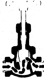
Figura 3-2. Trayectoria del flujo en una válvula tipo globo.
