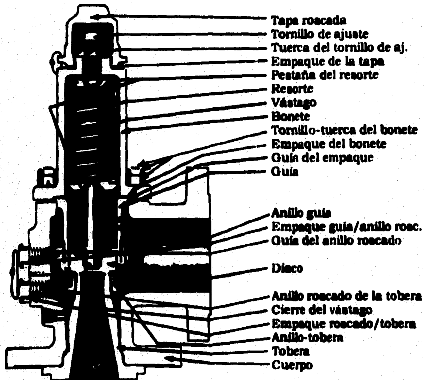
Figura 3-13. Boquilla de la válvula de seguridad.
