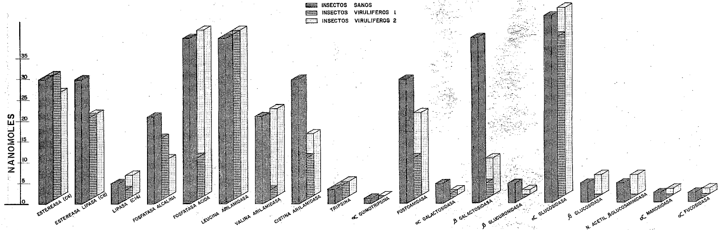
GRAFICA 3 ACTIVIDAD ENZIMÁTICA DEL MESENTERON DE DALBULUS ELIMATUS (BALL)
