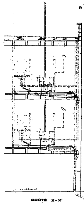
CORTE X-X'
