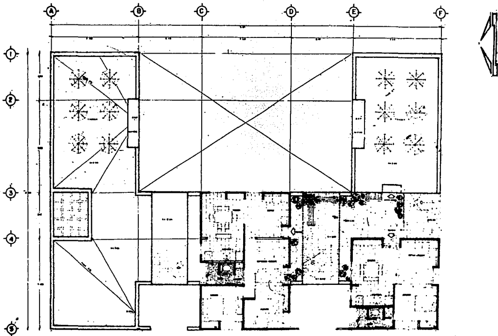
PLANTA ARQUITECTONICA 3 er NIVEL
