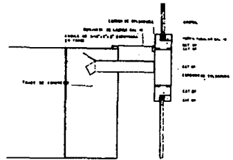
ANCLAJE DE HERRERIA
