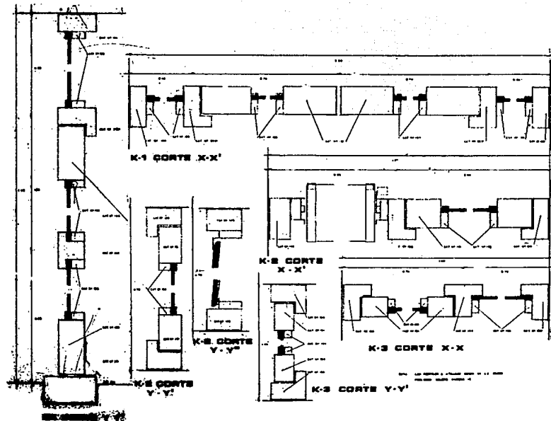
PLANO DE HERRERIA
