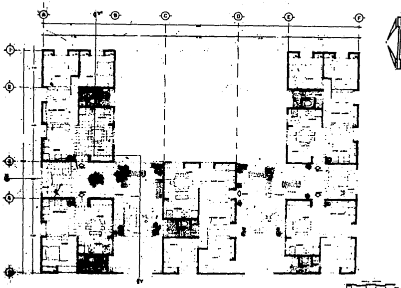
PLANTA ARQUITECTONICA 2º NIVEL
