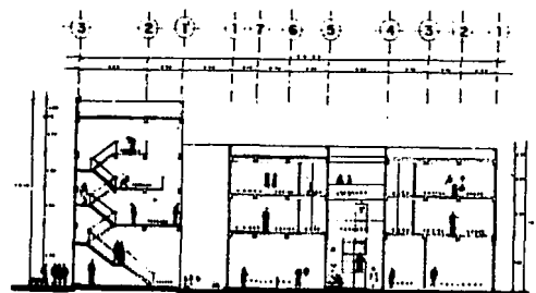
CORTE TRANSVERSAL
