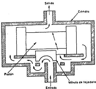
Fig. II.1.2.3 Medidor de pistón convencional.
