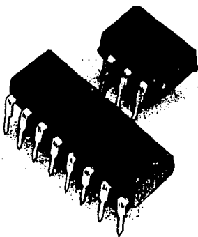
Fig. II.3.1.5 Paquetes y configuraciones de pines de los opto-aisladores Litronix ISO-LIT 1 y el ISO-LIT Q1.
