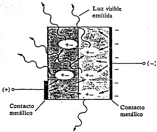
Fig. II.4b.1 Proceso de electroluminiscencia en el LED.
