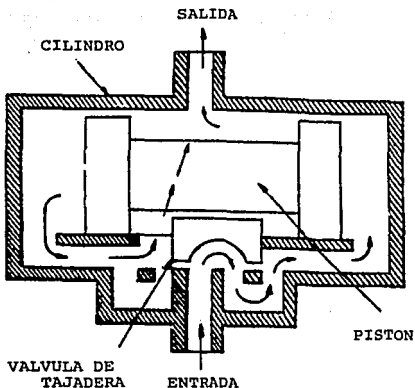
Fig. II.3.2 Llenado de cámara derecha y vaciado de la izquierda.
