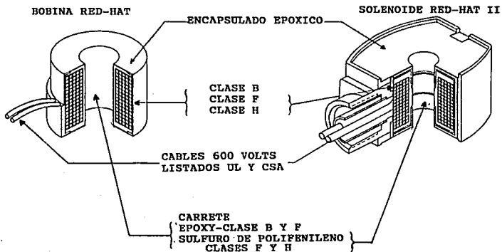
Fig. II.2.2.4 Tipos de aislamiento y limitaciones de temperatura de los solenoides.
