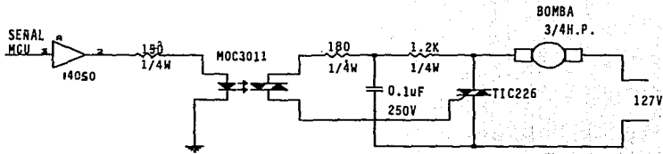
Fig. III.3a.2 Circuito de activación de la bomba.
