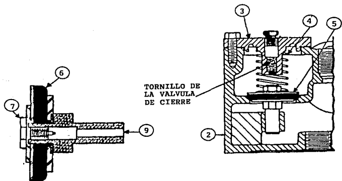
Fig. II.2.5.1 Válvula de control o de retención.
