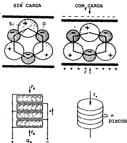
Fig. II.1.1.6 El efecto piezoeléctrico.
