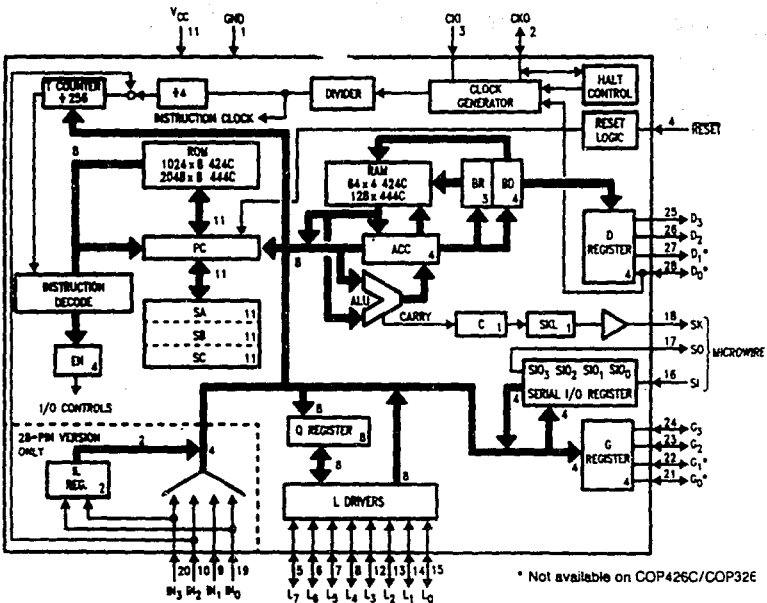
Fig. III.2.2.8 Diagrama a bloques de los siguientes MCU'S:
