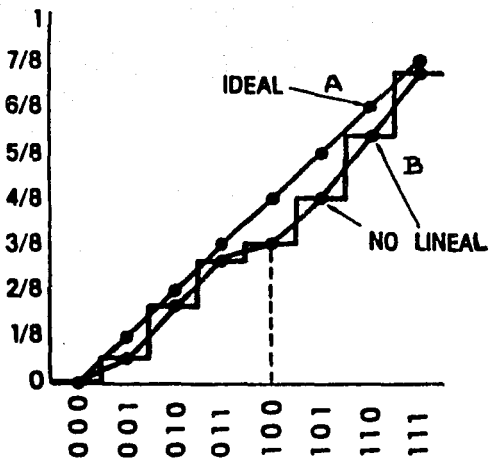
Fig. A.1.3.1 Error de linealidad.
