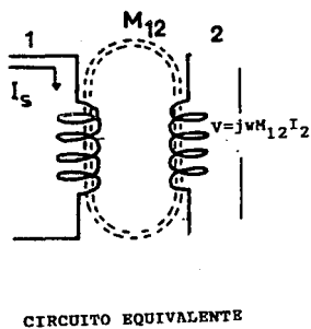
Fig. III.3c.2.1 Representación física y circuito equivalente de los campos eléctrico y magnético.
