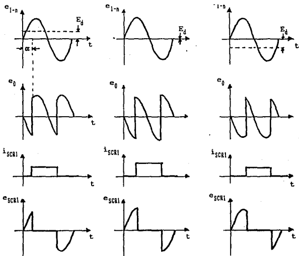
Fig. III.3d.2.2 Rectificador controlado por fase.
