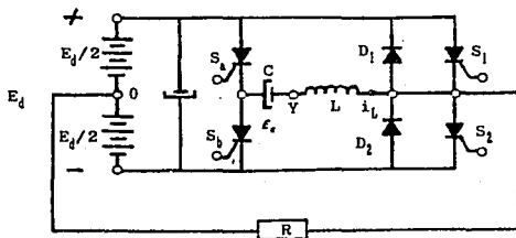
Fig. D.II.4 Inversor conmutado por impulso.
