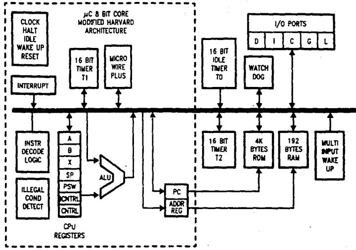
Fig. III.2.2.12 Diagrama a bloques del MCU COP888CL.
