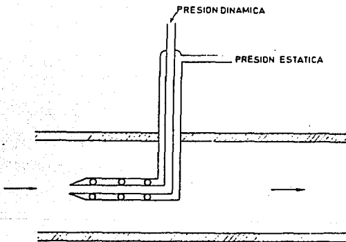
Fig. II.1.2.12 Tubo de Pitot.
