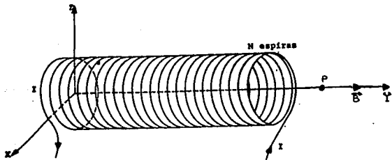
Fig. II.3.3.1 Campo magnético producido en el punto P , debido a la circulación de la corriente I por el solenoide.
