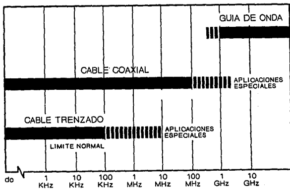
Fig. III.3c.4.13 Propagación en diferentes tipos de cables.
