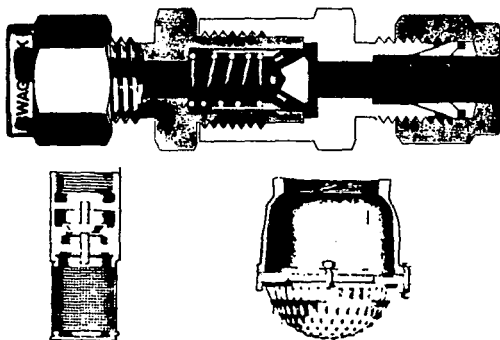
Fig. II.2.3.4 Válvulas de movimiento vertical o válvulas "check".
