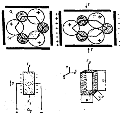
Fig. II.1.1.7 Efecto piezoeléctrico transversal.
