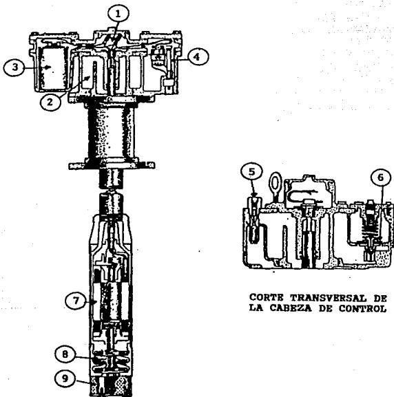
Fig. I.2.1.5 Bomba para sistemas de control remoto.
