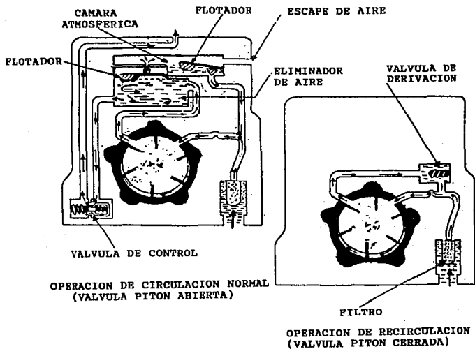
Fig. I.2.1.2 Operación de las unidades de bombeo de succión directa.
