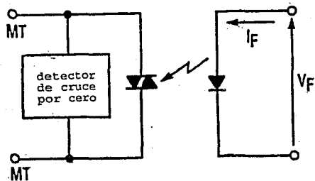
Fig. II.3.1.9 Esquema de un Driver aislado ópticamente de cruce por cero.
