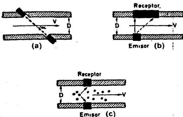
Fig. II.1.2.17 Medición de caudal por ultrasonidos. a) Diferencia de tiempo, de fase o de frecuencia, b) Desviación del haz, c) Método Doppler.
