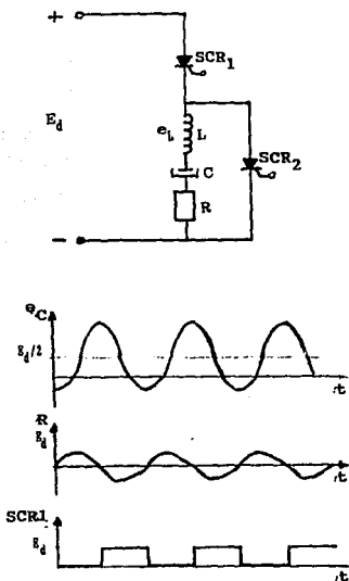
Fig. D.II.3 Inversor conmutado por capacitor en serie.
