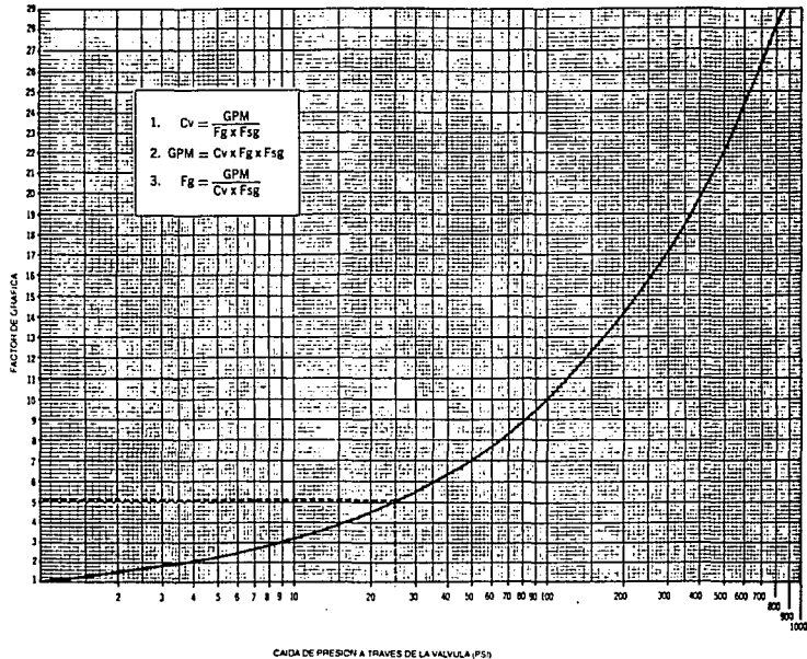
Figura II.2.2.5 Gráfica para obtener el factor F_g .
