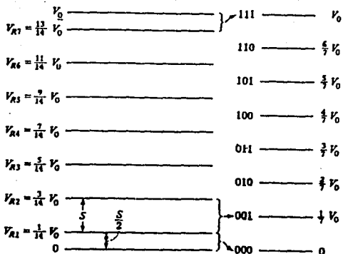
Fig. A.1.2.3 Equivalencia entre voltajes de entrada analógicos con combinaciones binarias y voltajes de salida.
