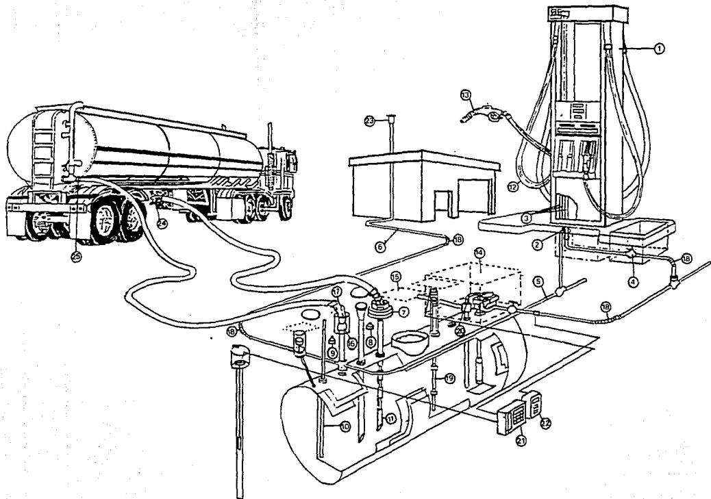
Fig. I.1.1 Sistema general de una estación de servicio.
