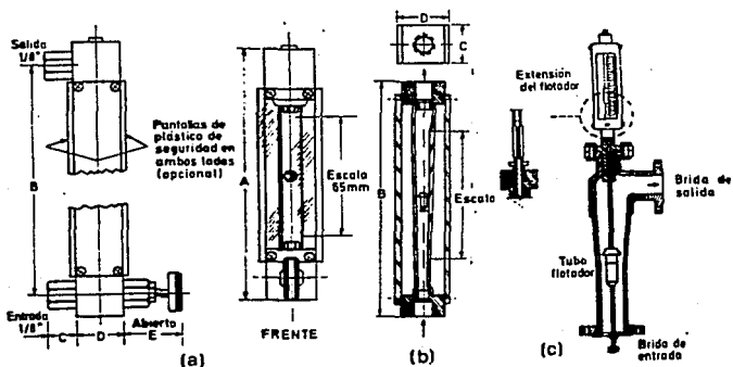
Fig. II.1.2.14 Tipos de rotámetros. a) Purga; b) Indicación directa; c) Armado.
