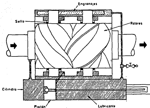
Fig. II.1.2.5 Medidor Birrotor.
