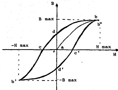
Fig. D.I.1 Ciclo de Histéresis.
