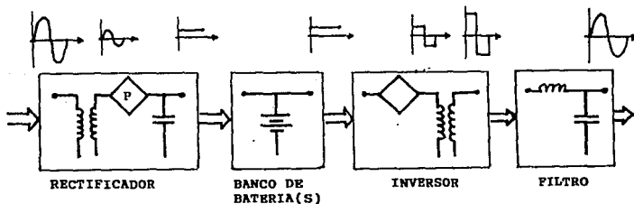
Fig. III.3d.1.1 Diagrama esquemático a bloques de un UPS.
