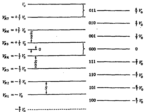
Fig. A.1.2.4 Niveles de referencia y salidas digitales para el convertidor A/D comparador utilizando representación de complemento a dos.
