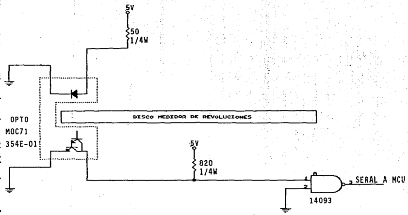
Fig. III.3a.4 Circuito de medición de revoluciones.
