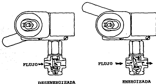
Fig. II.2.1.3 Válvulas solenoides con restablecimiento manual.
