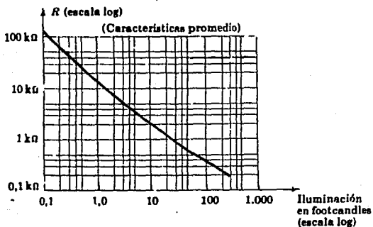
Fig. II.1.1.13 Características de una fotoresistencia.
