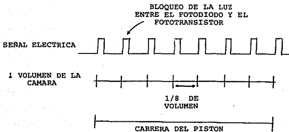
Fig. II.3.6 Gráfica de relación señal de salida contra volumen a medir.
