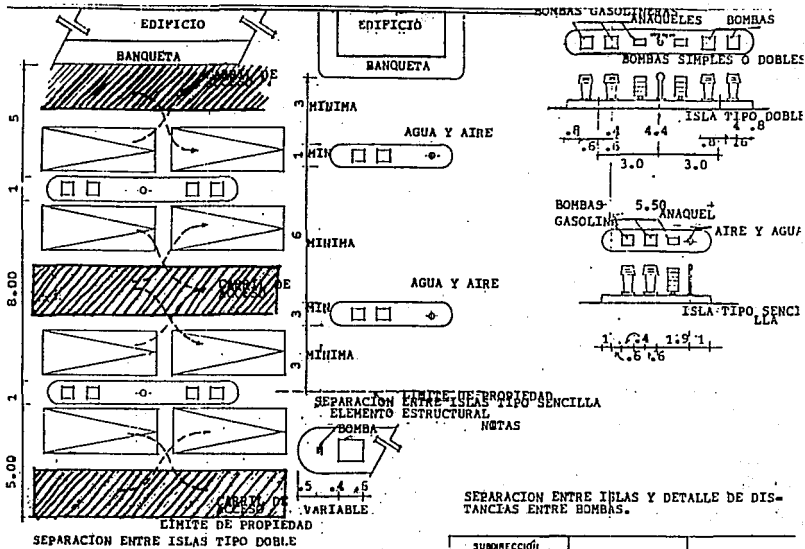
Fig. I.4.1 Ubicación de los surtidores.
