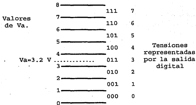
Fig. A.1.2.7 Ejemplo sin el desplazamiento de tensión.
