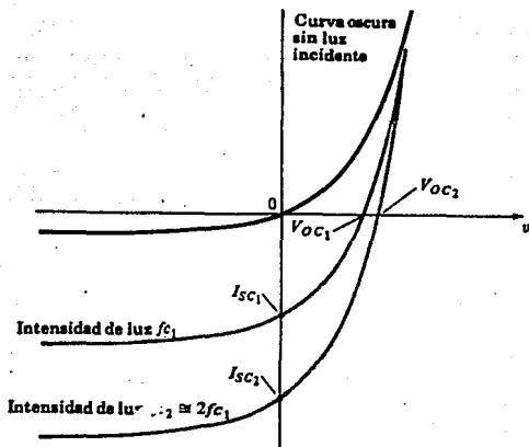
Fig. II.1.1.17 Corriente de corto circuito y voltaje de circuito abierto contra iluminación.
