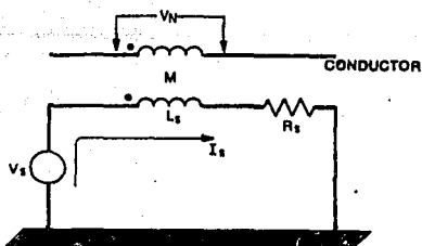
Fig. III.3c.4.9 Circuito equivalente.
