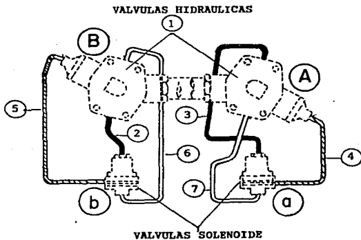
Fig. I.2.2.2 Válvula solenoide para surtidores de succión directa de dos mangueras y un mismo producto.
