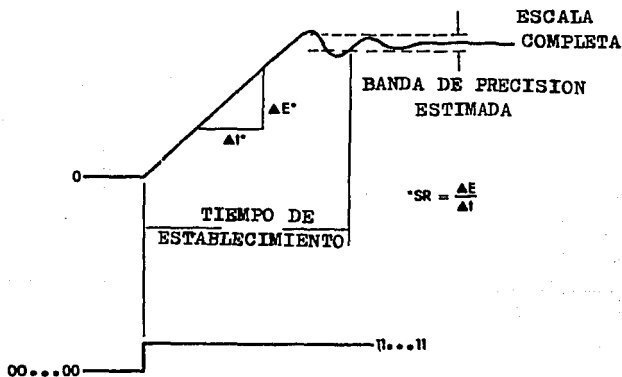
Fig. A.1.3.5 Slew rate y tiempo de establecimiento.
