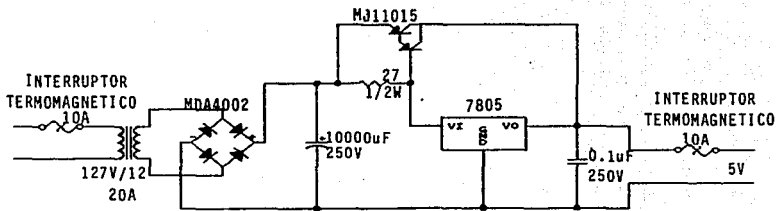
Fig III.3a.9 Fuente de alimentación de 5V.
