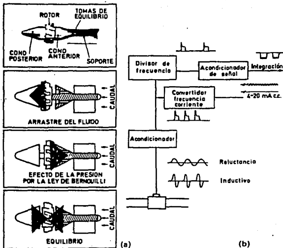
Fig. II.1.2.15 Medidor de turbina. a) Rotor de turbina. b) Diagrama de bloques de la turbina.
