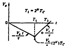
Fig. A.1.2.11 Convertidor A/D de doble rampa.
