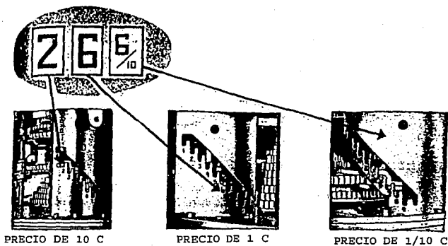
Fig. I.3.4.1 Ubicación de los variadores por ranuras en el computador mecánico.
