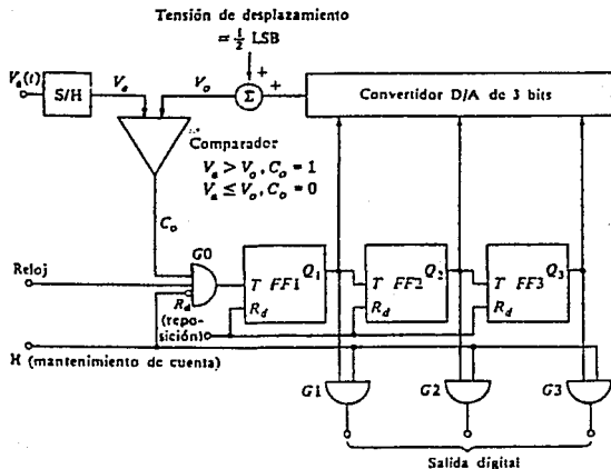
Fig. A.1.2.9 Un convertidor A/D contador de tres bits.
