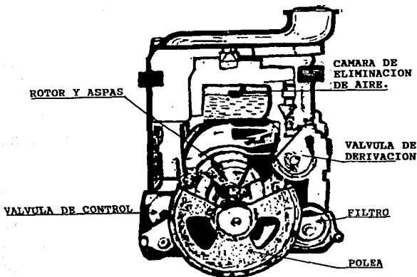
Fig. I.2.1.1 Unidad de bombeo para surtidores de succión directa.
