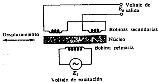
Fig. II.1.1.2 Diagrama esquemático de un transformador diferencial.
