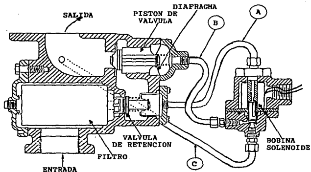
Fig. I.2.1.6 Válvula solenoide para sistemas de control remoto.
