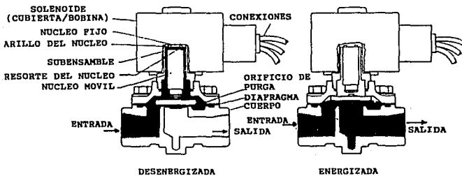
Fig. II.2.1.2 Válvula solenoide pilotadas internamente.
