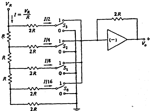
Fig. A.1.1.4 El convertidor D/A con escalera invertida.
