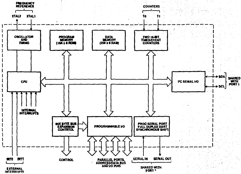
Fig. III.2.1.6 Diagrama a bloques del MCU 83C652.
