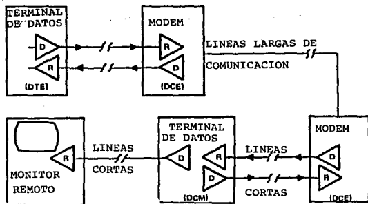
Fig. II.5a.1 Interface entre un equipo terminal de datos (DTE) y un equipo de comunicación de datos (DCE).
