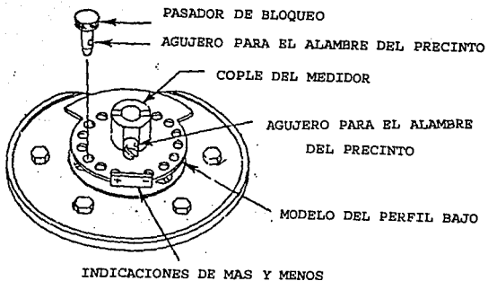
Fig. I.3.1.2 Unidad de calibración del medidor de flujo.
