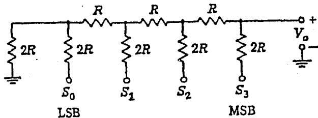
Fig. A.1.1.3 El convertidor D/A en escalera R-2R.
