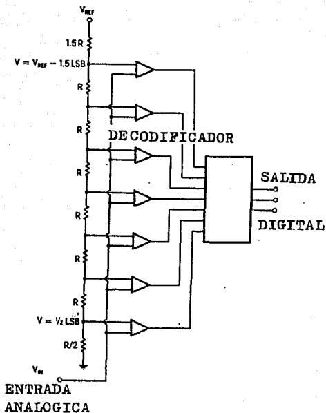
Fig. A.1.2.1 El convertidor A/D comparador.
