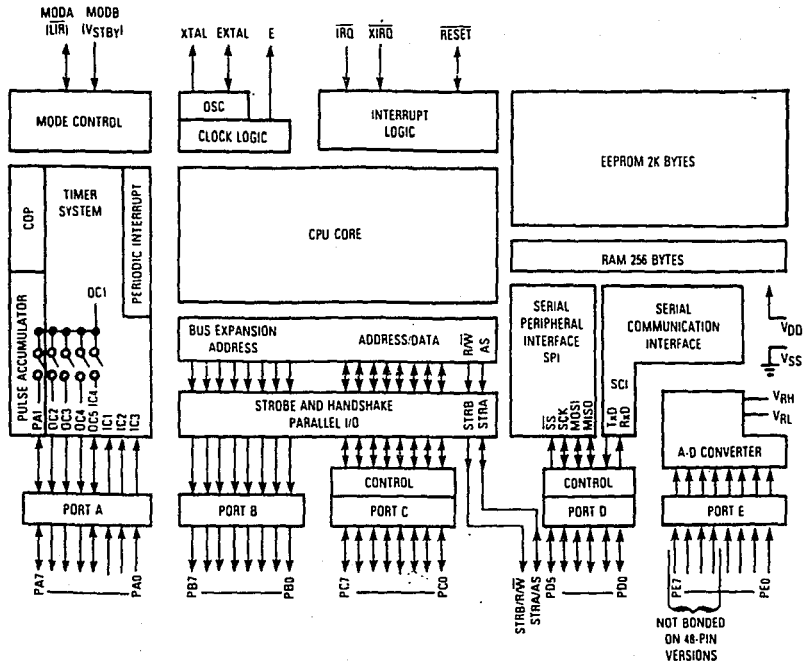
Fig. III.2.3.2 Diagrama a bloques del MCU 68HC811E2.
