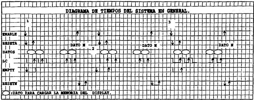
Fig. III.3b.3 Diagrama de tiempos general.
