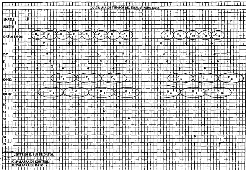
Fig. III.3B.12 Diagrama de tiempos del display numérico.
