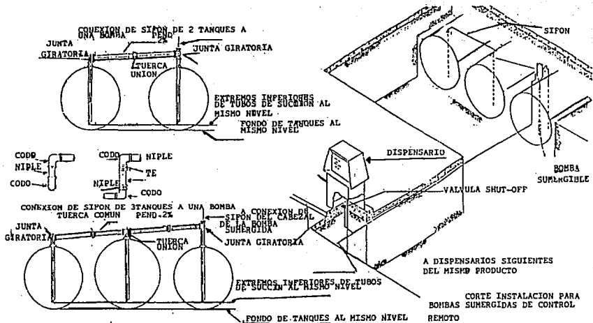
DETALLE DE LA INSTALACION DE TUBERIAS EN SISTEMA DE CONTROL REMOTO
