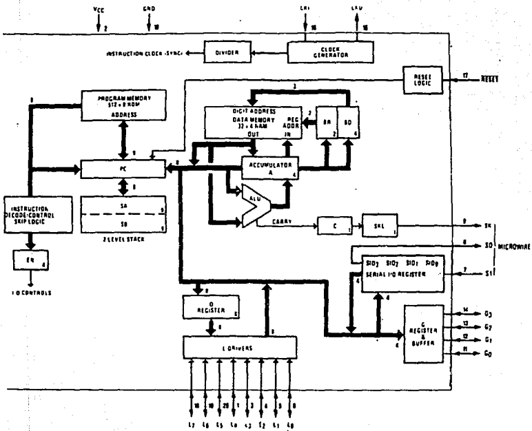
Fig. III.2.2.5 Diagrama a bloques de los siguientes MCU's: COP413L, COP313L.
