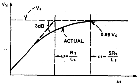
Fig. III.3c.4.10 Comportamiento de V_N contra la frecuencia.
