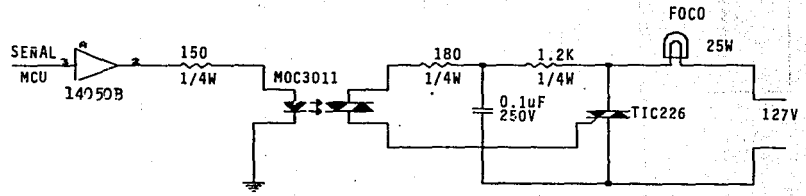
Fig. III.3a.8 Circuito de activación del foco indicador. III - 104
