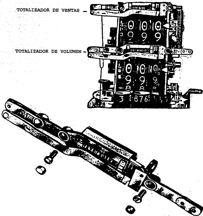
Fig. I.3.5.1 Totalizadores en computador mecánico.
