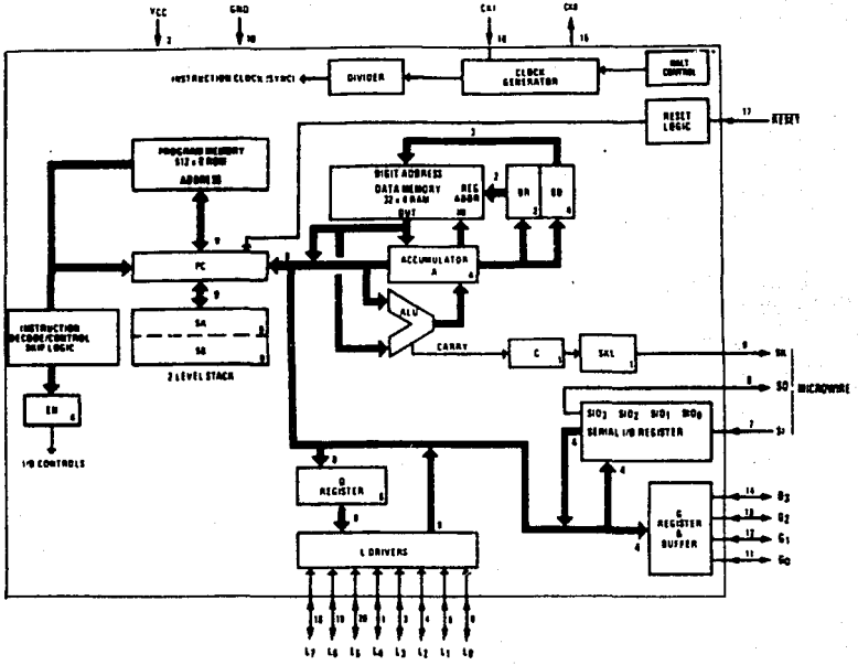
Fig. III.2.2.6 Diagrama a bloques de los siguientes MCU's:
