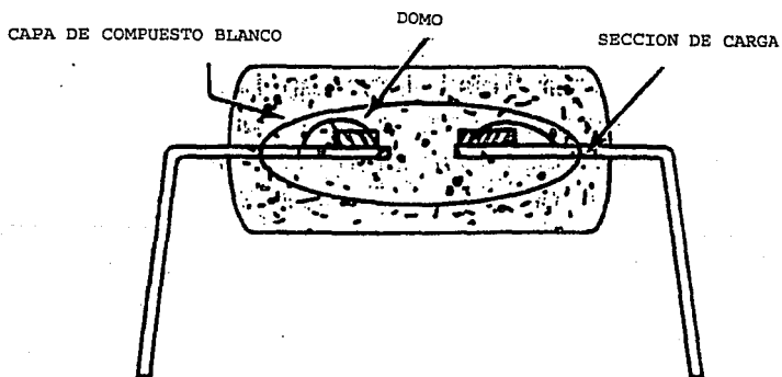
Fig. II.3.1.3 Paquete de aisladores coplanares.
