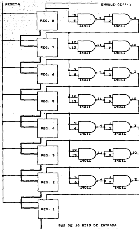
Fig. III.3b.8 Registro de desplazamiento.
