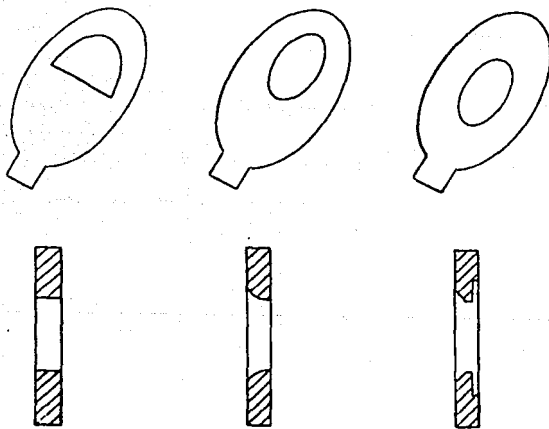
Fig. II.1.2.9 Tipos de orificio.
