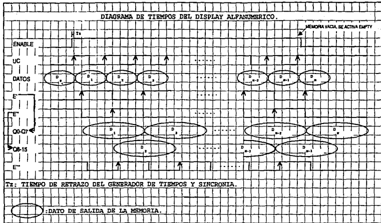
Fig. III.3b.9 Diagrama de tiempos del display alfanumérico.
