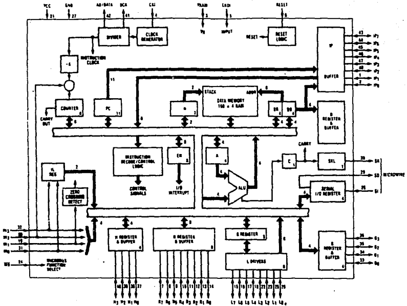
Fig. III.2.2.2 Diagrama a bloques del MCU COP404.
