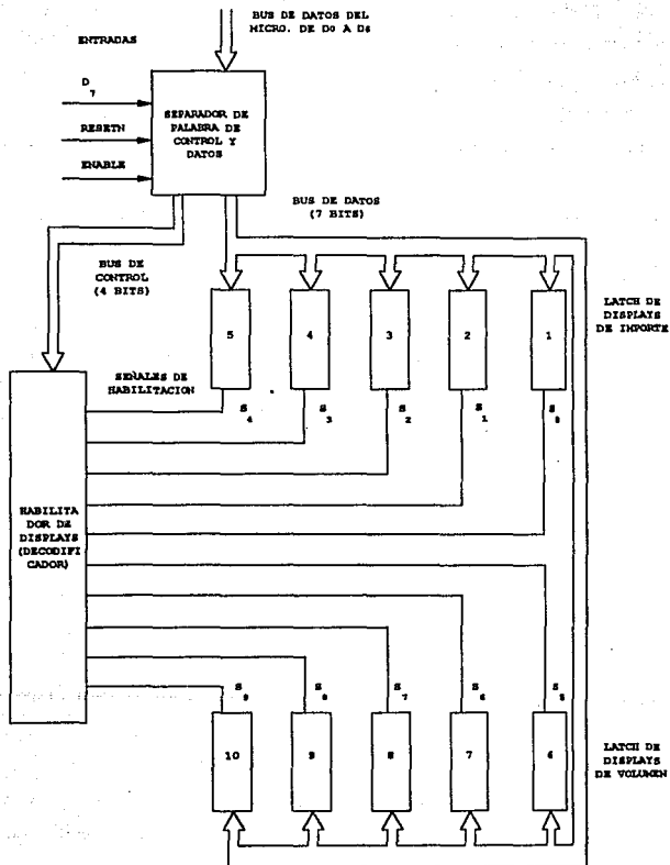
Fig. III.1.10 Diagrama de bloques del display numérico.
