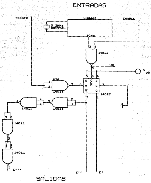
Fig. III.3b.5 Módulo generador de tiempos y sincronía.
