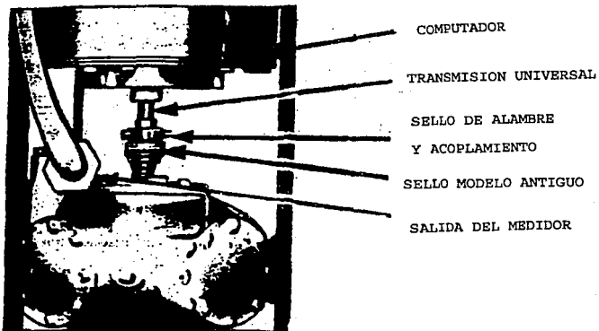
Fig. I.3.3.2 Acoplamiento del medidor de flujo con el computador mecánico.
