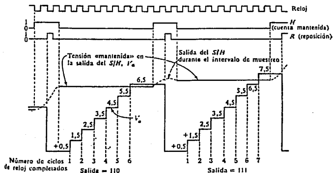
Fig. A.1.2.10 Formas de onda del convertidor contador.
