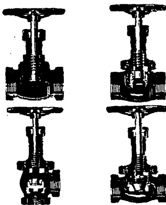
Fig. II.2.3.3 Válvulas de globo.
