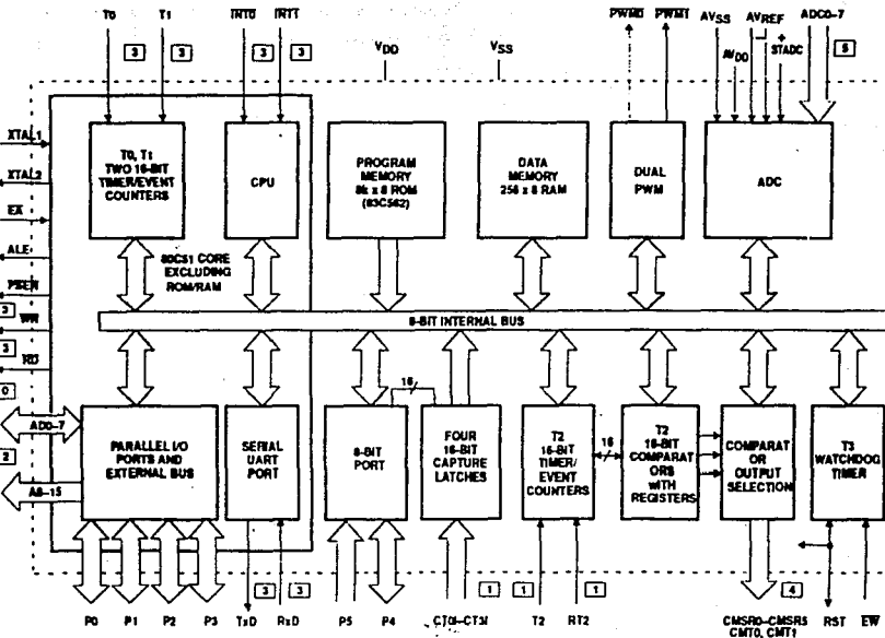
Fig. III.2.1.3 Diagrama a bloques del 83C562.
