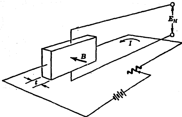
Fig. II.1.1.20 El efecto Hall.
