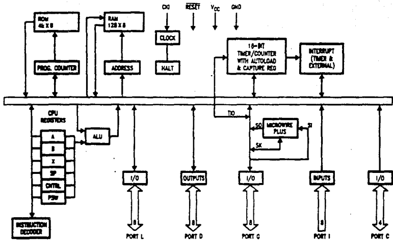
Fig. III.2.2.10 Diagrama a bloques del MCU COP880C.
