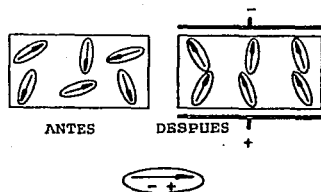
Fig. II.1.1.8 Efecto piezoeléctrico en cerámicas.
