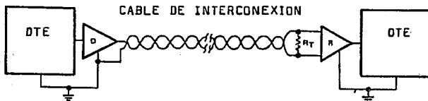
Figura II.5c.1 Configuración básica para una interface digital desbalanceada RS-423-A.
