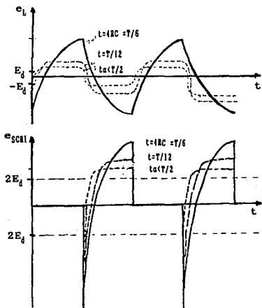
Fig. D.II.2 Formas de onda de un inversor conmutado por capacitor en paralelo.
