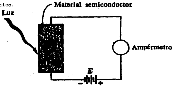
Fig. II.1.1.11 Diagrama esquemático de un transductor fotoconductorivo.
