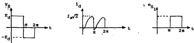
Fig. III.3d.3.1 Inversor controlado por impulso con diodos de retroalimentación.
