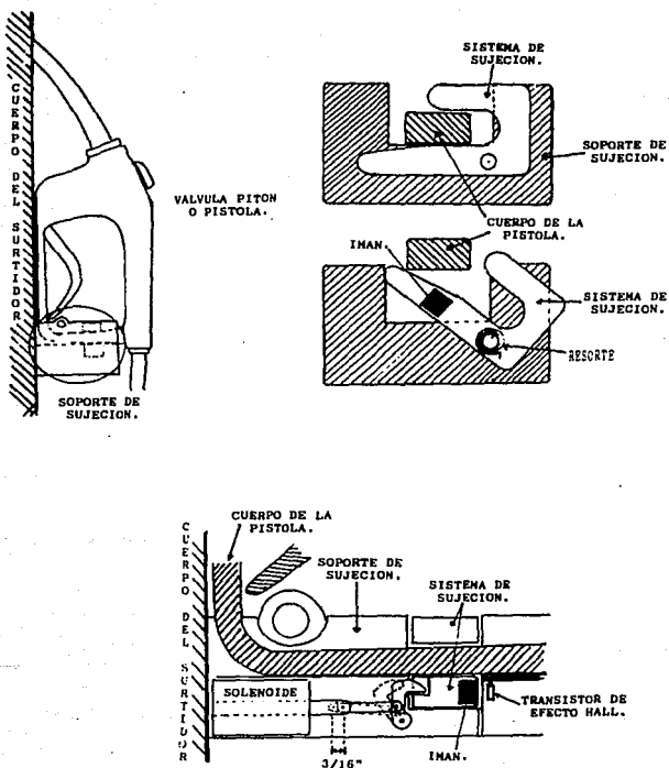
Fig. III.1.6.1 Sistema de sujeción de la pistola o válvula pitón.
