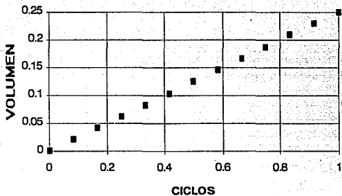
Fig. II.3.12 Característica de volumen contra ciclos por pistón.
