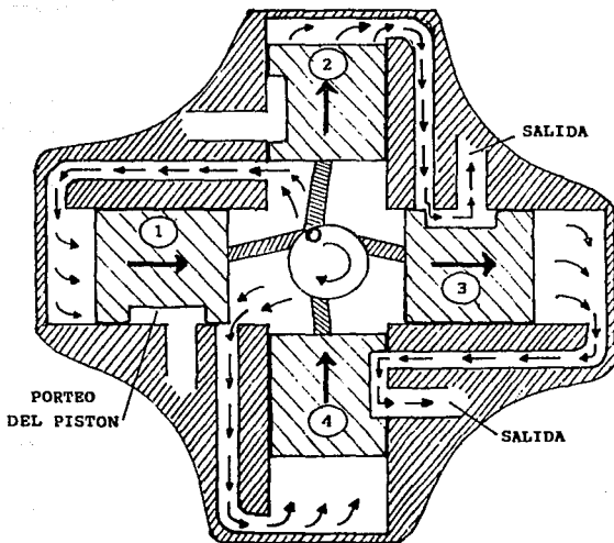
Fig. I.2.2.1 Unidad de medición de los surtidores existentes en el mercado.
