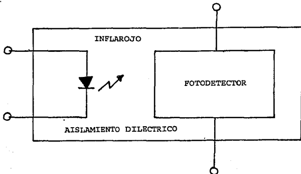
Fig. II.3.1.1 Diagrama de bloques de un optoaislador.
