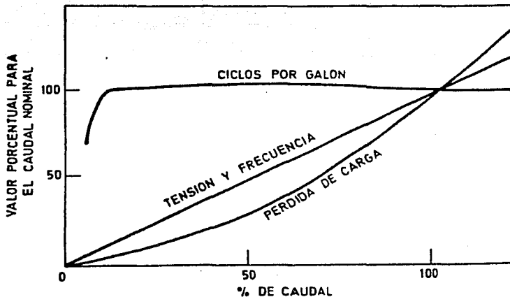
Fig. II.1.2.16 Curvas del medidor de turbina.
