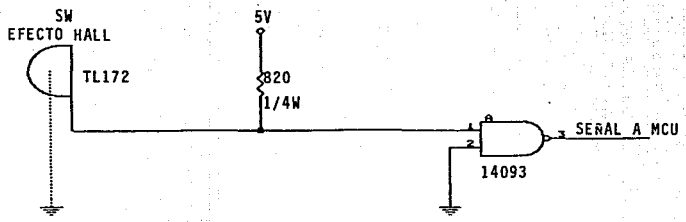
Fig. III.3a.3 Circuito interruptor pistola en su lugar.
