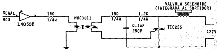
FIG. III.3a.5 Circuito de activación de la válvula solenoide.
