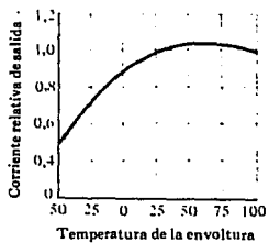
Fig. II.3.1.8 Características típicas optoelectrónicas para cada uno de los canales.
