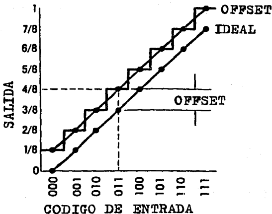
Fig. A.1.3.3 Error de offset.
