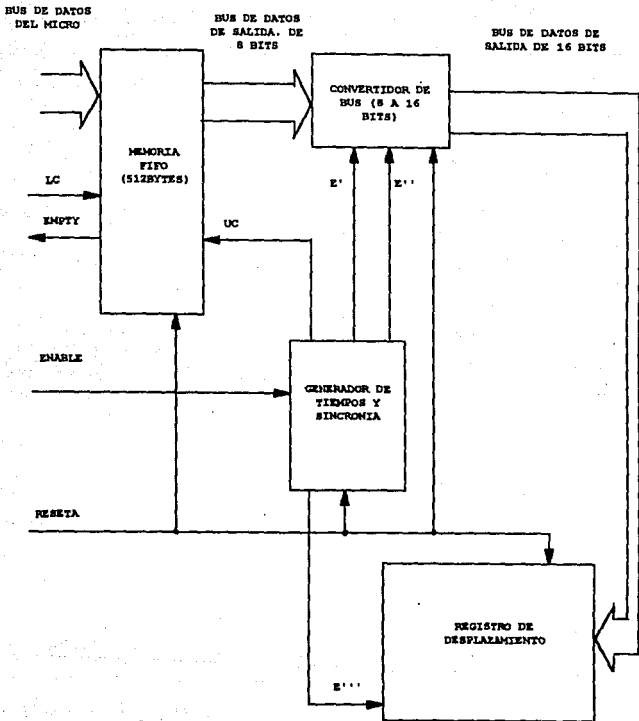
Fig. III.3b.4 Display alfanumérico
