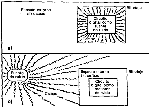
Fig. III.3c.4.1 Blindaje de los circuitos.
