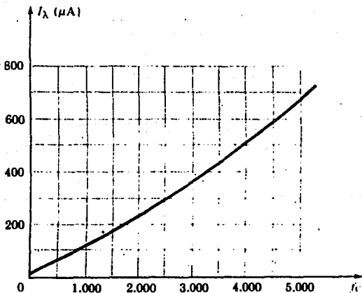
Fig. II.1.1.14 Conjunto de características de un fotodiodo.
