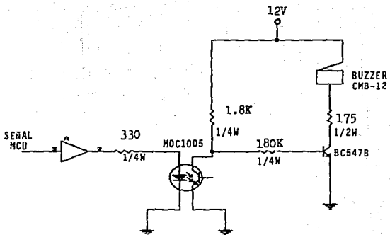
Fig III.3a.1 Circuito de activación del buzzer indicador.
