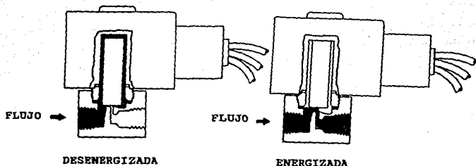
Fig. II.2.1.1 Válvulas solenoide de acción directa.
