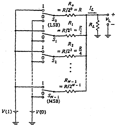
Fig. A.1.1.1 Un convertidor D/A de resistencias ponderadas.
