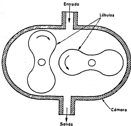
Fig. II.1.2.4 Medidor cicloidal.
