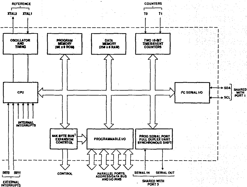
Fig. III.2.1.7 Diagrama a bloques del MCU 83C654.
