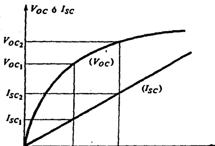
Fig. II.1.1.16 Corriente contra voltaje en una fotocelda.
