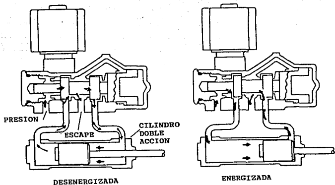
Fig. II.2.2.2 Válvulas de cuatro vías.
