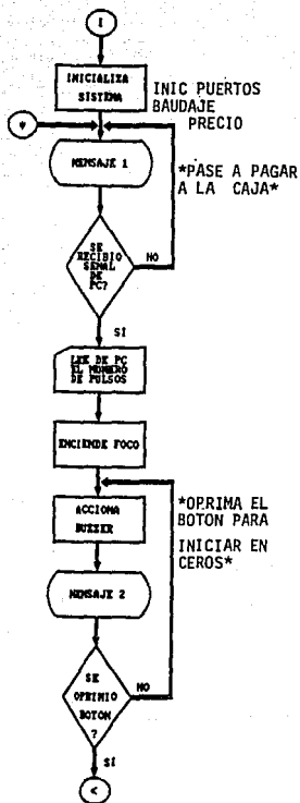
Fig. III.3.1 Diagrama de flujo del proceso de suministro (I).
