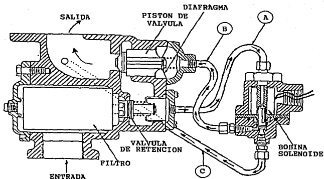
Fig. II.2.5.3 Ensamble de válvula solenoide y filtro.
