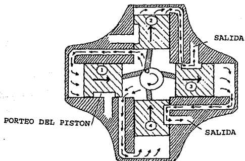
Fig. I.3.1.3 Circulación del líquido por el medidor de flujo.
