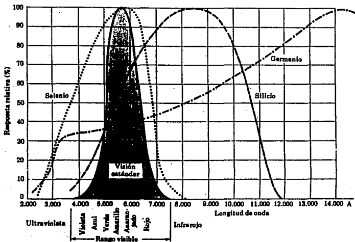
Fig. II.1.1.12 Respuesta de algunos semiconductores a distintas longitudes de onda.
