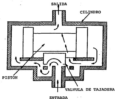
Fig. II.3.1 Medidor de pistón convencional.
