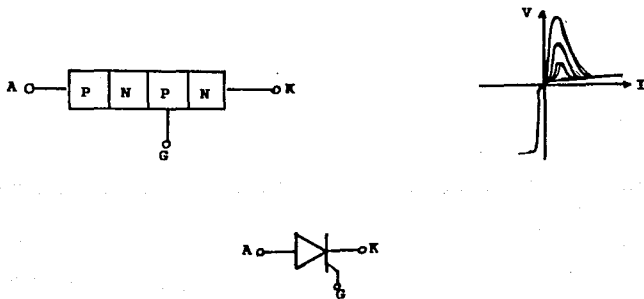
Fig III.3d.2.1 Estructura de un SCR.
