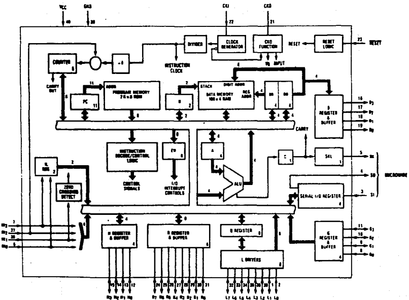
Fig. III.2.2.3 Diagrama a bloques de los siguientes MCU'S: COP440, COP441, COP442, COP340, COP341, COP342.
