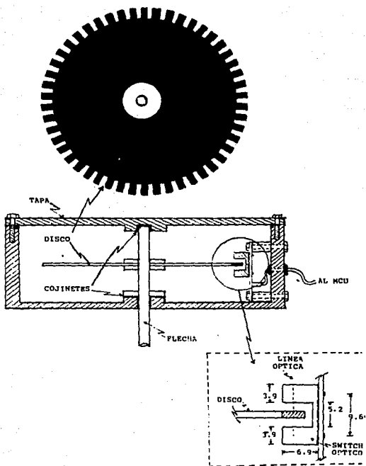
Fig. III.1.3.1 Transductor de la unidad de medición.
