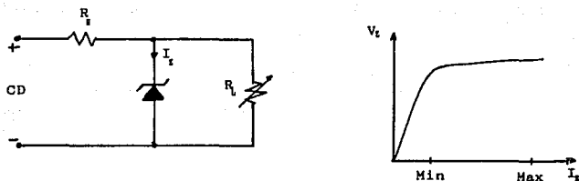
Fig. D.I.4 Circuito regulador de diodo Zener.
