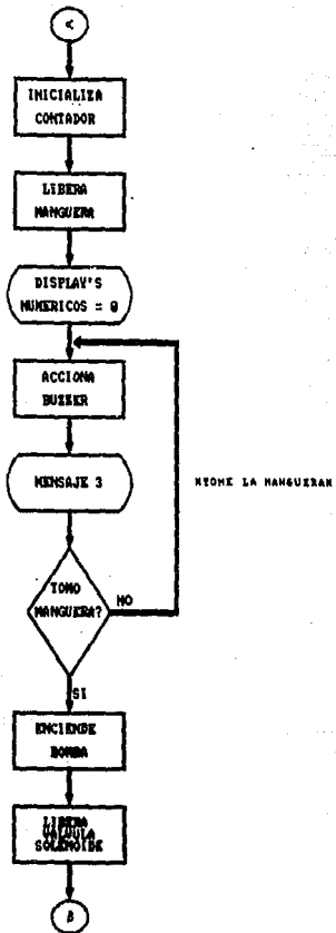
Fig. III.3.2 Diagrama de flujo del proceso de suministro (II).
