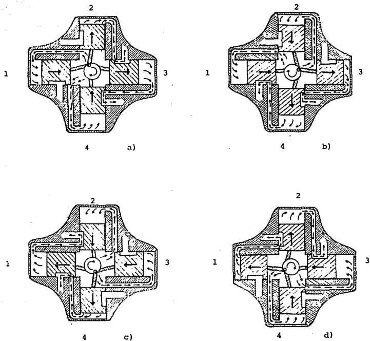
Fig. II.3.9 Secuencia del funcionamiento del medior de cuatro pistones.
