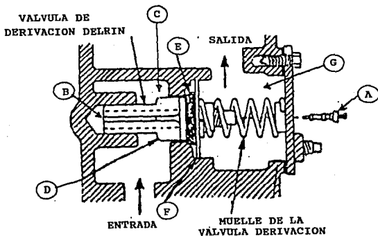
Fig. II.2.4.1 Válvula de control.
