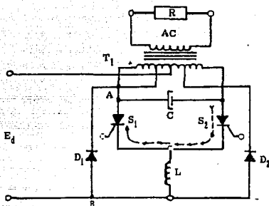
Fig. D.II.6 Inversor conmutado por impulso, modificado con capacitor en paralelo.
