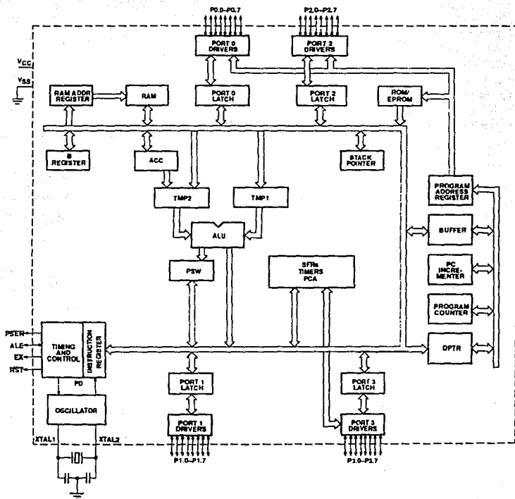
Fig. III.2.1.1 Diagrama a bloques del MCU 80C51.
