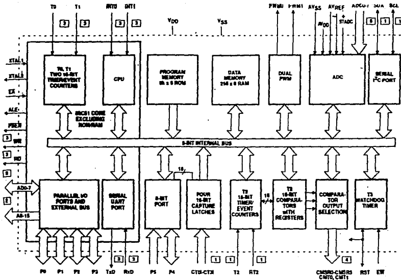
Fig. III.2.1.2 Diagrama a bloques del MCU 83C552.
