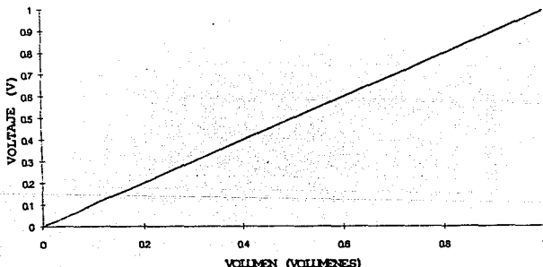
Fig. II.3.4 Característica ideal del medidor de flujo usando un LVDT.
