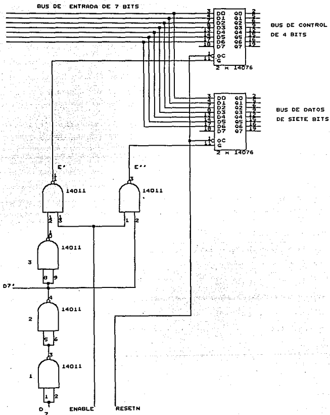
Fig. III.3b.11 Separador de bus.
