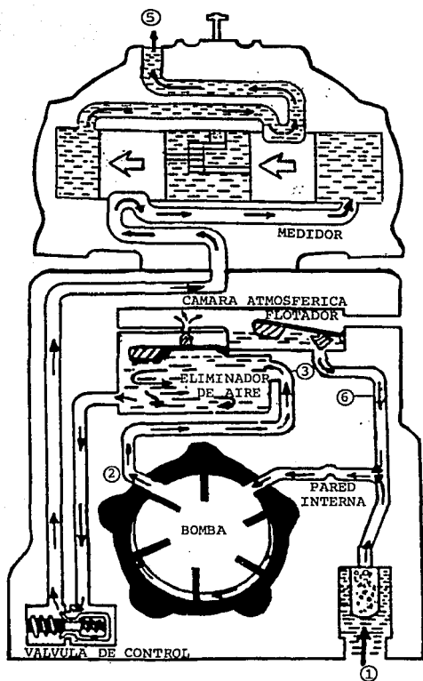
Figura I.1.2 Flujo esquemático de la gasolina.
