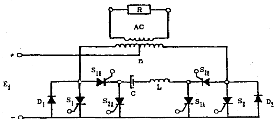
Inversor conmutado por impulso con transformador de acoplo.
