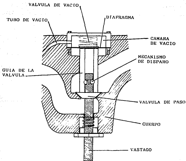
Fig. II.2.5.4 Válvula pitón o pistola.
