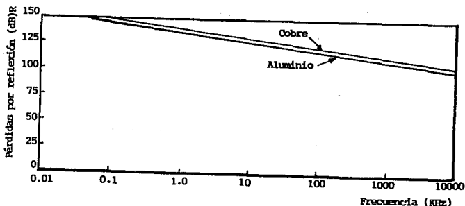
Fig. III.3c.4.6 Pérdidas por reflexión.
