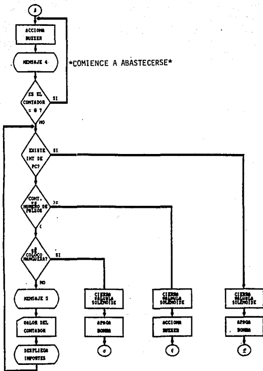
Fig. III.3.3 Diagrama de flujo del proceso de suministro (III).
