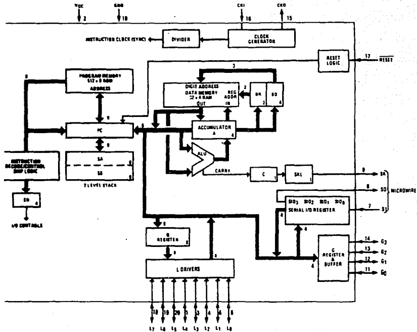
FIG. III.2.2.7 Diagrama a bloques del MCU COP414L.
