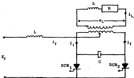
Fig. D.II.1 Inversor conmutado por capacitor en paralelo.
