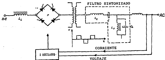
III.3d.3.2 Inversor de onda cuasi-cuadrada con filtro conformador.
