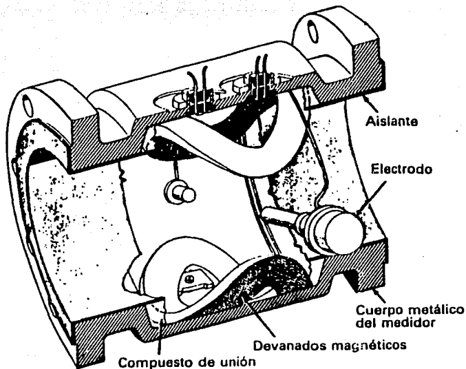
Fig. II.1.2.19 Diagrama básico de un medidor de flujo magnético.
