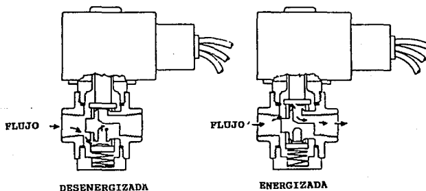
Fig. II.2.2.1 Válvula solenoides de tres vías.
