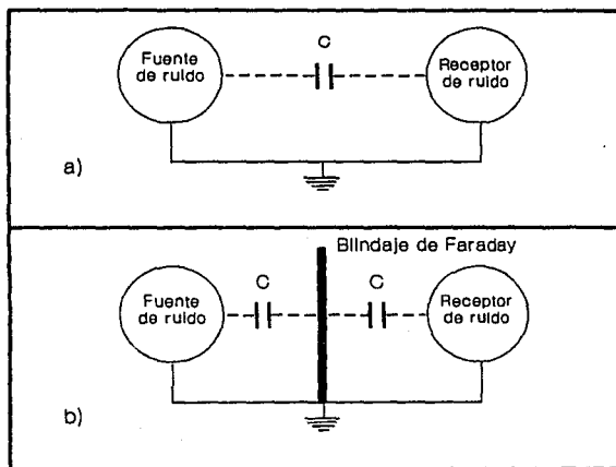
Fig. III.3c.4.8 Blindajes de tipo electrostático.
