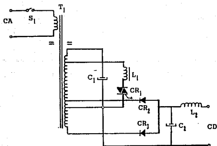
Fig. D.I.3 Circuito ferrosnante controlado.
