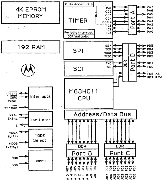
Fig. III.2.3.6 Diagrama a bloques del MCU 68HC711D3.
