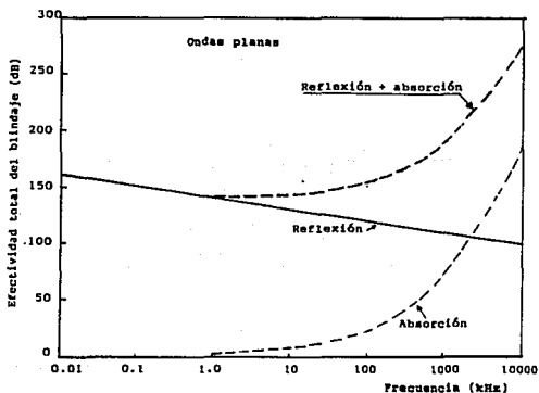
Fig. III.3c.4.7 Efectividad total del blindaje como una función de la frecuencia.
