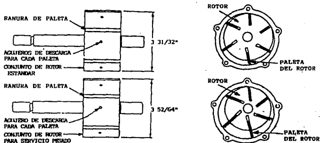
Fig. I.2.1.3 Diferencia entre las unidades de bombeo estándar y de servicio pesado.
