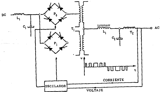
Fig. D.II.7 Inversor modulado por anchura de pulso.
