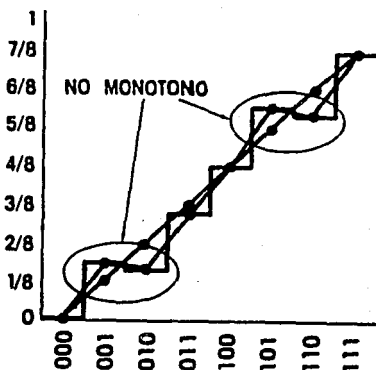
Fig. A.1.3.2 Monotonicidad.
