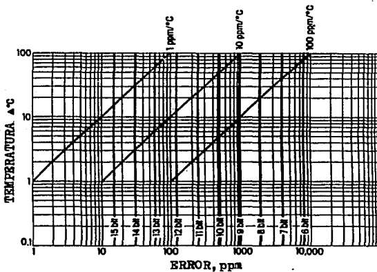
Fig. A.1.3.4 Rangos de cambios de temperatura para varias precisiones.
