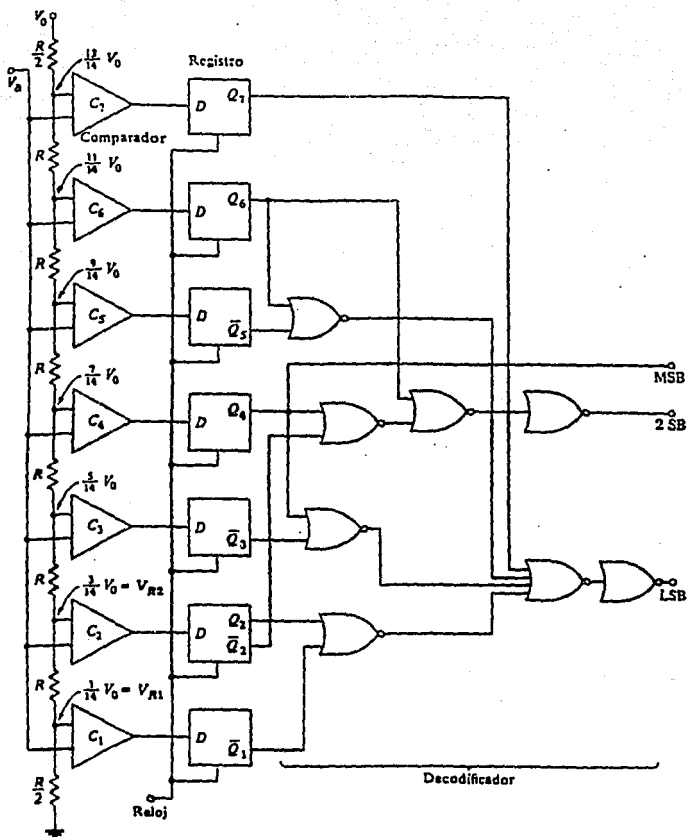
Fig. A.1.2.2 Un convertidor A/D comparador de tres bits.
