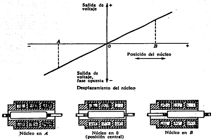
Fig. II.1.1.3 Características de un LVDT.
