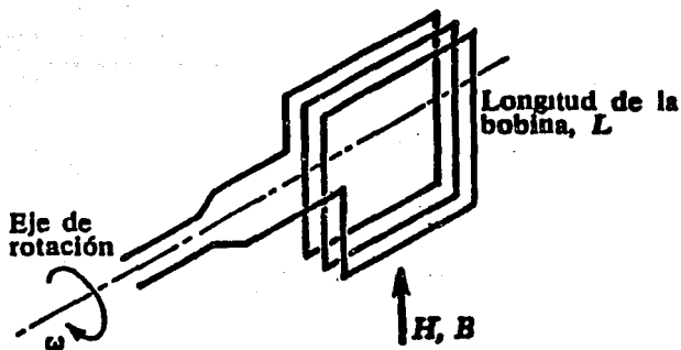
Fig. II.1.1.19 Generador eléctrico.
