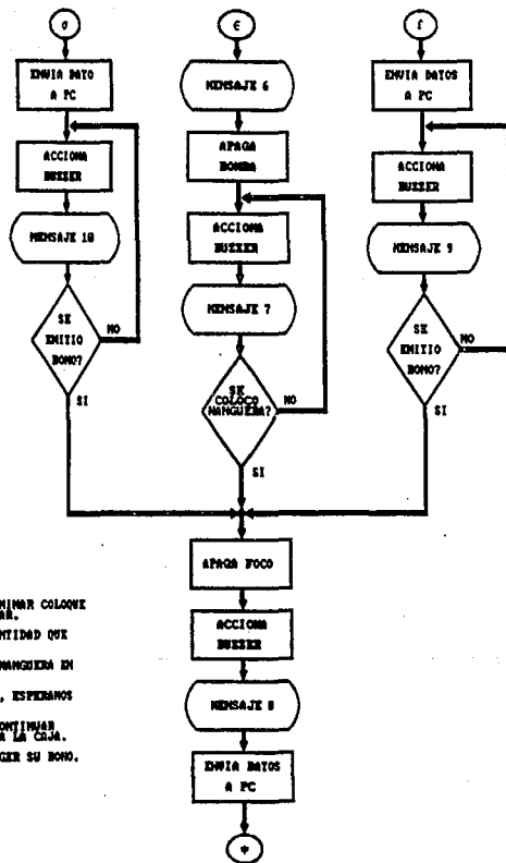
Fig. III.3.4 Diagrama de flujo del proceso de suministro (IV).
