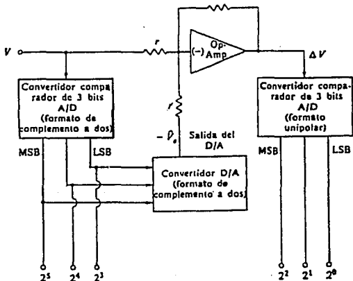
Fig. A.1.2.5 Un convertidor A/D de 6 bits que comprende una cascada de dos convertidores A/D comparadores de tres bits.
