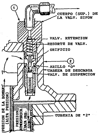
Fig. II.2.5.2 Válvula sifón.
