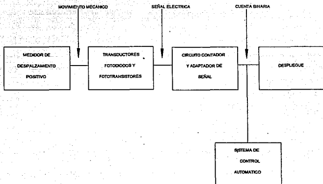
Fig. II.3.5 Diagrama de bloques del sistema de medición completo.
