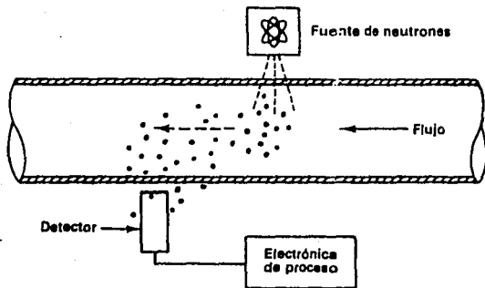
Fig. II.1.2.20 Método de flujo nucleónico.
