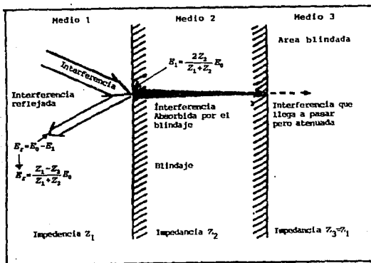
Fig. III.3c.4.5 Componentes en las señales en las pérdidas por reflexión.
