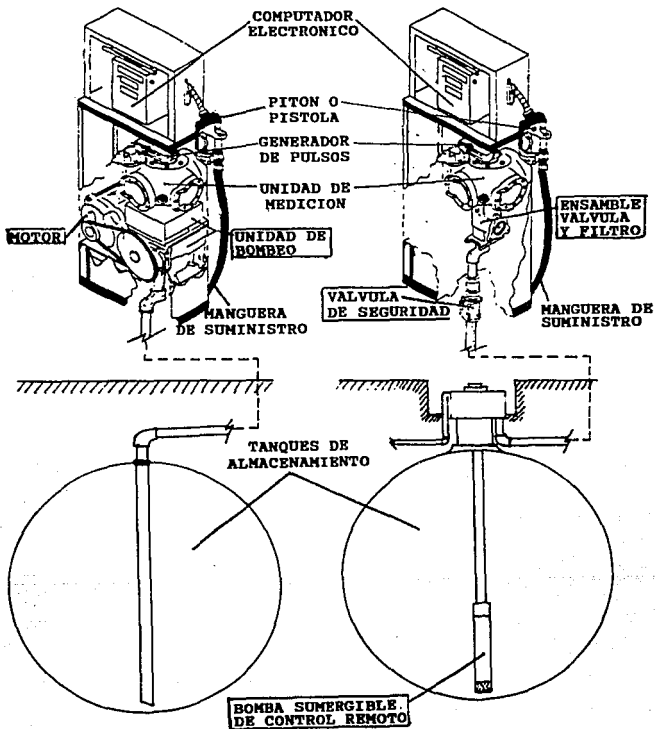
Fig. I.2.1 Surtidor de succión directa y de control remoto.
