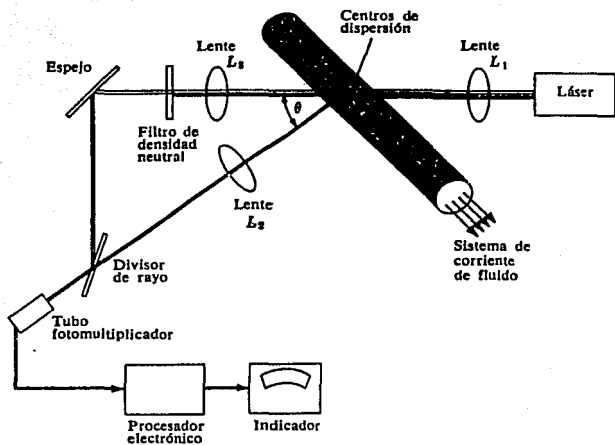
Fig. II.1.2.22 Esquema de un sistema de anemómetro láser para medición de flujo.
