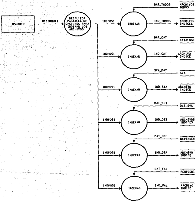
DIAGRAMA DE FLUJO DE DATOS DEL MODULO DE INDEXAR
