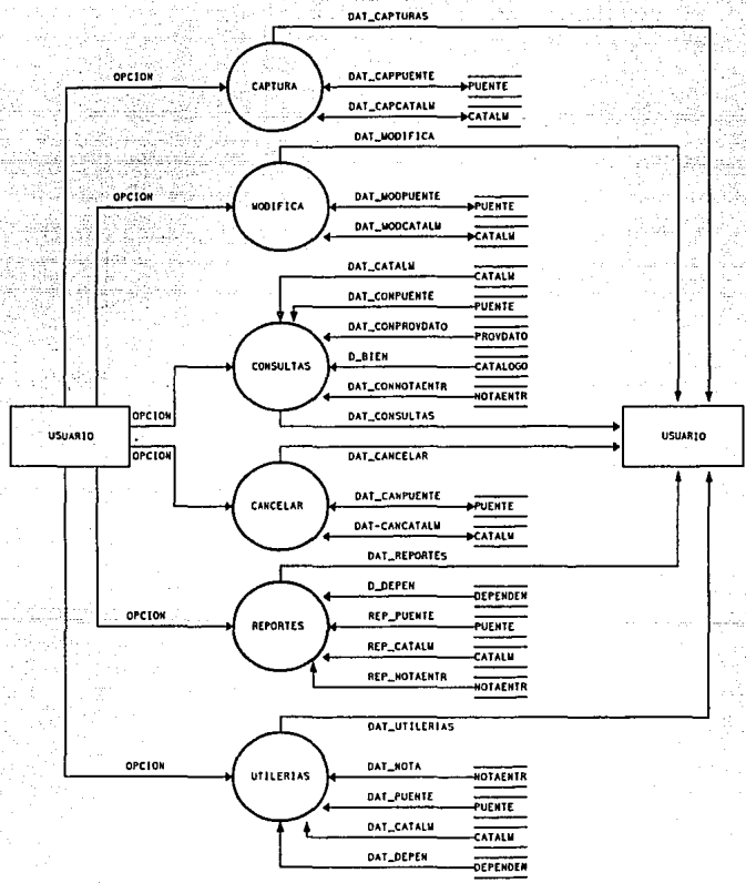
DIAGRAMA DE FLUJO DE DATOS DEL MODULO DE SALIDAS
