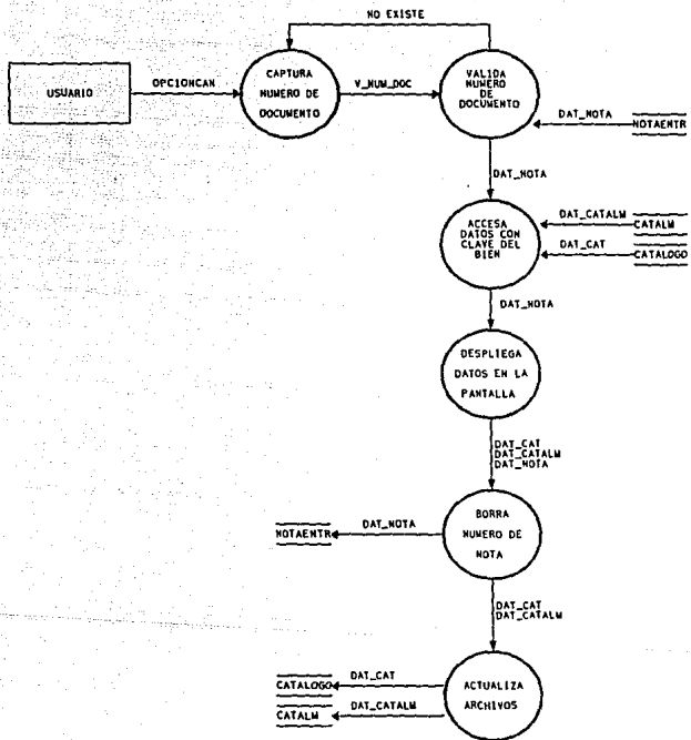
DIAGRAMA DE FLUJO DE DATOS DE CANCELAR REABASTECIMIENTO
