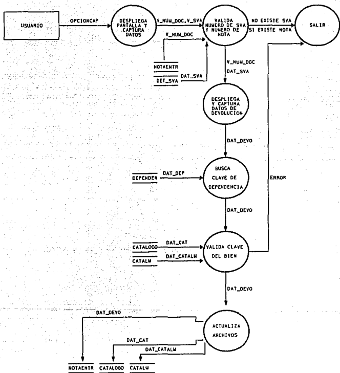
DIAGRAMA DE FLUJO DE DATOS DE CAPTURAS DE DEVOLUCION
