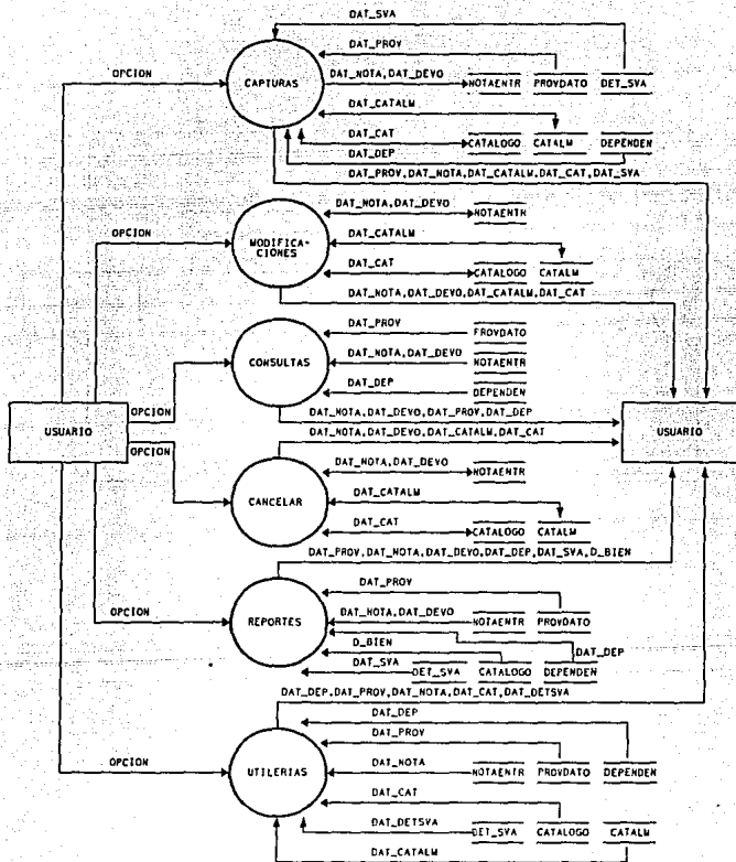
DIAGRAMA DE FLUJO DE DATOS DEL MODULO DE ENTRADAS
