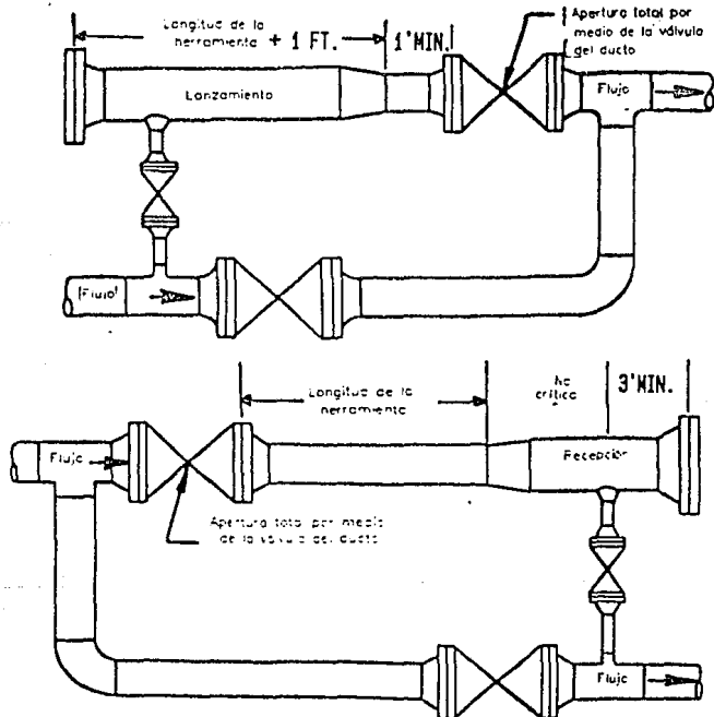
Figura 7.7 Funcionamiento del diablo vetcolog.
