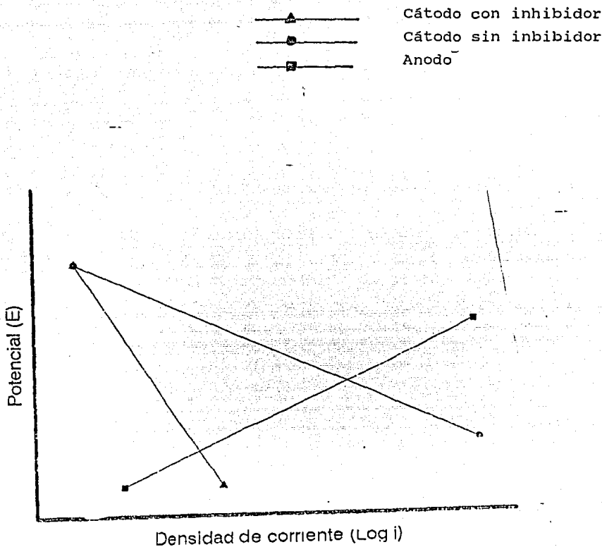
Figura 6.2 Influencia de los inhibidores catódicos en la i_c de corrosión.
