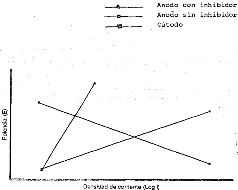
Figura 6.1 Influencia de los inhibidores anódicos en la i de corrosión.
