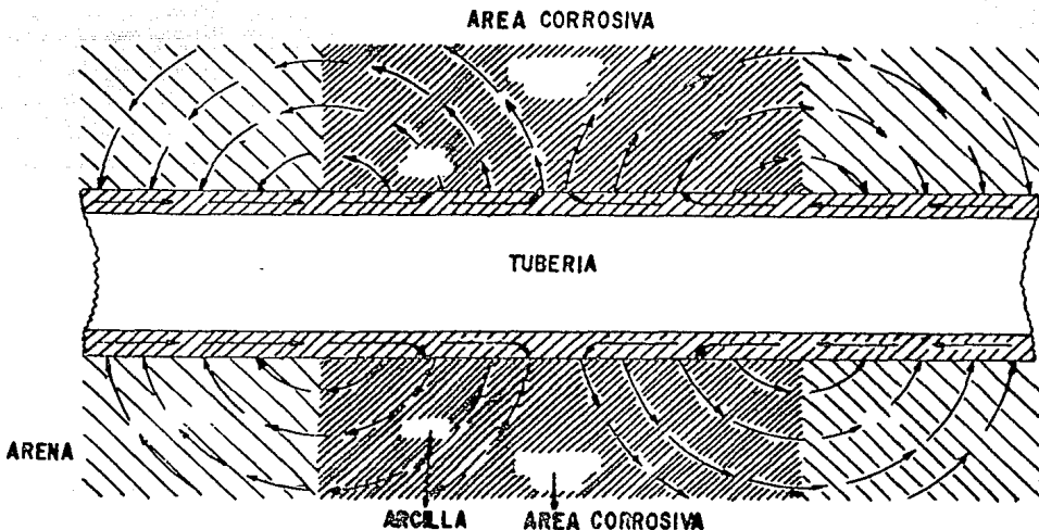
Figura 3.4 Corrosión causada cuando la tubería atraviesa suelos diferentes.
