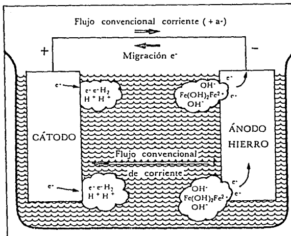
Figura . 2.2. Movimiento de electrones del ánodo al cátodo.
