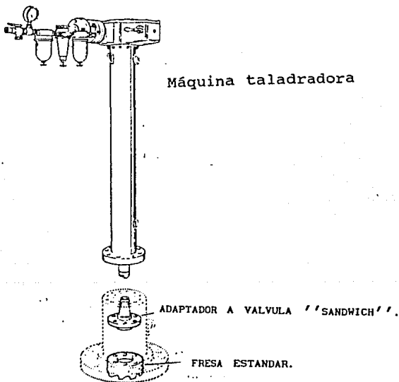
Figura 10.4 Máquina taladradora.
