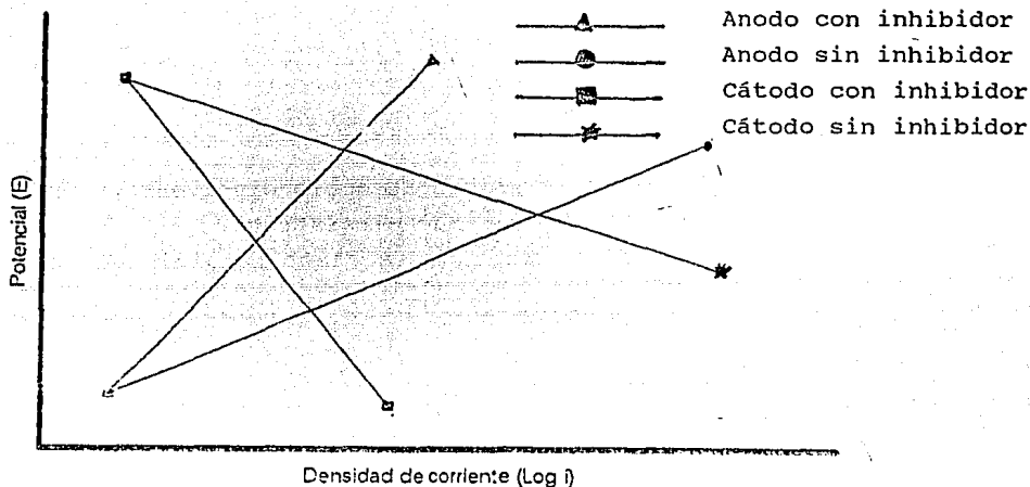
Figura 6.3 Disminución de la corrosión con inhibidores formadores de película orgánica.
