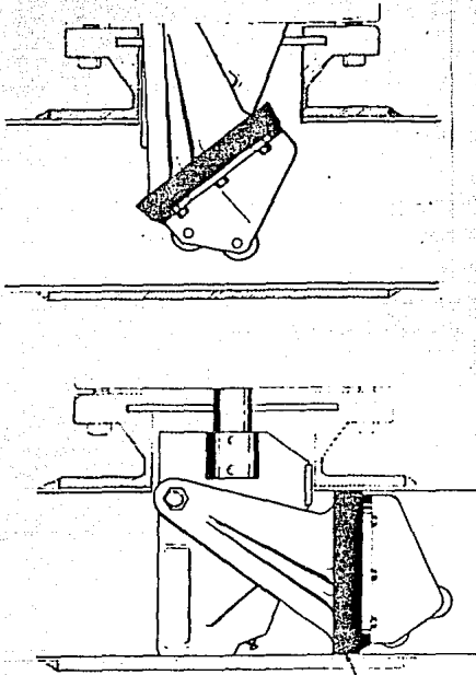
Figura 10.7 Máquina de obturar "stopples".
