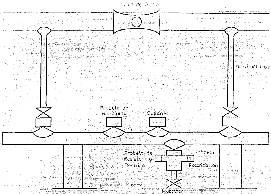
Figura 6.4 Estación de medición de corrosión en la tubería de la línea de gas.
