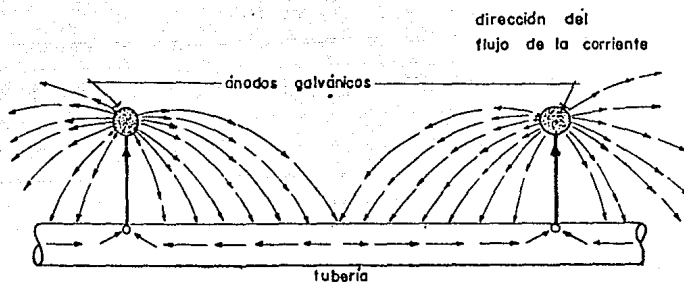
Figura 5.4 Sistema de protección catódica por medio de ánodos galvánicos.
