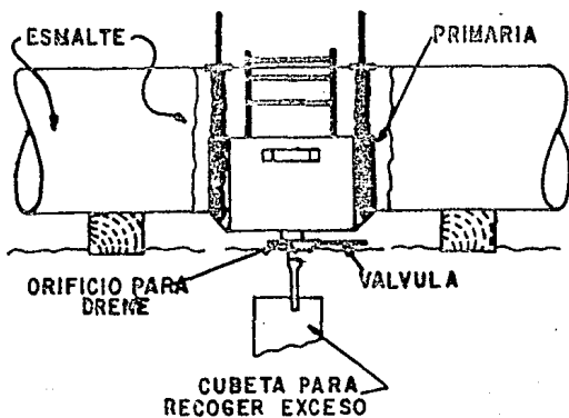
Figura 4. 12 Recubrimiento de coples mecánicos.
