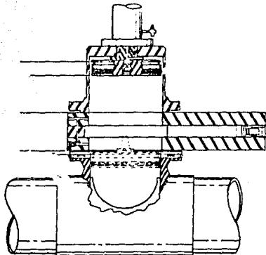
Figura 10.10 Colocación del tapón "lock-o-ring".
