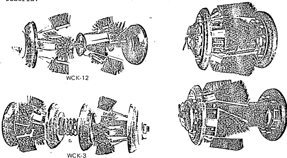
Figura 7.3 Dispositivo de limpieza de cepillo de alambre para tuberías menores.
