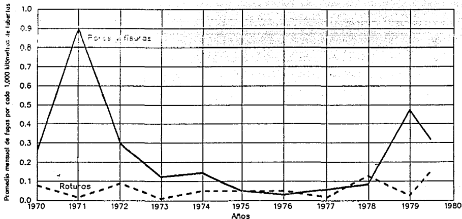
Figura 9.9 Fugas en tuberías en operación en el período comprendido entre 1970 y 1980.
