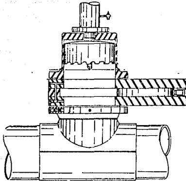
Figura 10.5 Sección de la tubería mostrando la fresa en posición de taladro terminado.
