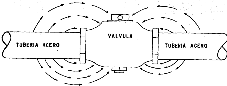
Figura 3.2 Corrosión causada por la diferencia de materiales.
