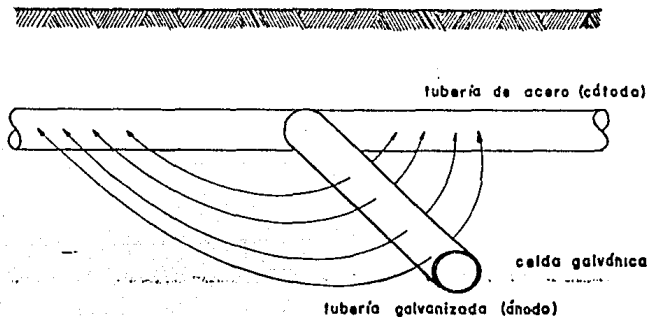
Figura 5.1 Tubería en estado catódico.
