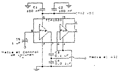
Diagrama 9 Preamplificador del Microfono.
