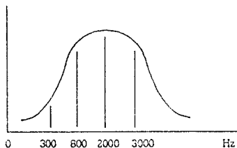
Fig. 2. Ancho de Banda del Canal Telefónico.
