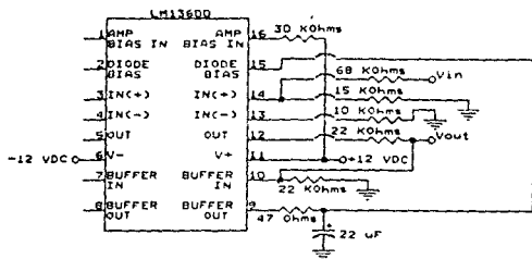
Diagrama 11. Control Automático de Ganancia.
