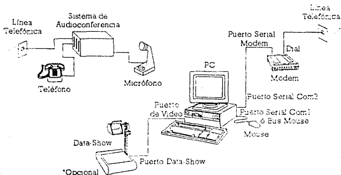
Diagrama 18. Conexión del Sistema Audiográfico.
