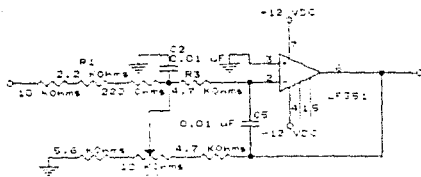
Diagrama 3. Control de Tono
