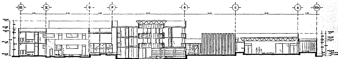
CORTE TRANSVERSAL Y-Y' ESC. 1 : 100
