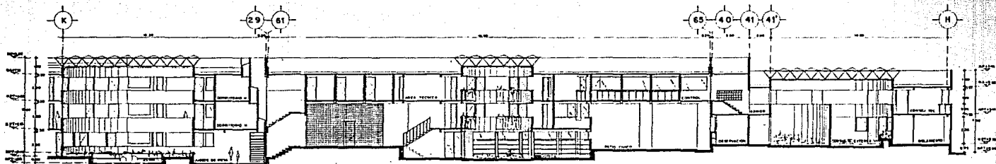
CORTE LONGITUDINAL X-X' ESC. 1 : 100
