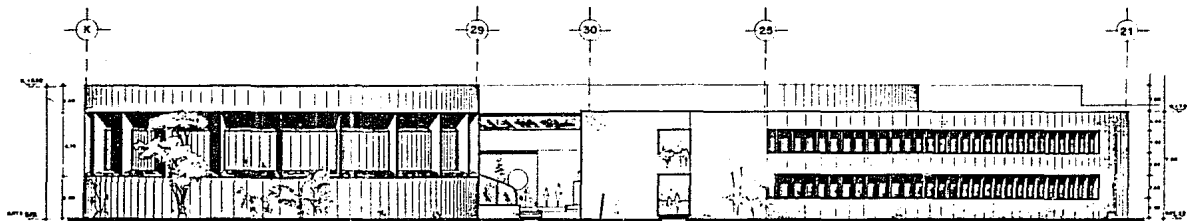
FACHADA POSTERIOR NOROESTE ESC. 1 : 100
