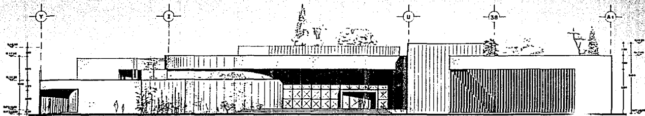
FACHADA PRINCIPAL SUR ESC. 1 : 100
