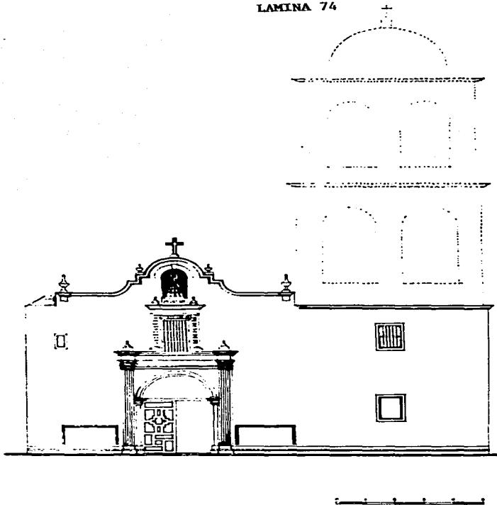
ALZADO PRINCIPAL DE LORETO
