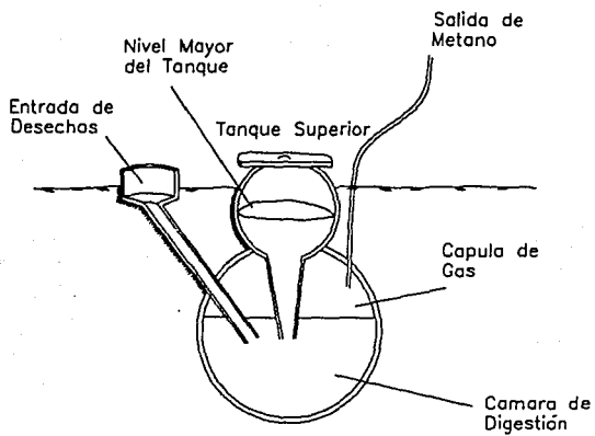
Fig. 11 Fermentador Chino
