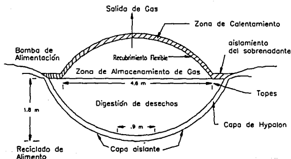
Fig. 5 Reactor de Flujo de Tapa
