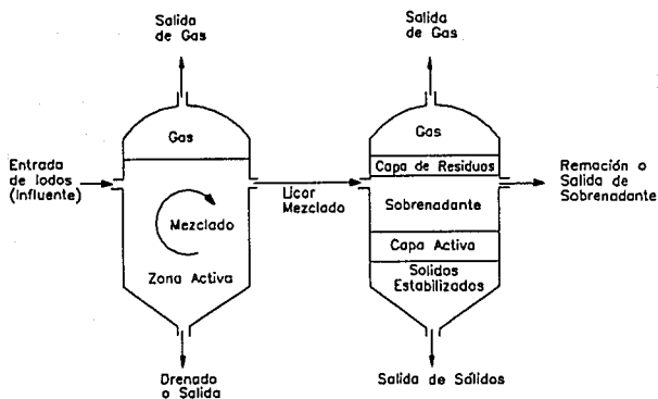
Fig. 7 Digestión Anaerobia en 2 Etapas
