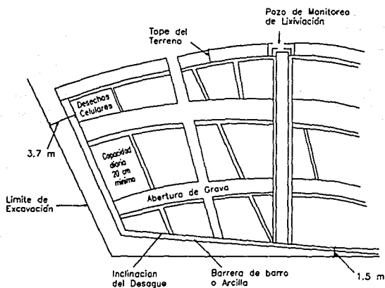
Fig. 2 Fosa Séptica
