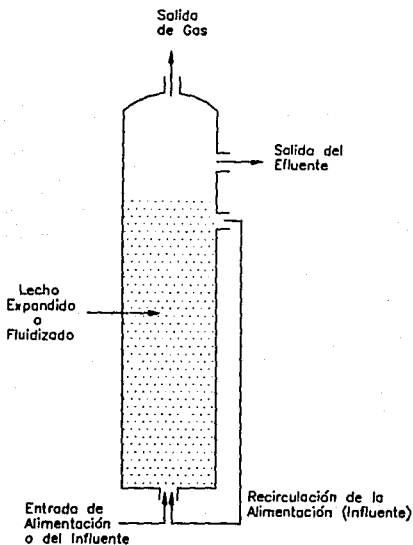
Fig. 10 Reactor de Lecho Expandido y de Masa Fija
