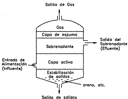
Fig. 3 Digestor convencional de una etapa
