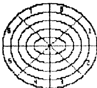
Fig. 4.1 PAQUETE DE DISCOS DIVIDIDO EN SECTORES
