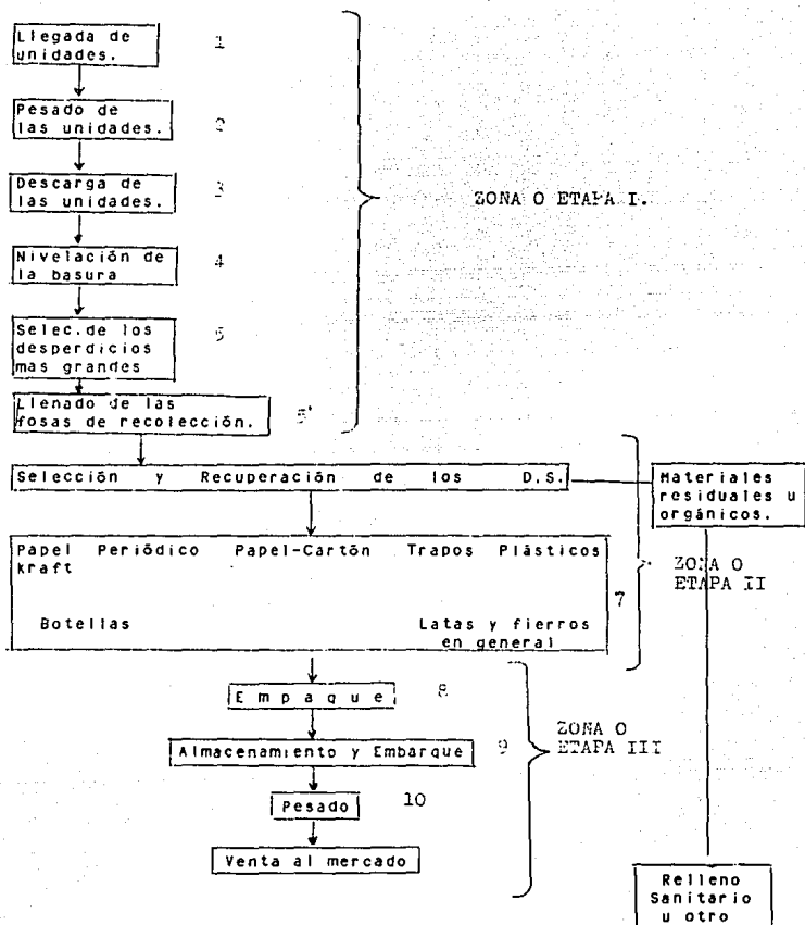
Diagrama General del Proceso.
