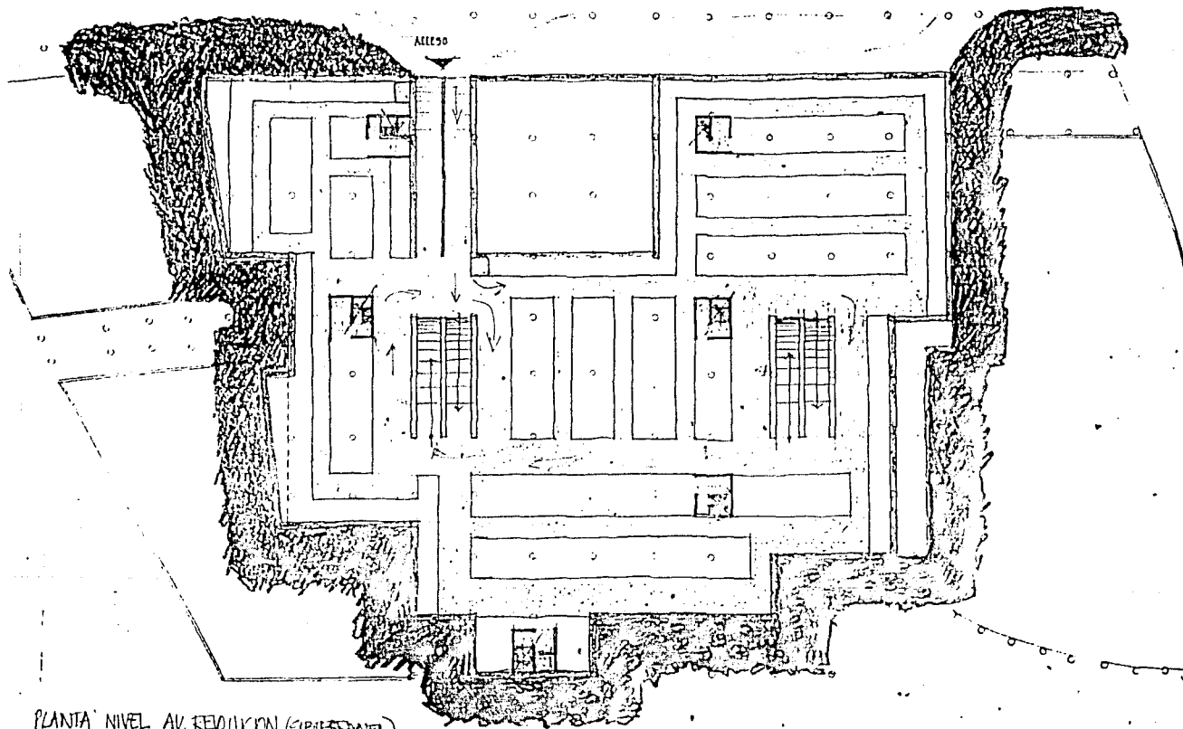
PLANTA NIVEL AV. REVOLUCION (SUBTERRANEA) ESTACIONAMIENTO
