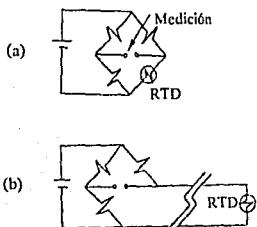
Fig. IV.15 Conexiones de sensores RTD
