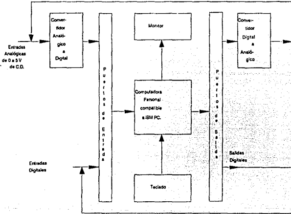
Fig. VI.2 Diagrama de Bloques General del Simulador.
