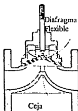
Fig. IV.43 Válvula de Diafragma
