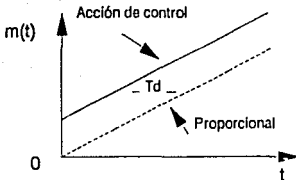
Fig. III.8b Diagrama de Salida de un Control P.D.
