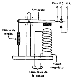
Fig. IV.48 Partes esenciales de un relevador
