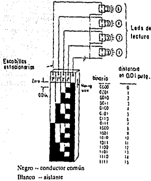
Fig. IV.11 Transductor digital de desplazamiento
