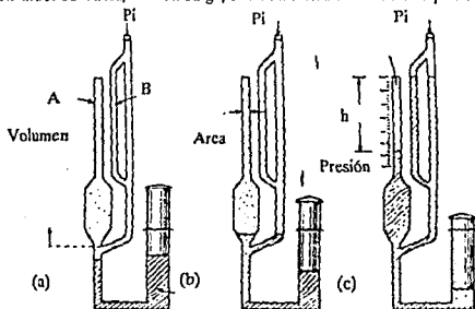
Fig. IV.32 Medidor de McLeod
