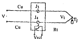
Fig. IV.13 Compensación por software
