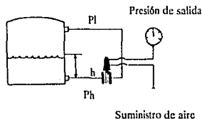
Fig. IV.39 Medidor de Presión Diferencial
