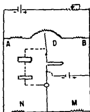
Fig. IV.22 Potenciómetro con compensación de juntura fría
