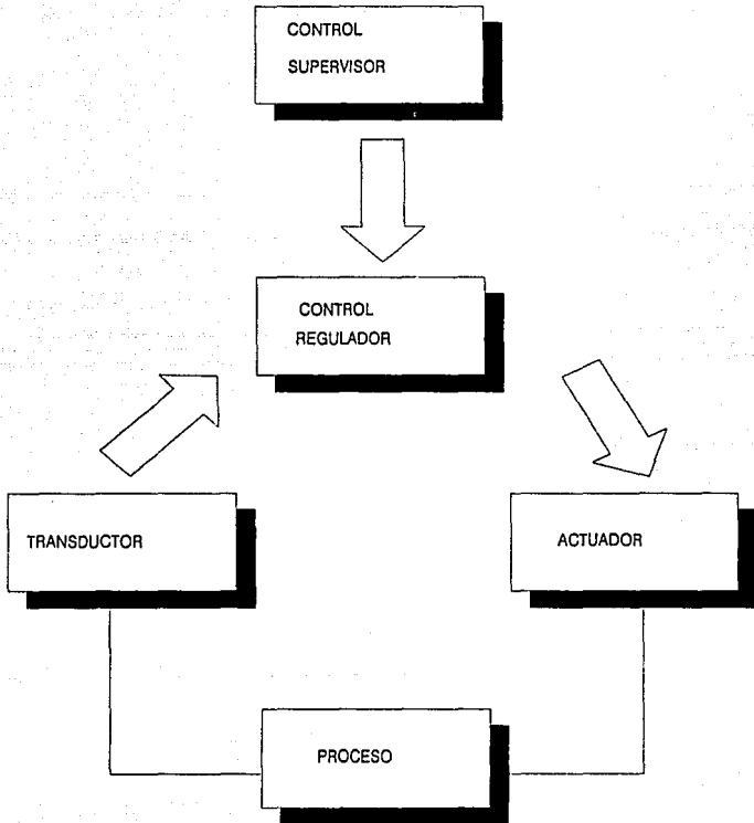
Fig. III.10 Sistemas de Control de un Proceso.
