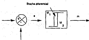
Fig. III.4b Diagrama de un Control con Brecha Diferencial.
