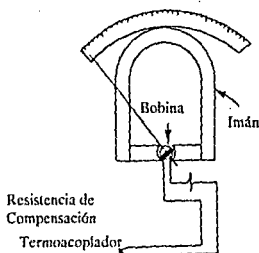
Fig. IV.18 Pirómetro
