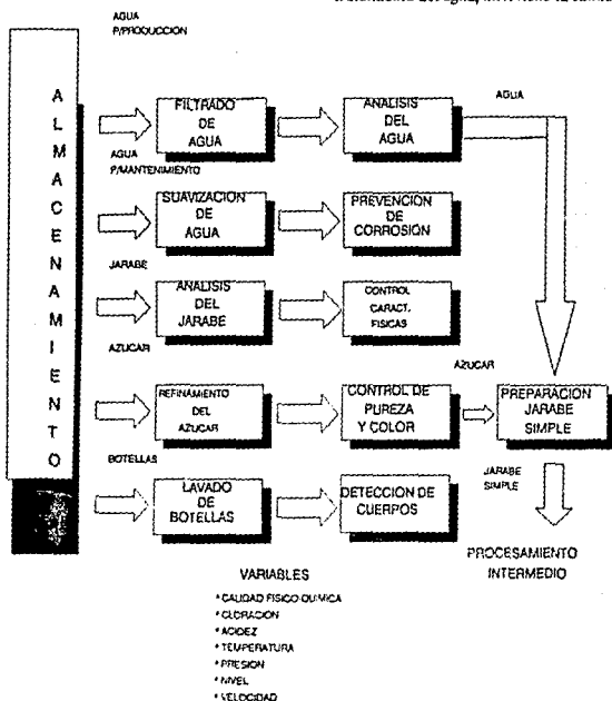
Fig. II.2 Variables en el Procesamiento Inicial
