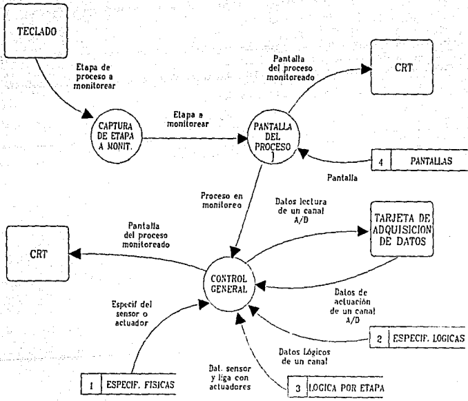
Fig. VI.10 Monitoreo de una Etapa de un Proceso a Controlar.
