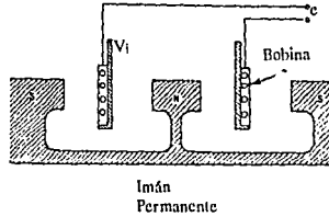
Fig. IV.12 Transductor de velocidad con bobina móvil
