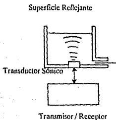
Fig. IV.36 Medidor Ultrasónico
