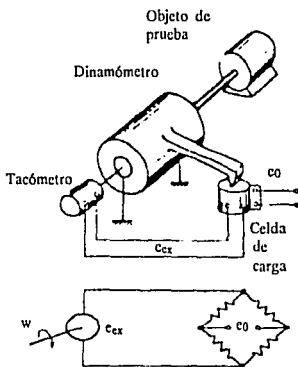
Fig. IV.25 Medición Instantánea de Poder
