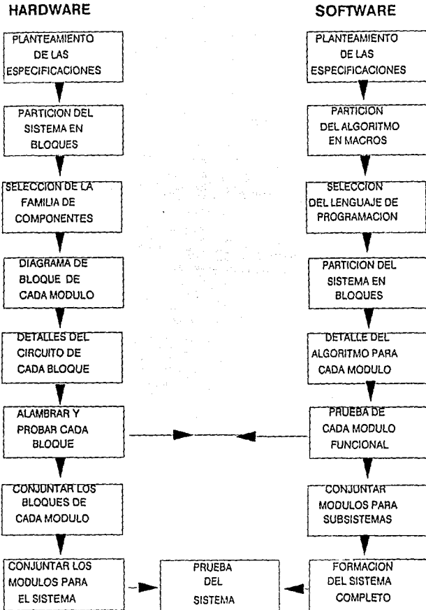
Fig. VI.4 Técnica de Diseño TOP-DOWN.
