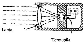
Fig. IV.17 Unidad de Radiación
