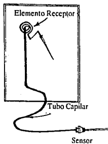
Fig. IV.19 Termómetro de Presión
