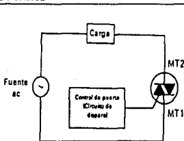
Fig. IV.47 Circuito con TRIAC
