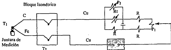
Fig. IV.14 Compensación por hardware
