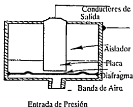
Fig. IV.29 Transductor de Presión Capacitivo
