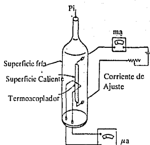
Fig. IV.34 Medidor de Vacío Termocoplado
