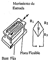
Fig. IV.3 Medidor de Tensión
