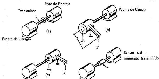
Fig. IV.24 Medición de Momentos de Máquinas Rotatorias
