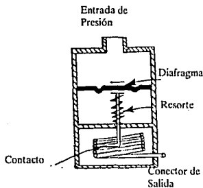
Fig. IV.27 Transductor de Presión Resistivo
