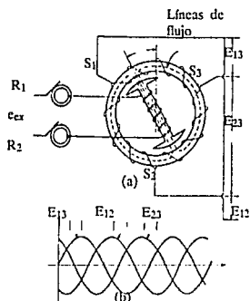
Fig. IV.6 Ejemplo de la familia de Synchros
