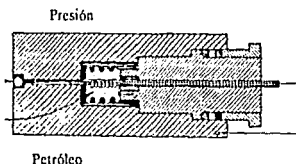
Fig. IV.31 Transductor de Alta Presión
