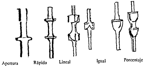
Fig. IV.41 Distintos tipos de tapones de válvulas
