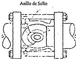
Fig. IV.42 Válvula de Bola
