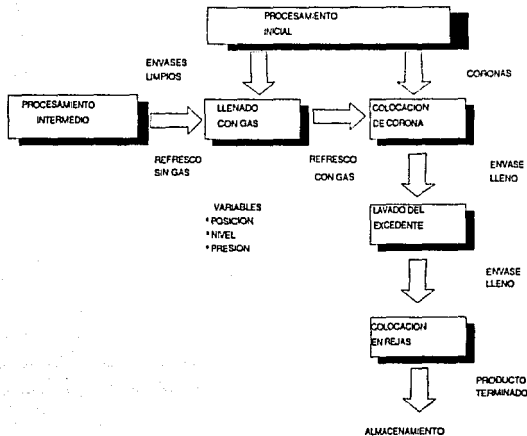
Fig. II.4 Variables en la etapa de Procesamiento Final
