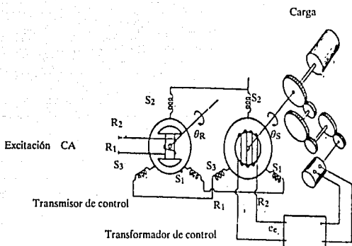
Fig. IV.6 Ejemplo de la familia de Synchros
