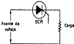
Fig. IV.45 Relación circuital del SCR y la carga
