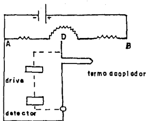
Fig. IV.20 Circuito Fundamental de un Potenciómetro
