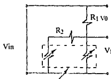
Fig. IV.16 Respuesta de un termistor y linealizador
