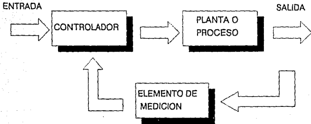
Fig. III.2 Sistema de control de lazo cerrado.
