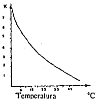
Fig. IV.16 Respuesta de un termistor y linealizador
