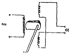
Fig. IV.4 Transformador Diferencial Rotacional
