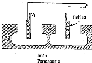
Fig. IV.12 Transductor de velocidad con bobina móvil
