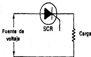
Fig. IV.45 Relación circuital del SCR y la carga
