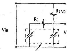
Fig. IV.16 Respuesta de un termistor y linealizador
