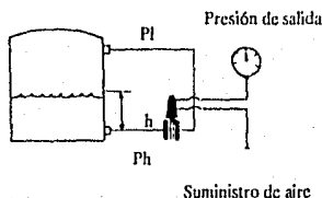
Fig. IV.39 Medidor de Presión Diferencial
