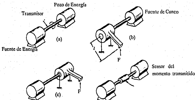
Fig. IV.24 Medición de Momentos de Máquinas Rotatorias
