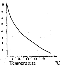
Fig. IV.16 Respuesta de un termistor y linealizador
