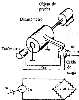
Fig. IV.25 Medición Instantánea de Poder
