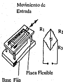
Fig. IV.3 Medidor de Tensión
