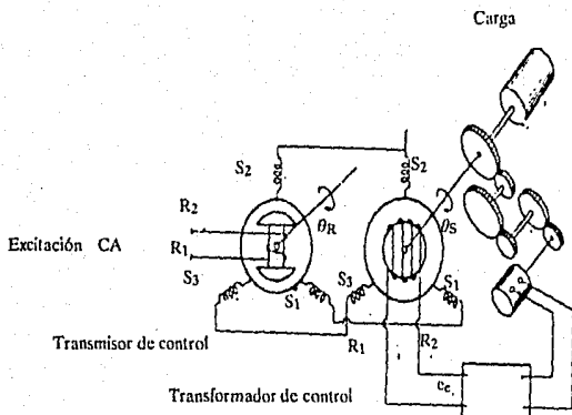
Fig. IV.6 Ejemplo de la familia de Synchros
