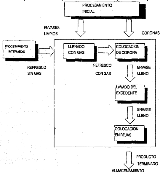
Fig. I.10 Procesamiento Final
