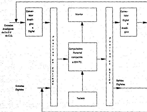
Fig. VI.2 Diagrama de Bloques General del Simulador.
