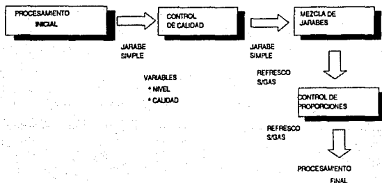
Fig. II.3 Variables en la etapa de Procesamiento Intermedio
