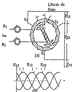
Fig. IV.6 Ejemplo de la familia de Synchros
