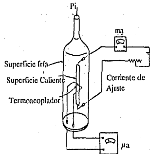
Fig. IV.34 Medidor de Vacío Termocoplado
