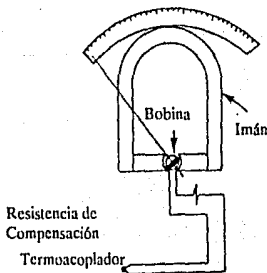
Fig. IV.18 Pirómetro
