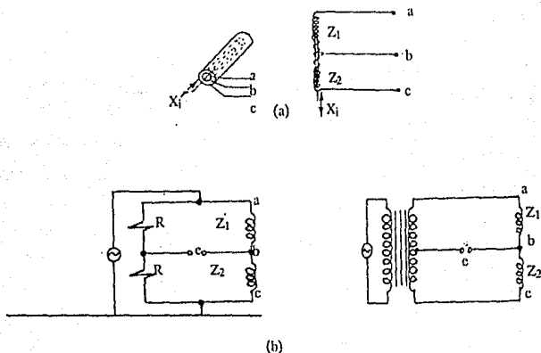
Fig. IV.8 Transductor de Inductancia Variable
