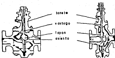
Fig. IV.40 Válvulas de Globo de puerto sencillo y doble
