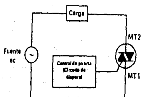
Fig. IV.47 Circuito con TRIAC
