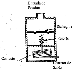
Fig. IV.27 Transductor de Presión Resistivo
