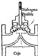
Fig. IV.43 Válvula de Diafragma
