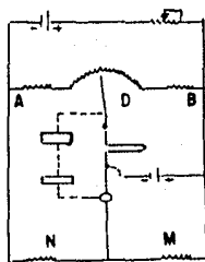
Fig. IV.22 Potenciómetro con compensación de juntura fría
