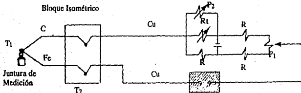
Fig. IV.14 Compensación por hardware
