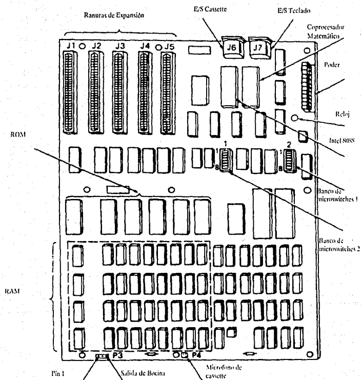
Fig. A.1 Componentes de la tarjeta del sistema
