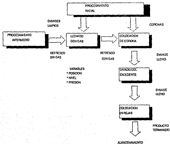
Fig. II.4 Variables en la etapa de Procesamiento Final
