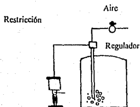
Fig. IV.38 Medidor de Burbujeo
