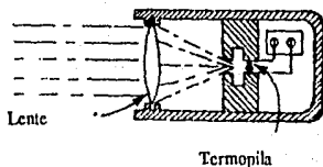
Fig. IV.17 Unidad de Radiación
