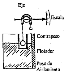
Fig. IV.37 Desplazador
