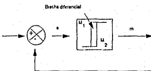
Fig. III.4b Diagrama de un Control con Brecha Diferencial.
