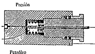
Fig. IV.31 Transductor de Alta Presión
