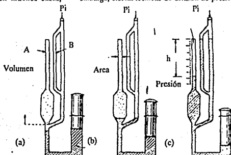
Fig. IV.32 Medidor de McLeod
