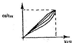
Fig. IV.2 Potenciómetro Resistivo y su efecto de carga
