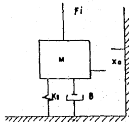
Fig. IV.23 Transductor de Fuerza Elástica
