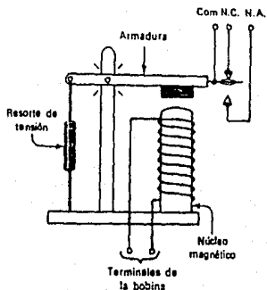
Fig. IV.48 Partes esenciales de un relevador
