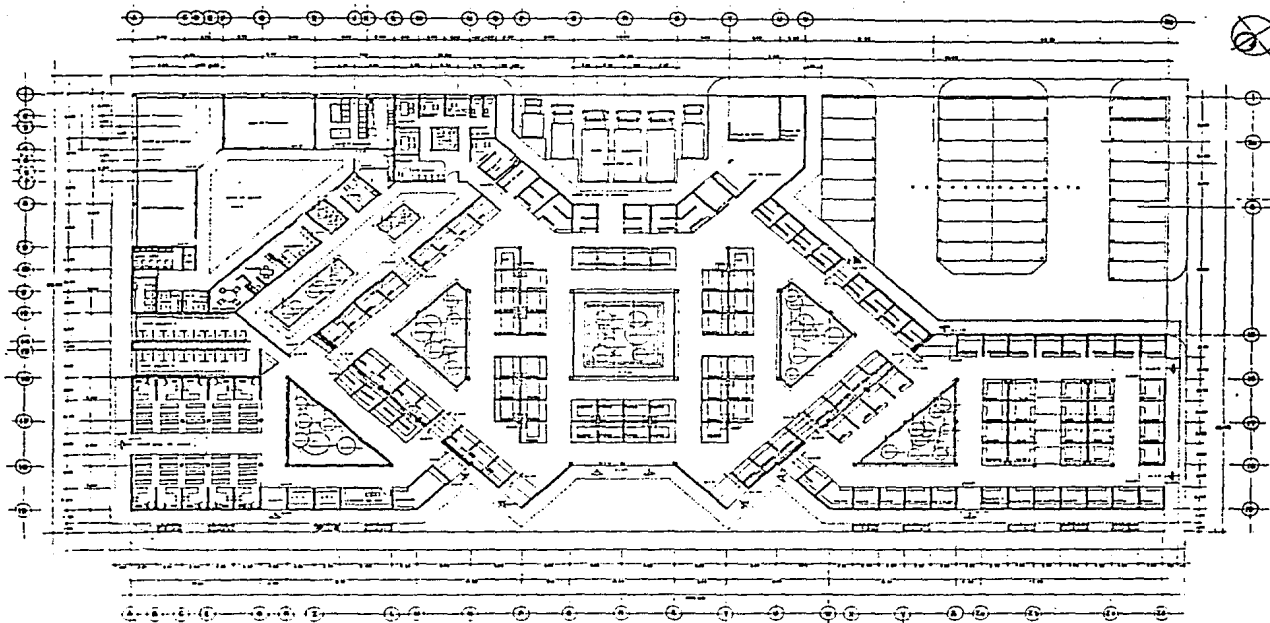
PLANTA ARQUITECTÓNICA DE CONJUNTO
