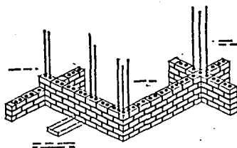
METALLES DE ARMADO DE TABIQUE EMBALTAZO
