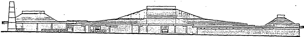
FACHADA SURESTE
