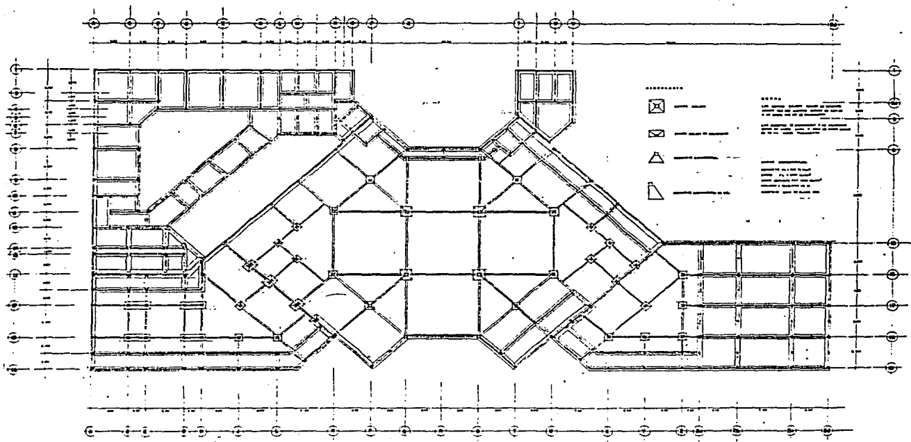
PLANTA DE CIMENTACION DE CONJUNTO
