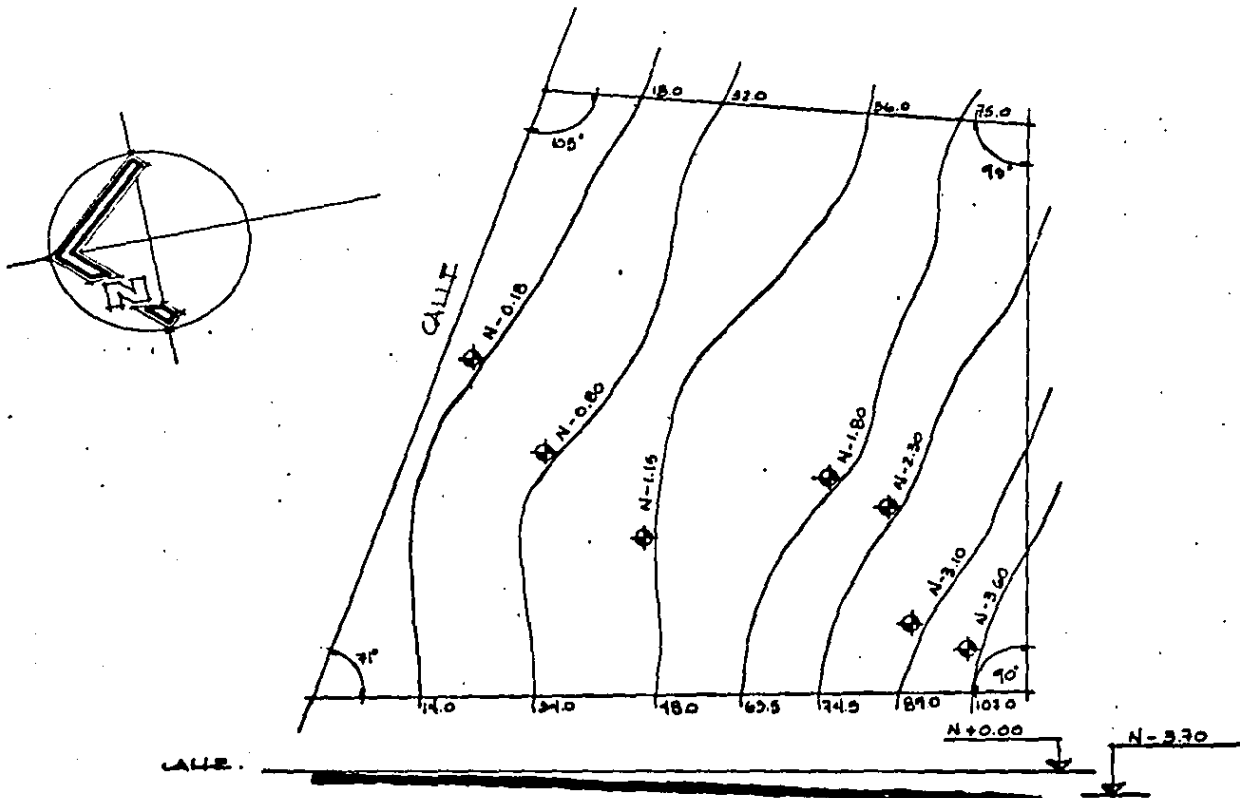
TOPOGRAFIA Y PERFIL DEL TERRENO
