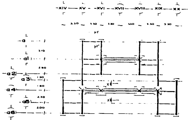
PLANTA DE CIMENTACION Escala 1:100
