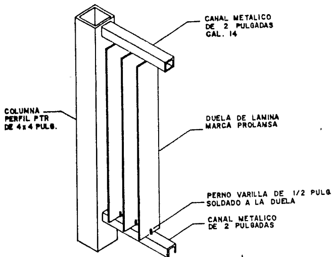
DETALLE 6
