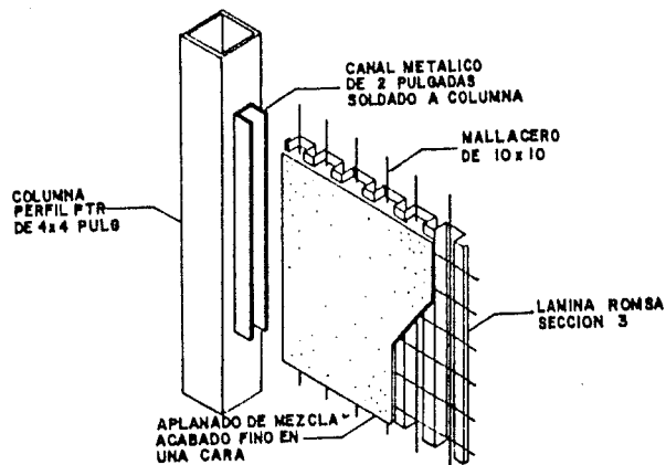
DETALLE 7
