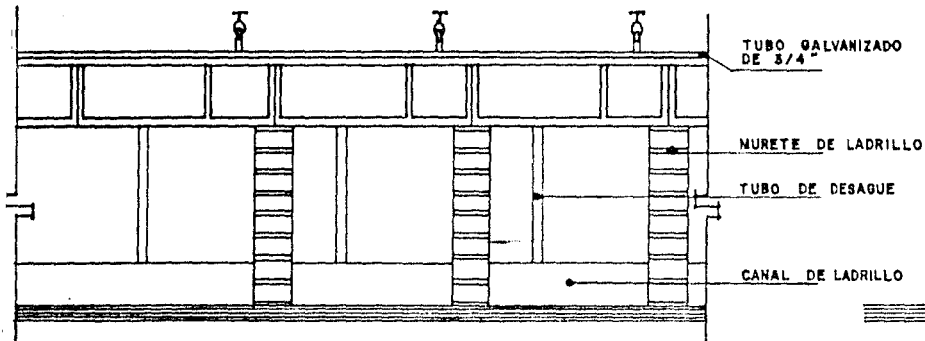
ALZADO
