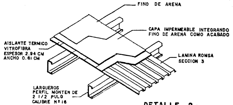
DETALLE 2
