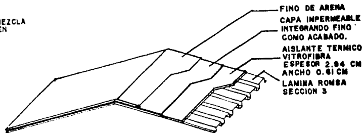
DETALLE 9
