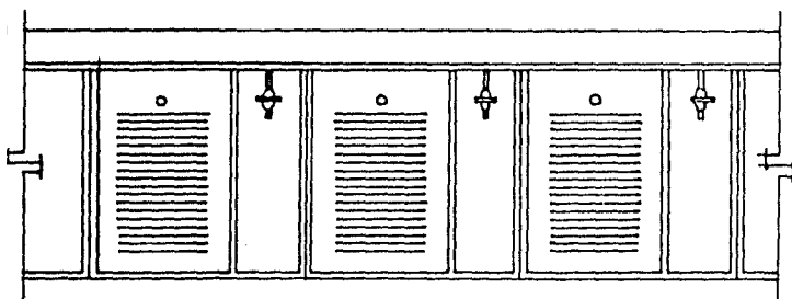
PLANTA
