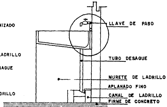
CORTE
